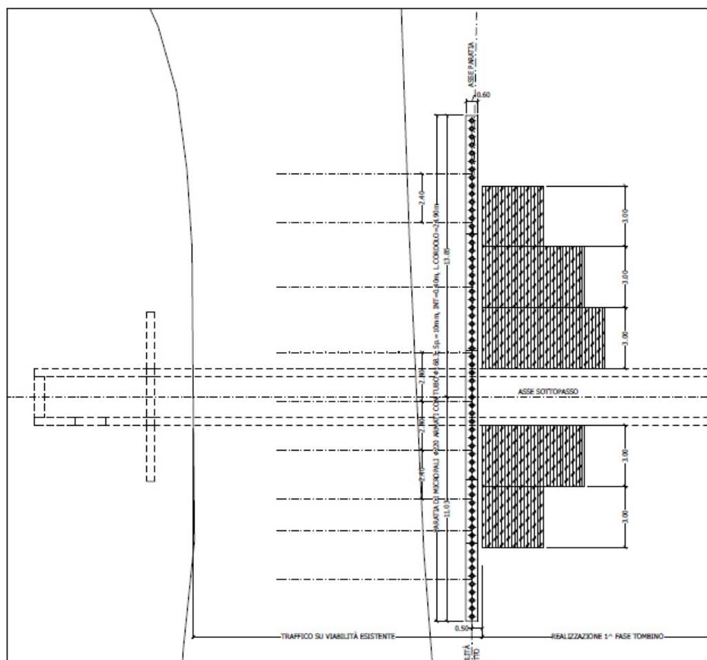
Figura 1-1: Pianta
