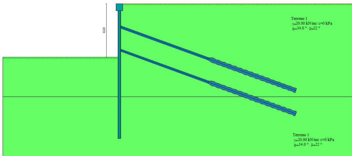
Figura 3-1: Geometria della paratia
