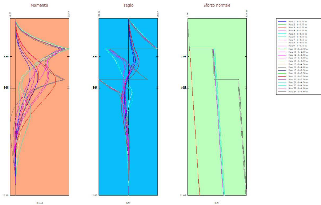
Figura 6-1: Involuppo sollecitazioni paratia
