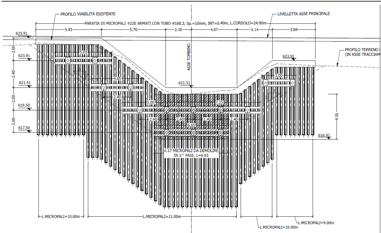
Figura 1-2: Prospetto
