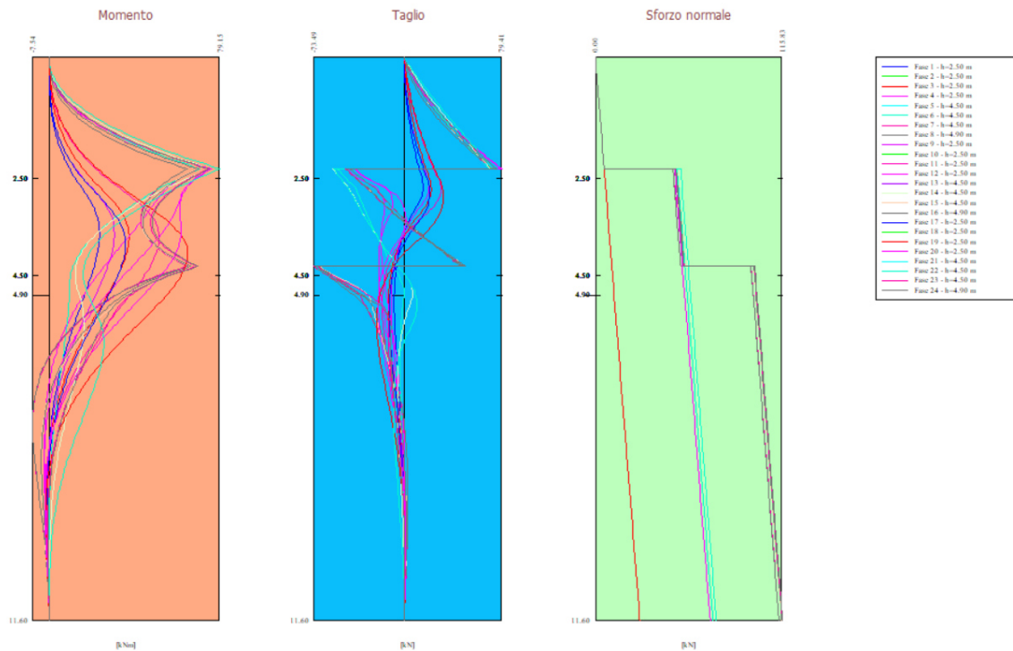
Figura 6-1: Involuppo sollecitazioni paratia
