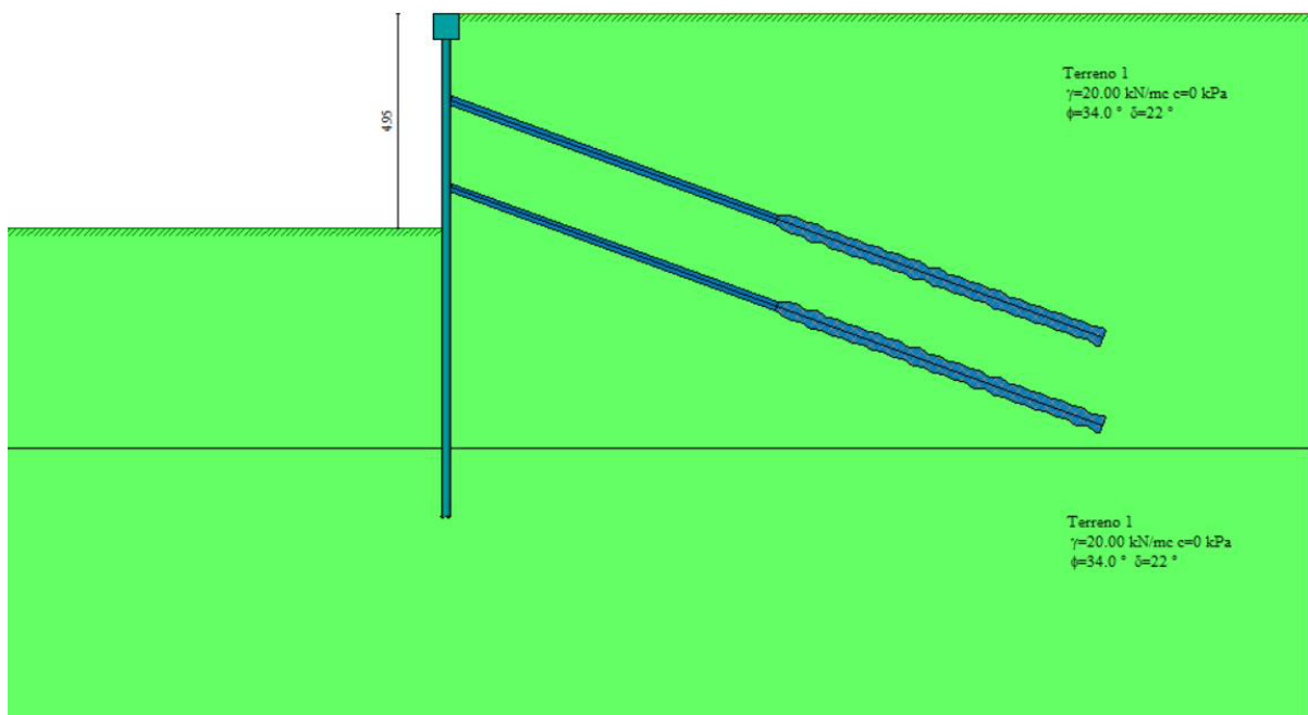
Figura 3-1: Geometria della paratia
