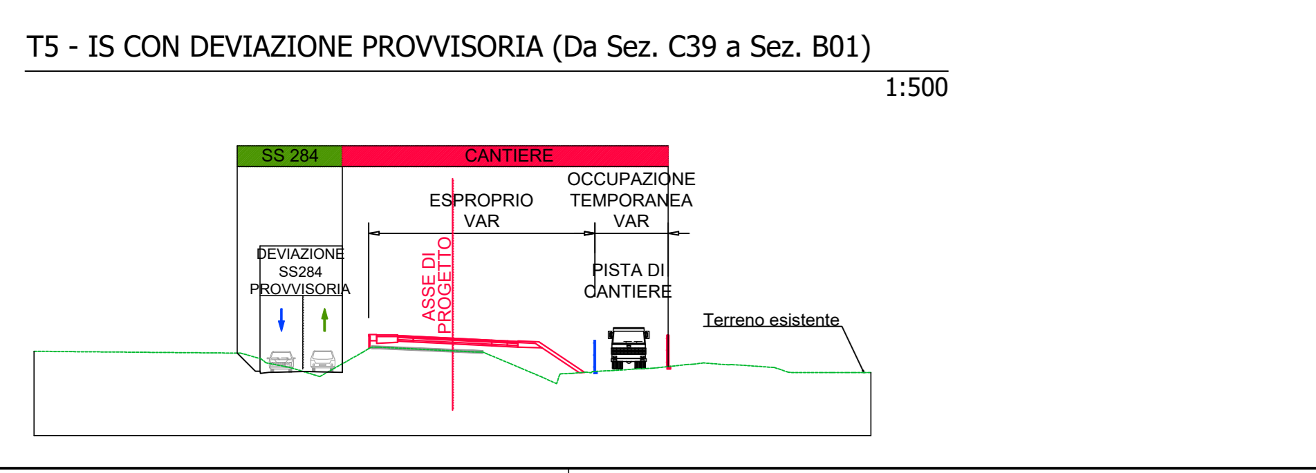
SEZIONI TRASVERSALI DI CANTIERIZZAZIONE TIPOLOGICHE DEL SUB CANTIERE DI APPARTENENZA
