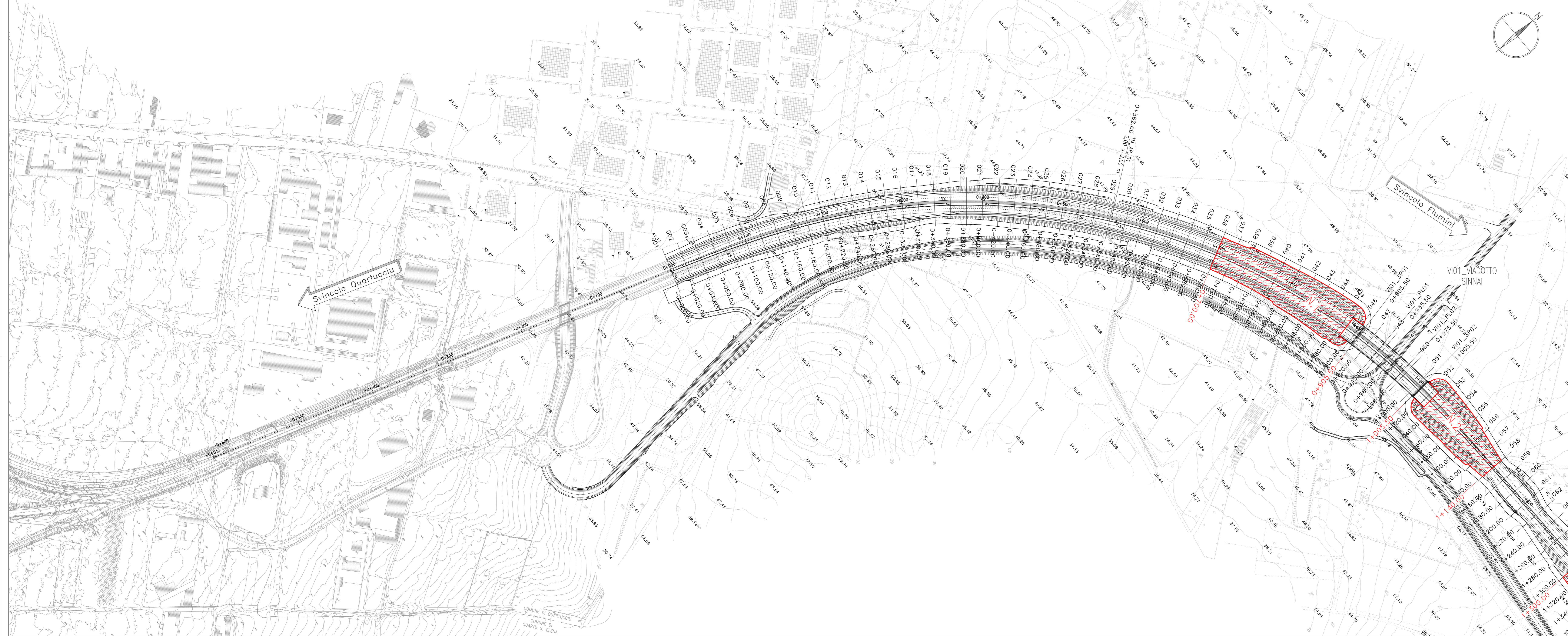
PLANIMETRIA DA prog. 0+860,00 a prog. 2+700,00
