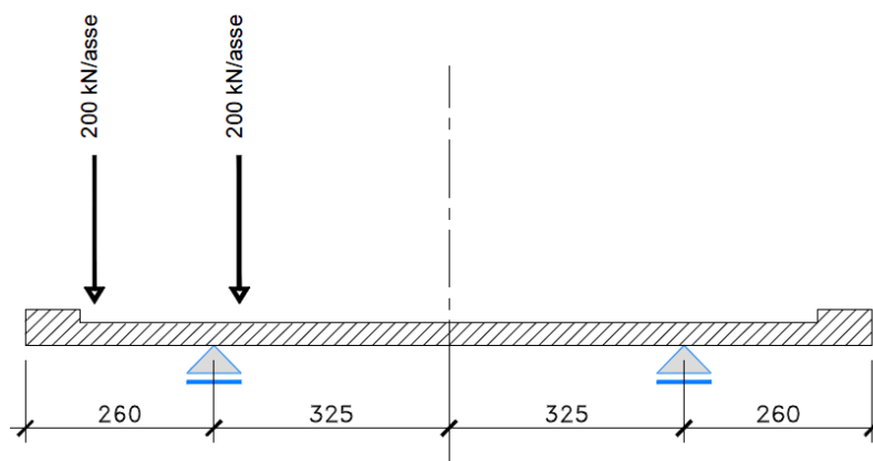
Figura 6.15. Disposizione trasversale dei carichi mobili – Configurazione E
