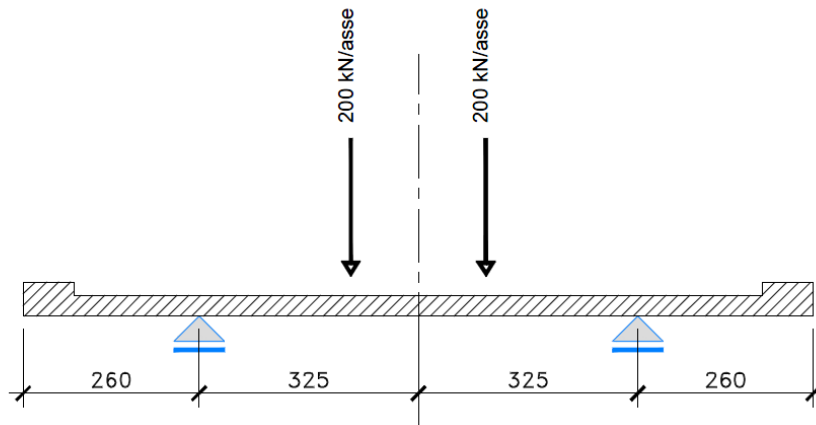
Figura 6.14. Disposizione trasversale dei carichi mobili – Configurazione D
