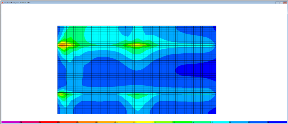
Figura 6.25. Combinazione ENVESLER – M11 min
