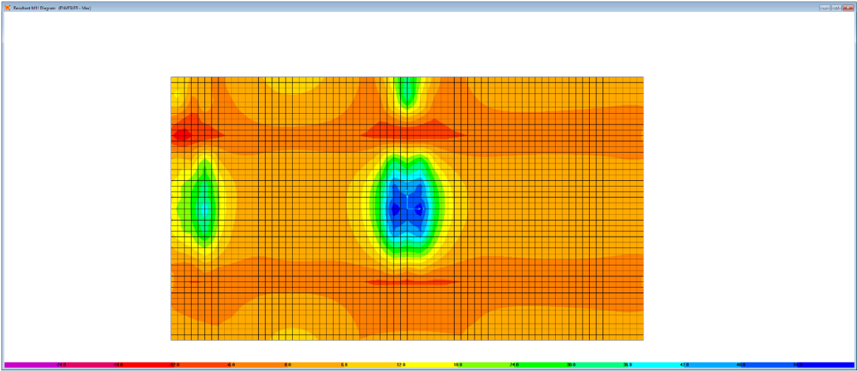
Figura 6.24. Combinazione ENVESLER – M11 max
