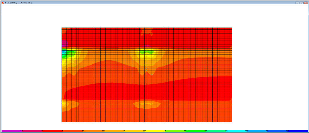
Figura 6.20. Combinazione ENVELSU – V23 max
