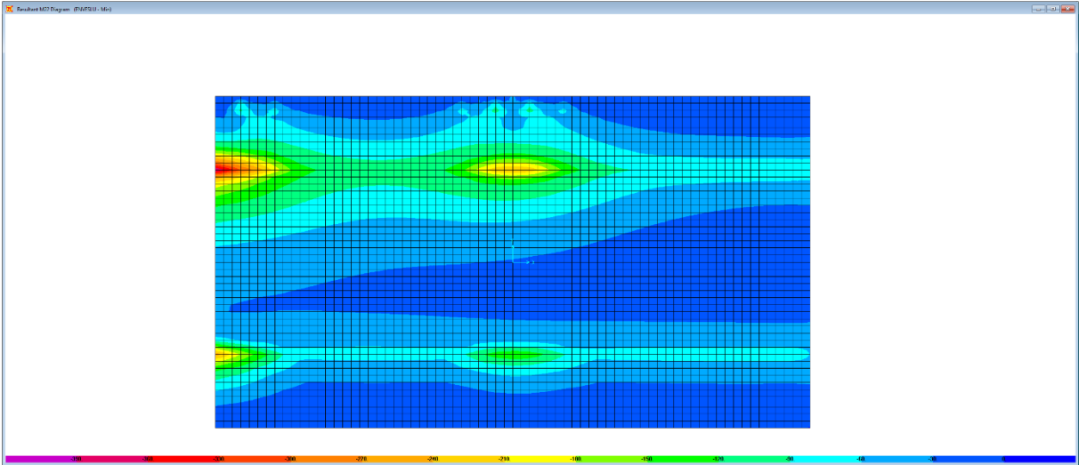
Figura 6.17. Combinazione ENVESLU – M22 min
