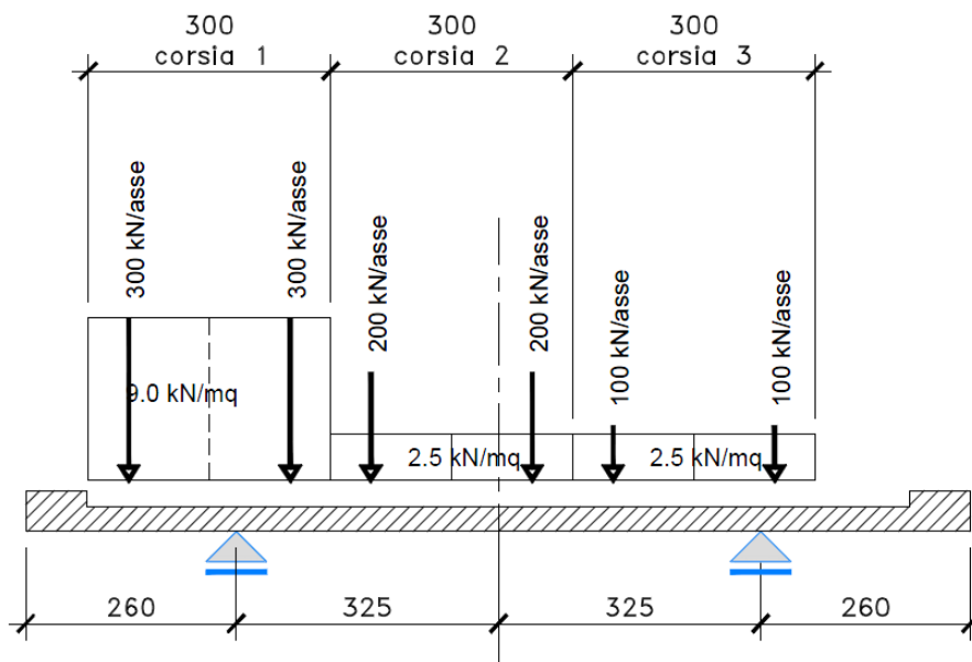
Figura 6.11. Disposizione trasversale dei carichi mobili – Configurazione A
