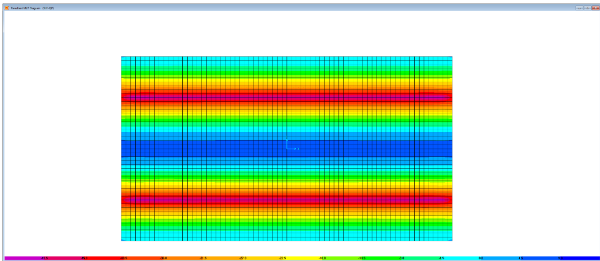
Figura 6.30. Combinazione SLE-QP – M22
