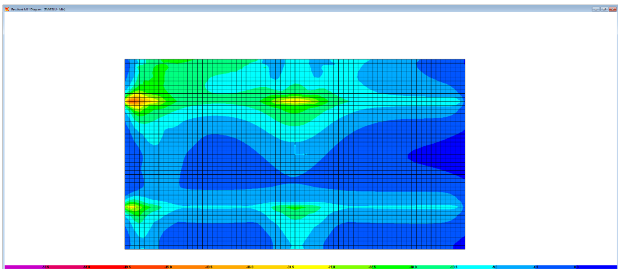
Figura 6.19. Combinazione ENVELSU – M11 min
