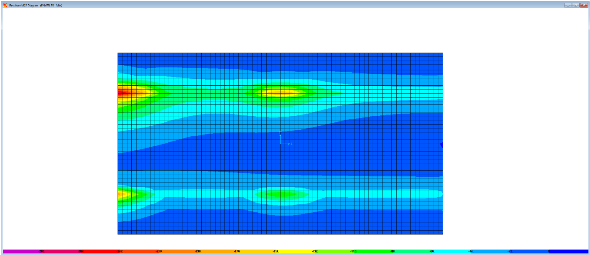
Figura 6.23. Combinazione ENVESLER – M22 min
