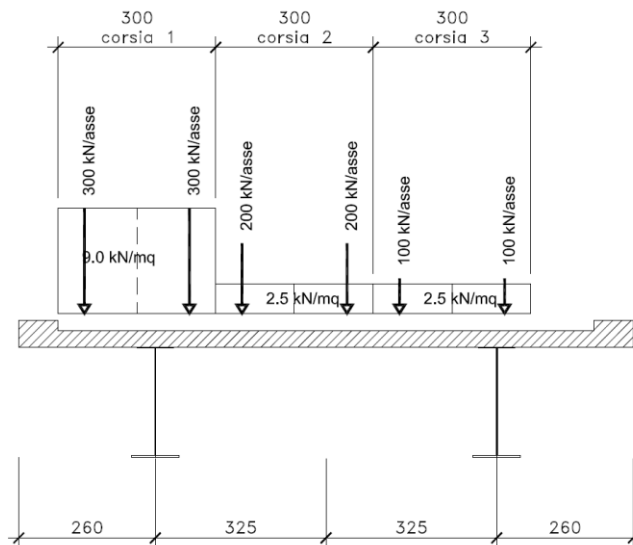
Figura 5.1. Disposizione trasversale carichi mobili per analisi globale travi principali impalcato
