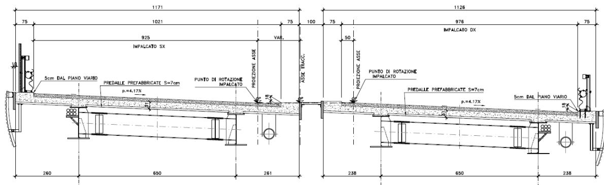
Figura 1.1. Sezione trasversale impalcato in campata
