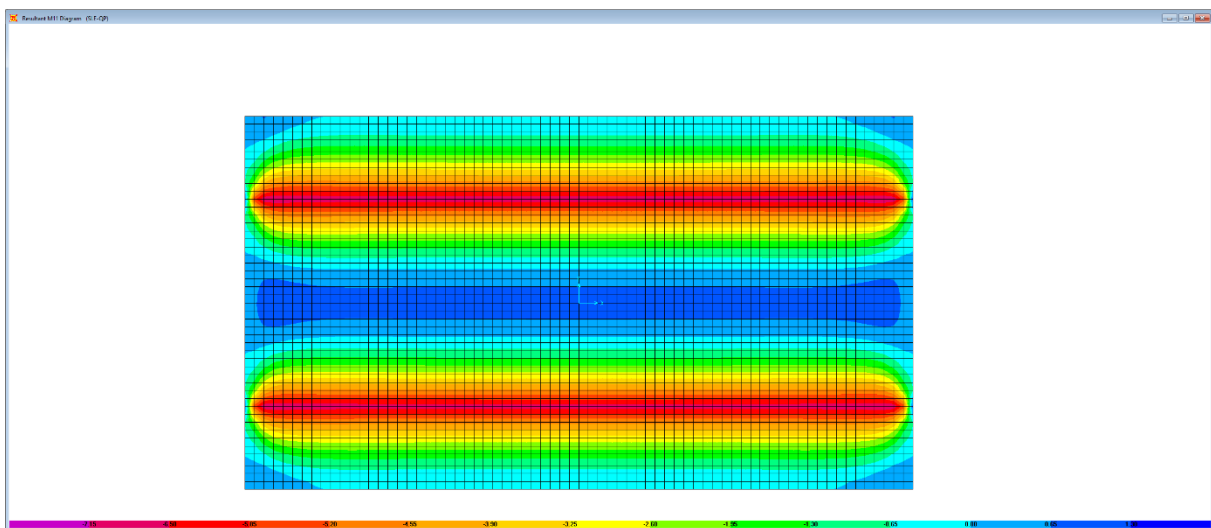
Figura 6.31. Combinazione SLE-QP – M11
