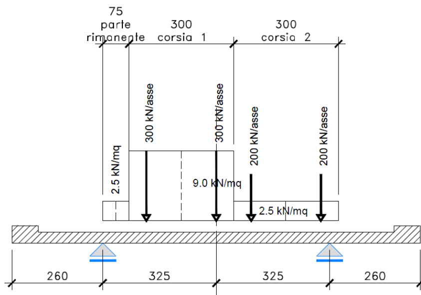
Figura 6.13. Disposizione trasversale dei carichi mobili – Configurazione C
