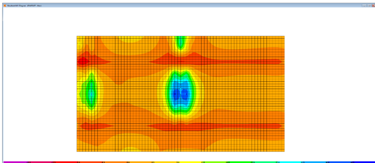
Figura 6.28. Combinazione ENVSLEF – M11 max
