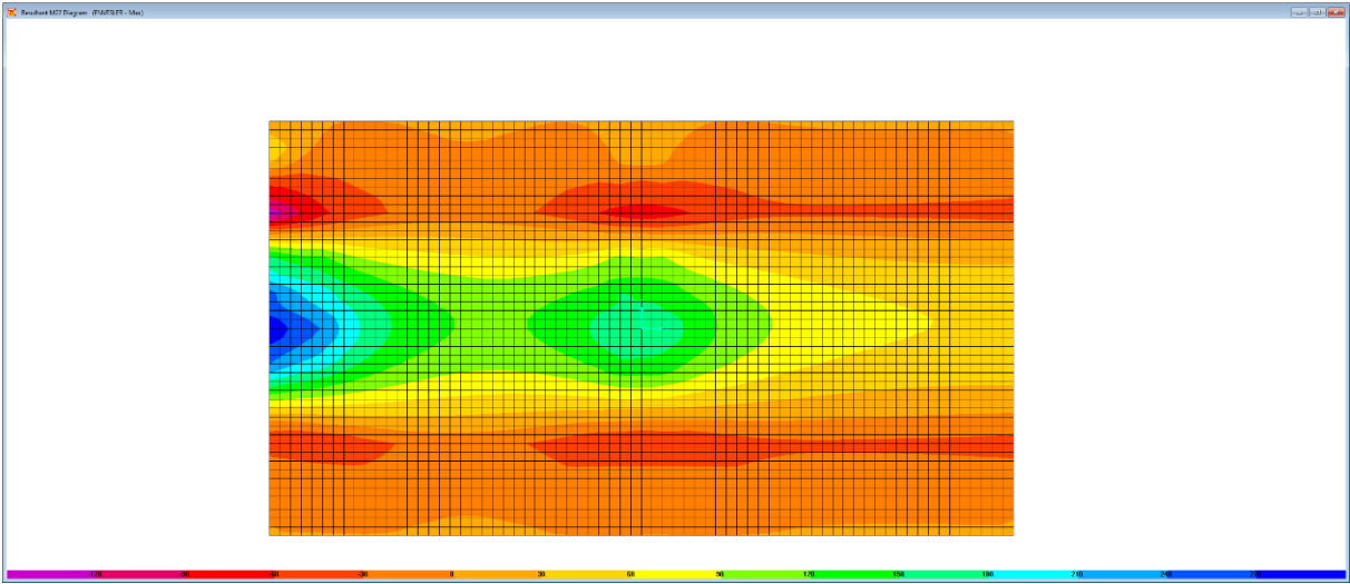
Figura 6.22. Combinazione ENVESLER – M22 max
