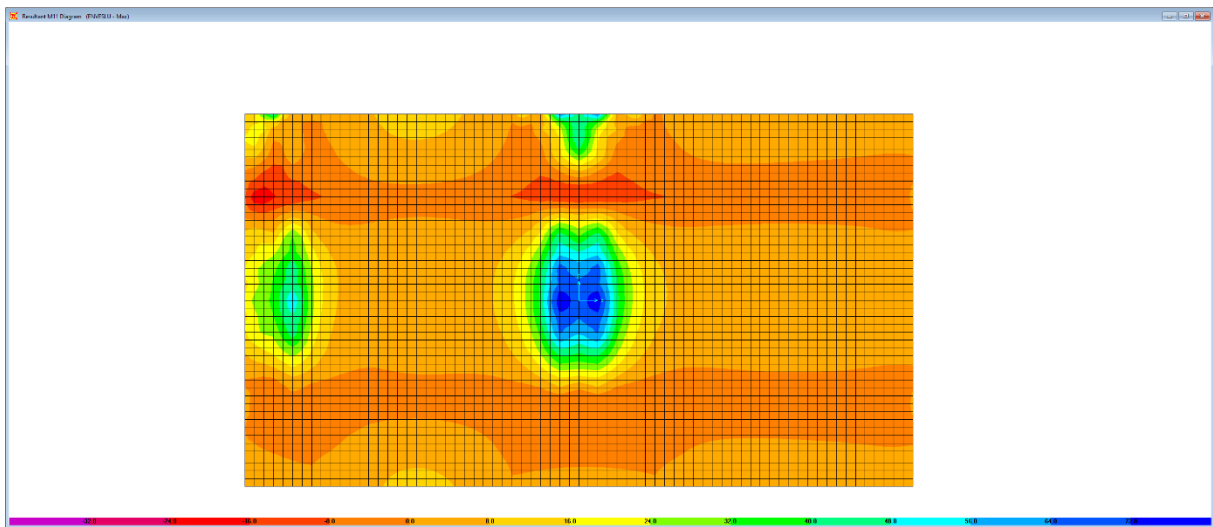
Figura 6.18. Combinazione ENVELSU – M11 max
