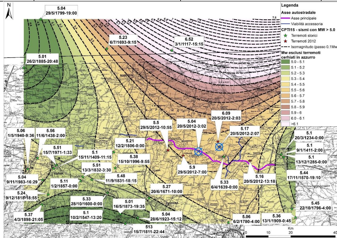
Epicentri, magnitudo e linee di iso-magnitudo – CPT115/DBM15. Sono stati esclusi dall'analisi i sismi del 2012 cerchiati in azzurro (repliche). In linea magenta il tracciato autostradale di progetto 2012.
