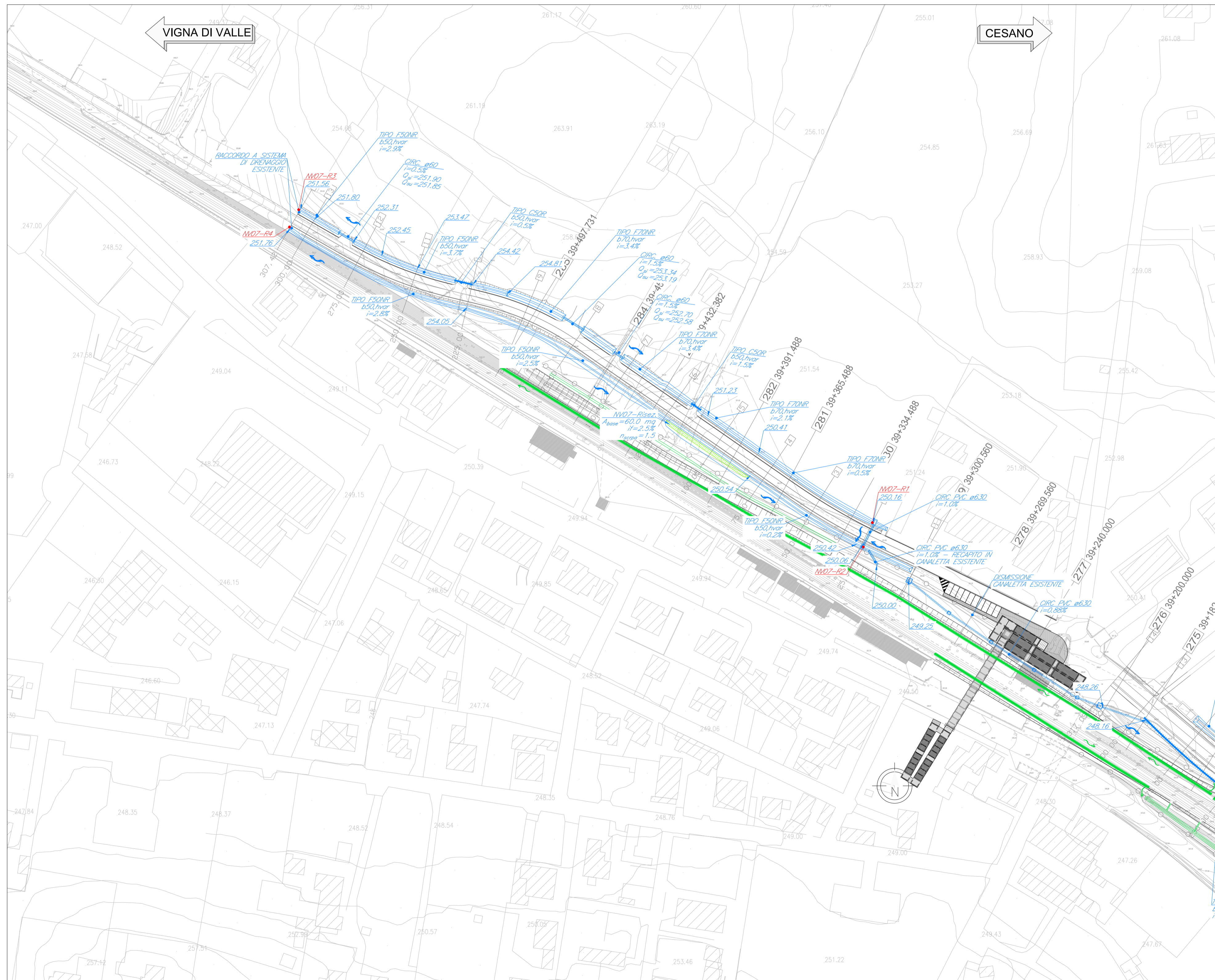
PLANIMETRIA DI PROGETTO SCALA 1:1000
