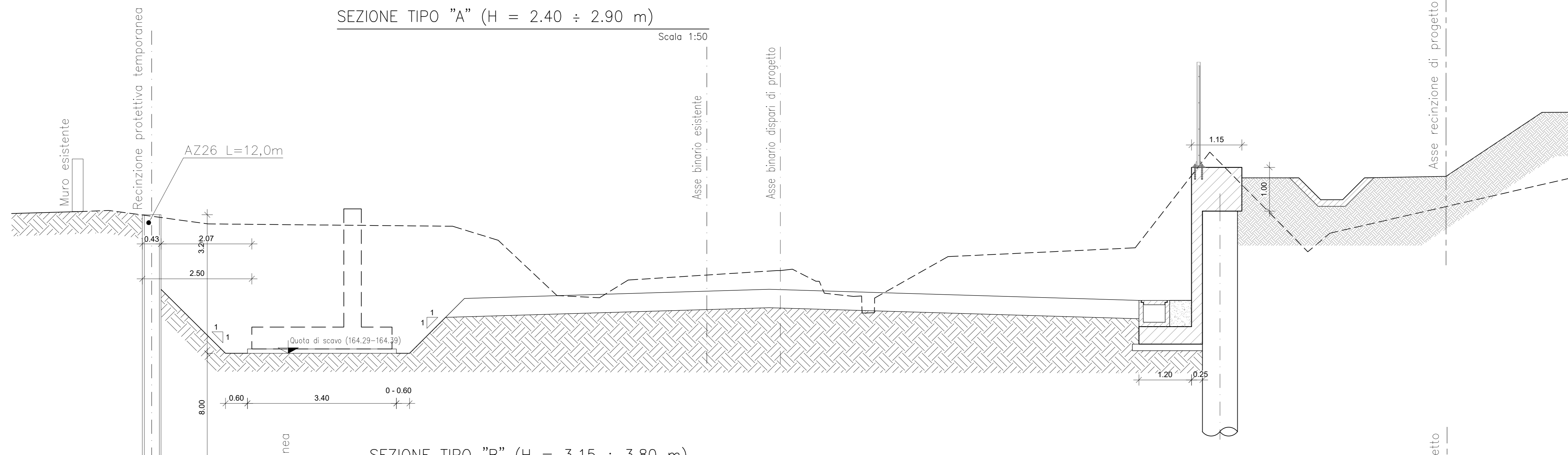
SEZIONE TIPO "B" (H = 3.15 ÷ 3.80 m)
