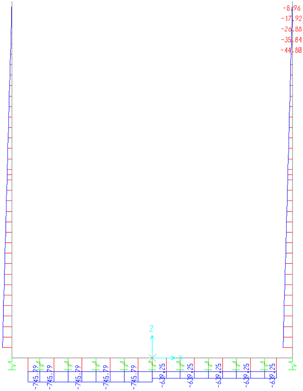
Fig. 3 – Involuppo azioni assiali SLU
