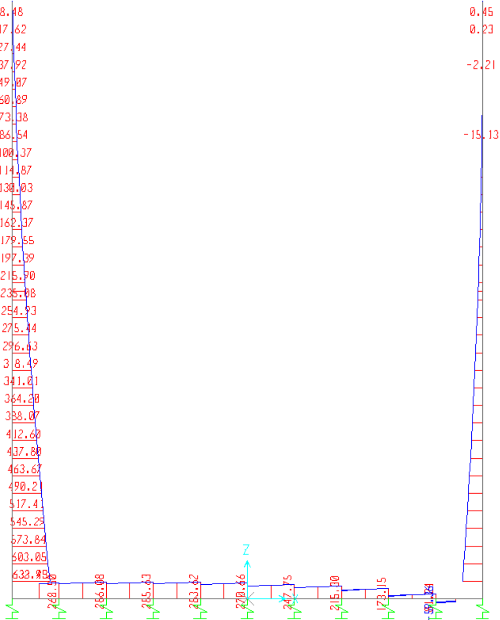
Fig. 5 – Involuppo sforzi taglianti SLV
