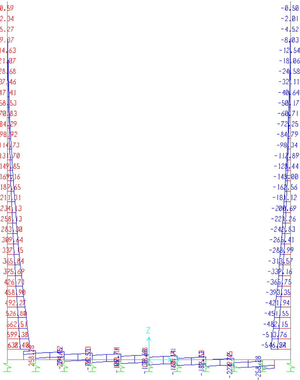
Fig. 2 – Involuppo sforzi taglianti SLU
