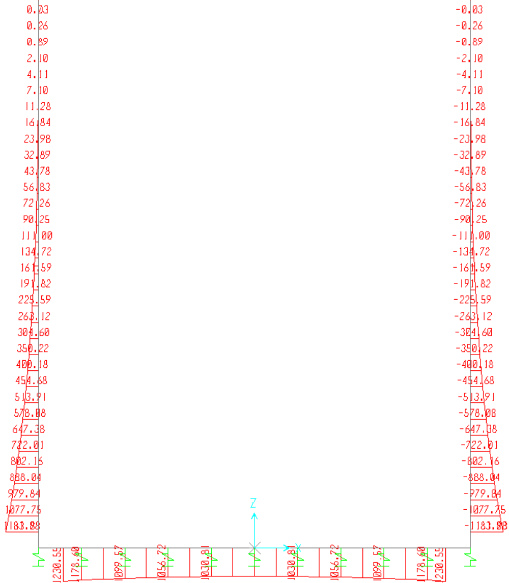
Fig. 7 – Involuppo momenti flettenti SLE rara
