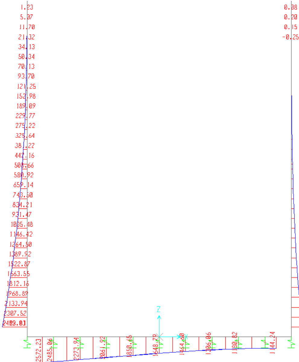
Fig. 4 –Involuppo momenti flettenti SLV
