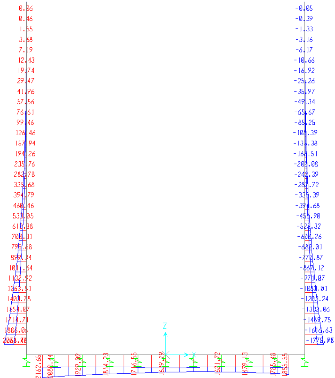
Fig. 1 – Involuppo momenti flettenti SLU
