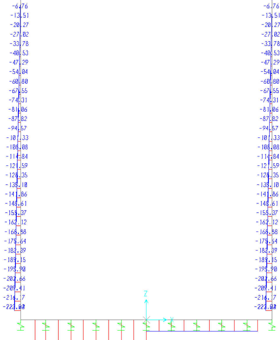
Fig. 6 – Inviluppo azioni assiali SLV
