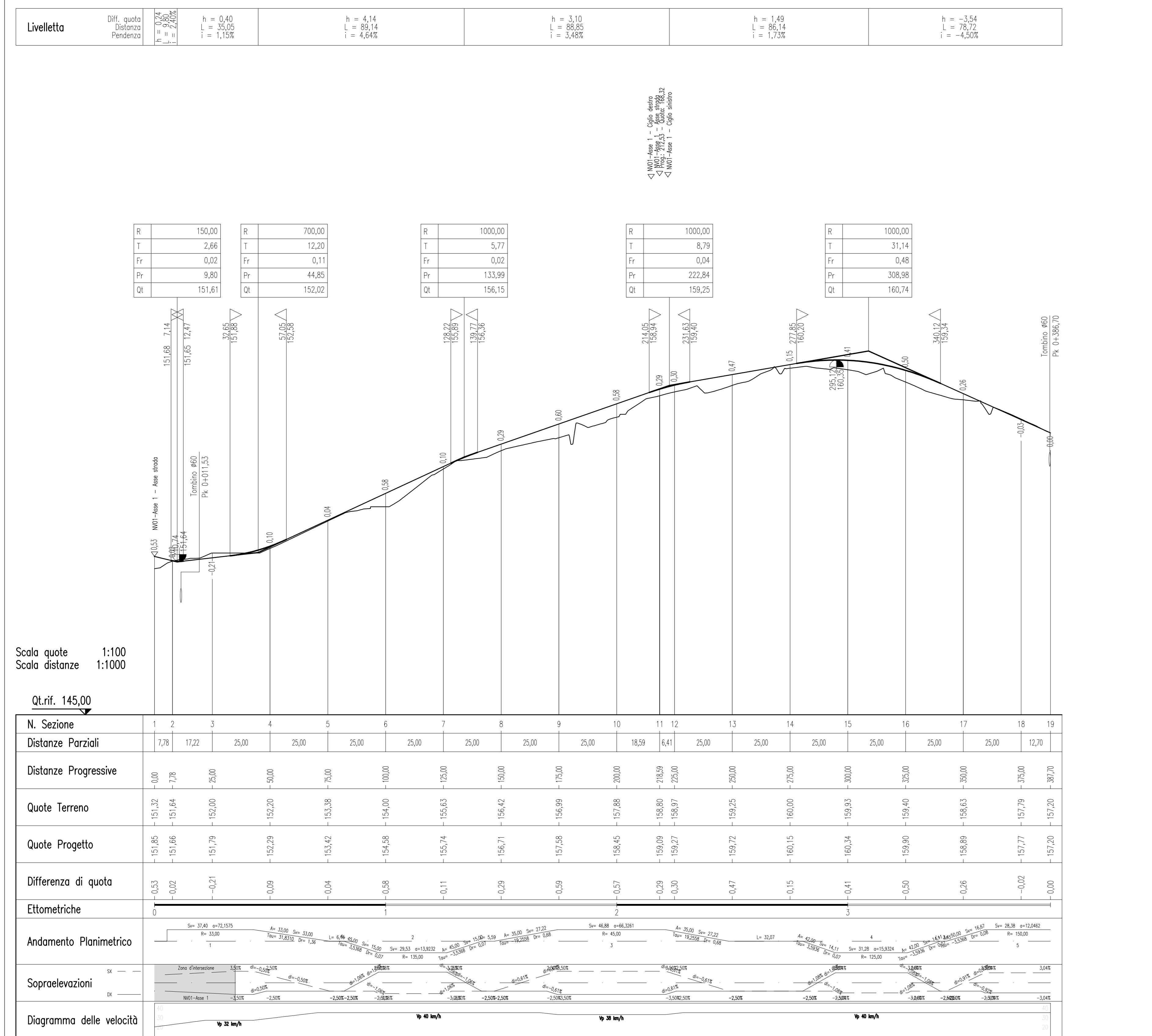
PROFILO LONGITUDINALE - Asse 2 - SCALA 1:1000/100
