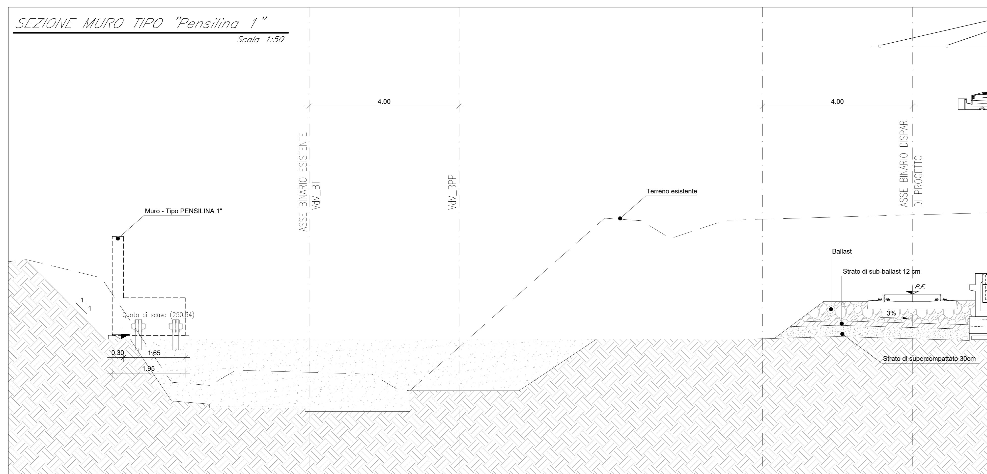
SEZIONE MURO TIPO "B" Scala 1:50
