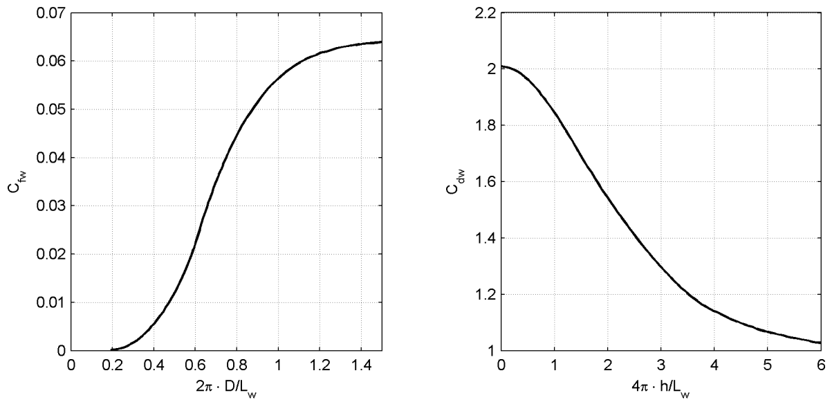
Figura 3-4. Valori dei coefficienti C_{fw} e C_{dw} per il calcolo della forza esercitata dal moto ondoso sulla nave (ROM 02-90).
