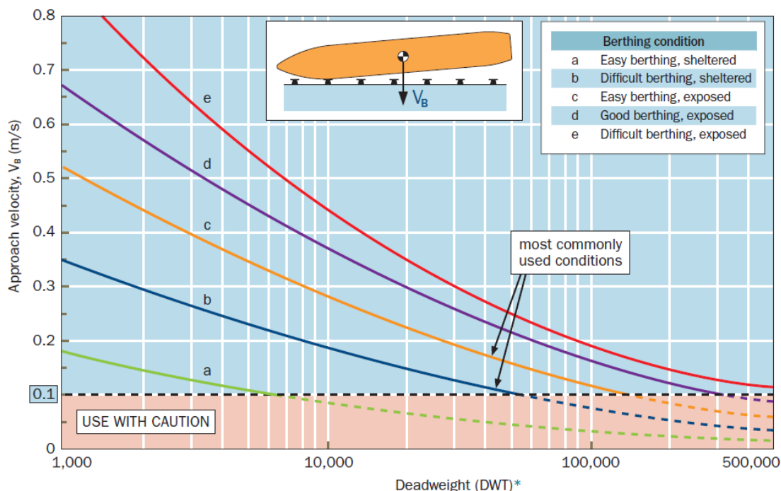
Figura 3-3. Velocità di accosto delle navi.
