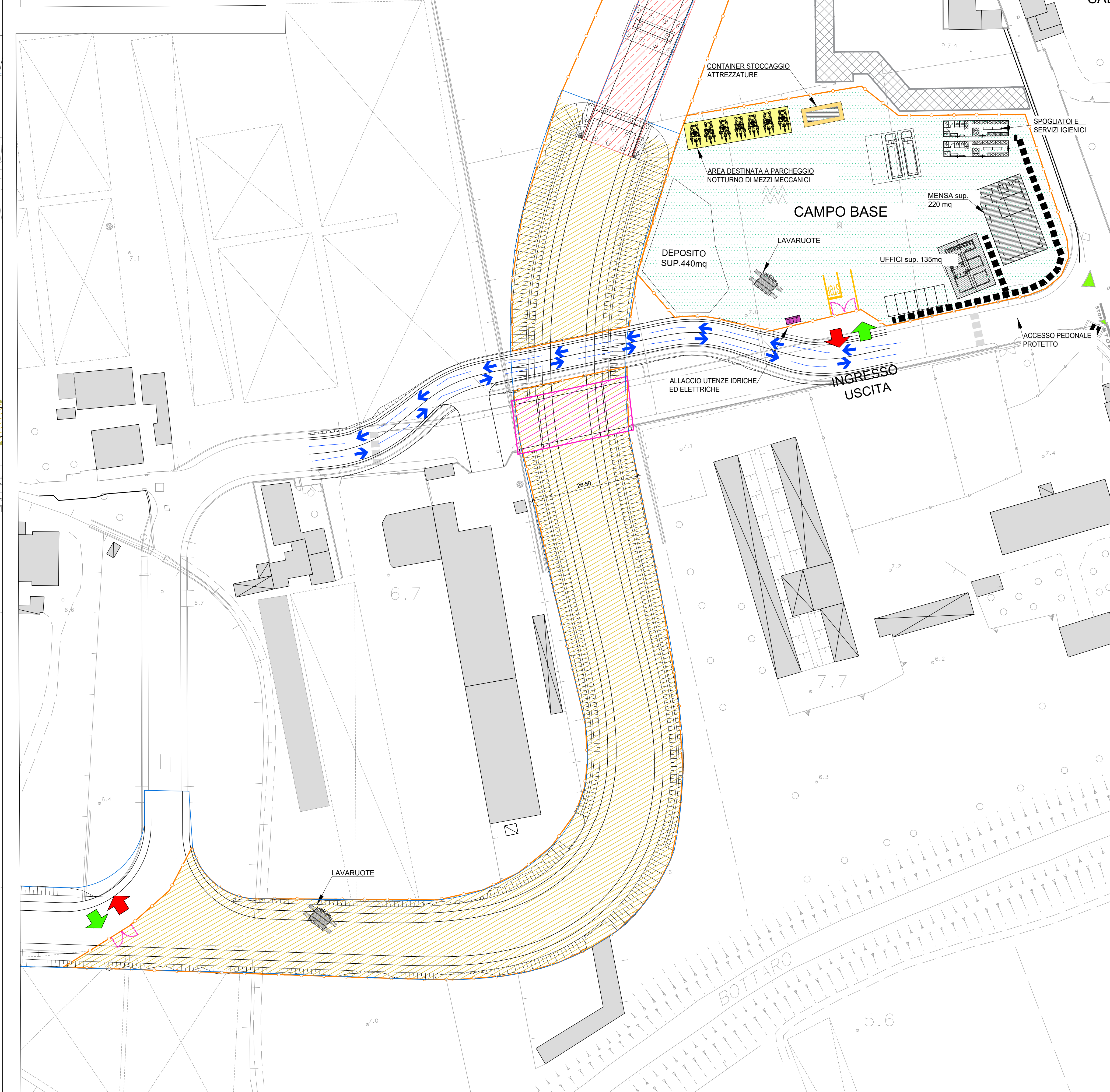
PLANIMETRIA DI CANTIERE - FASE 3 - VIABILITA' NORD scala 1:500
