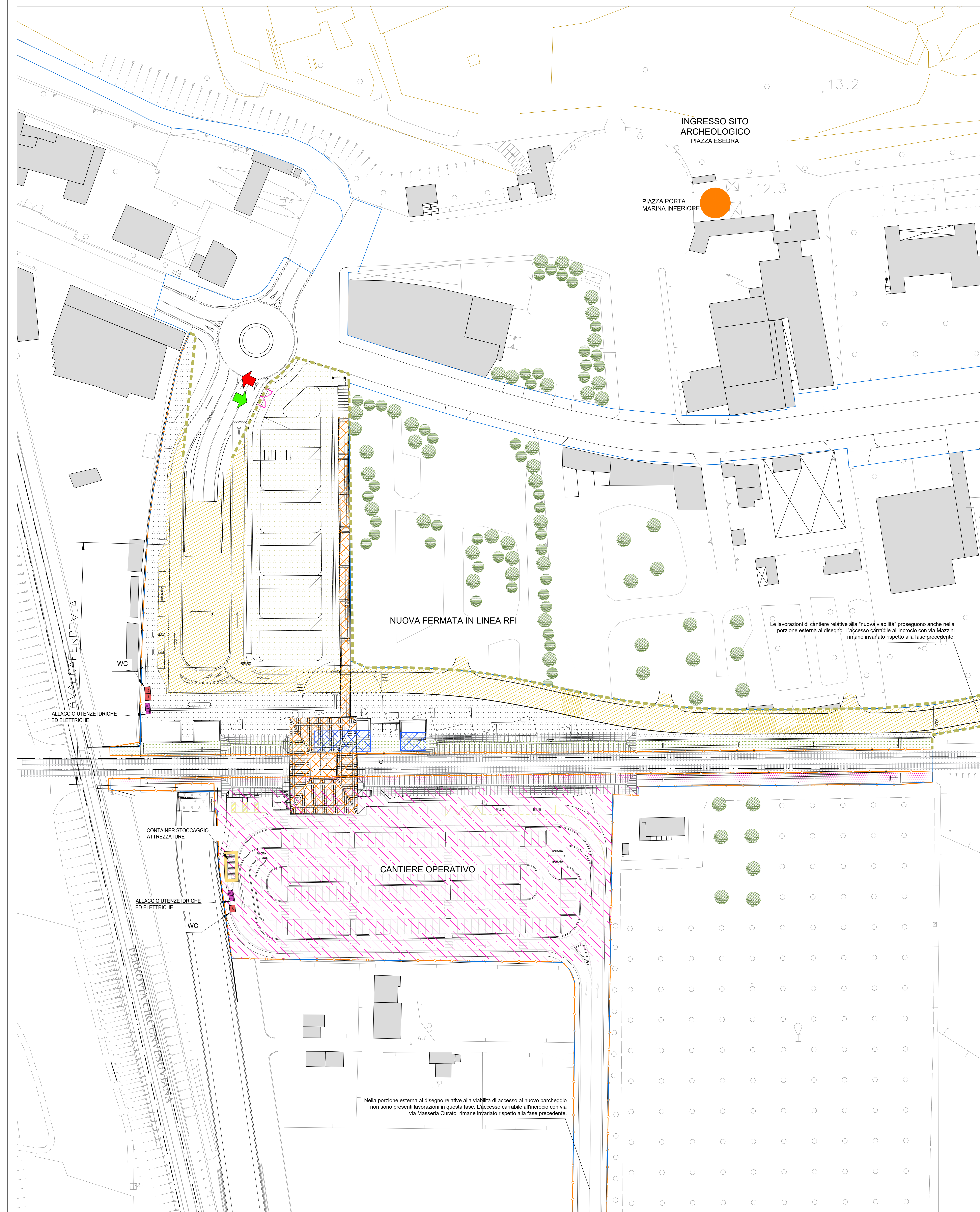
PLANIMETRIA DI CANTIERE - FASE 3 - LATO INGRESSO SCAVI PIAZZA ESEDRA scala 1:500
