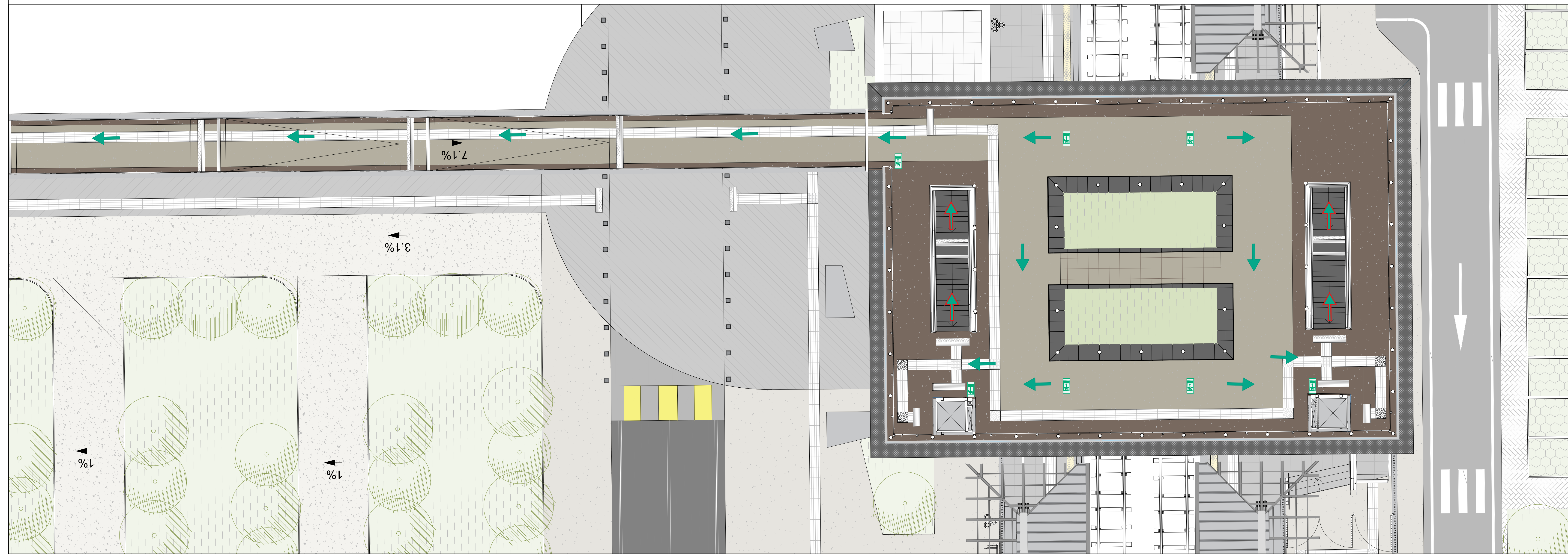
PLANIMETRIA QUOTA PERISTILIO - PASSERELLA scala 1:100
