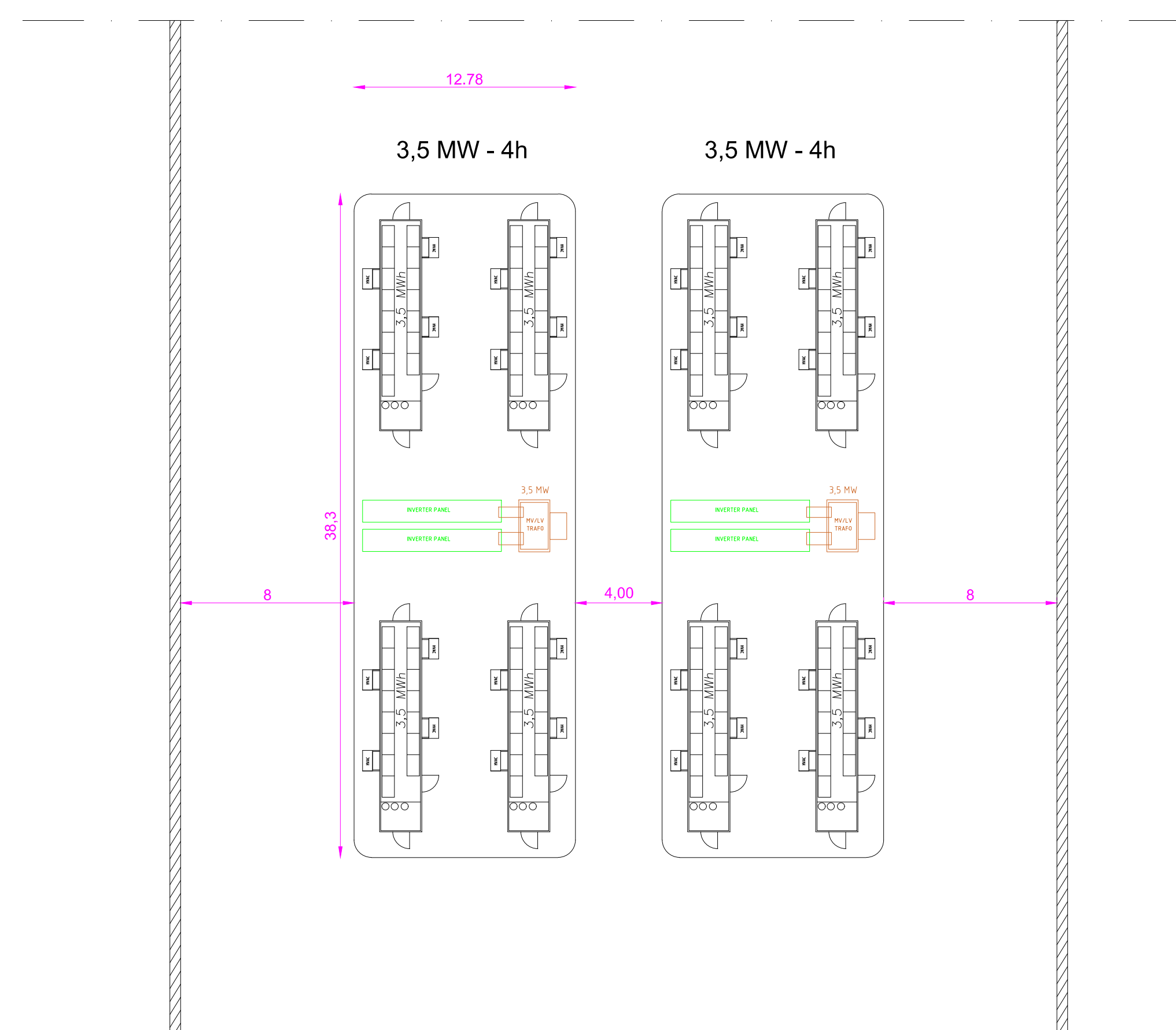
PARTICOLARE ACCUMULO SCALA 1:25
