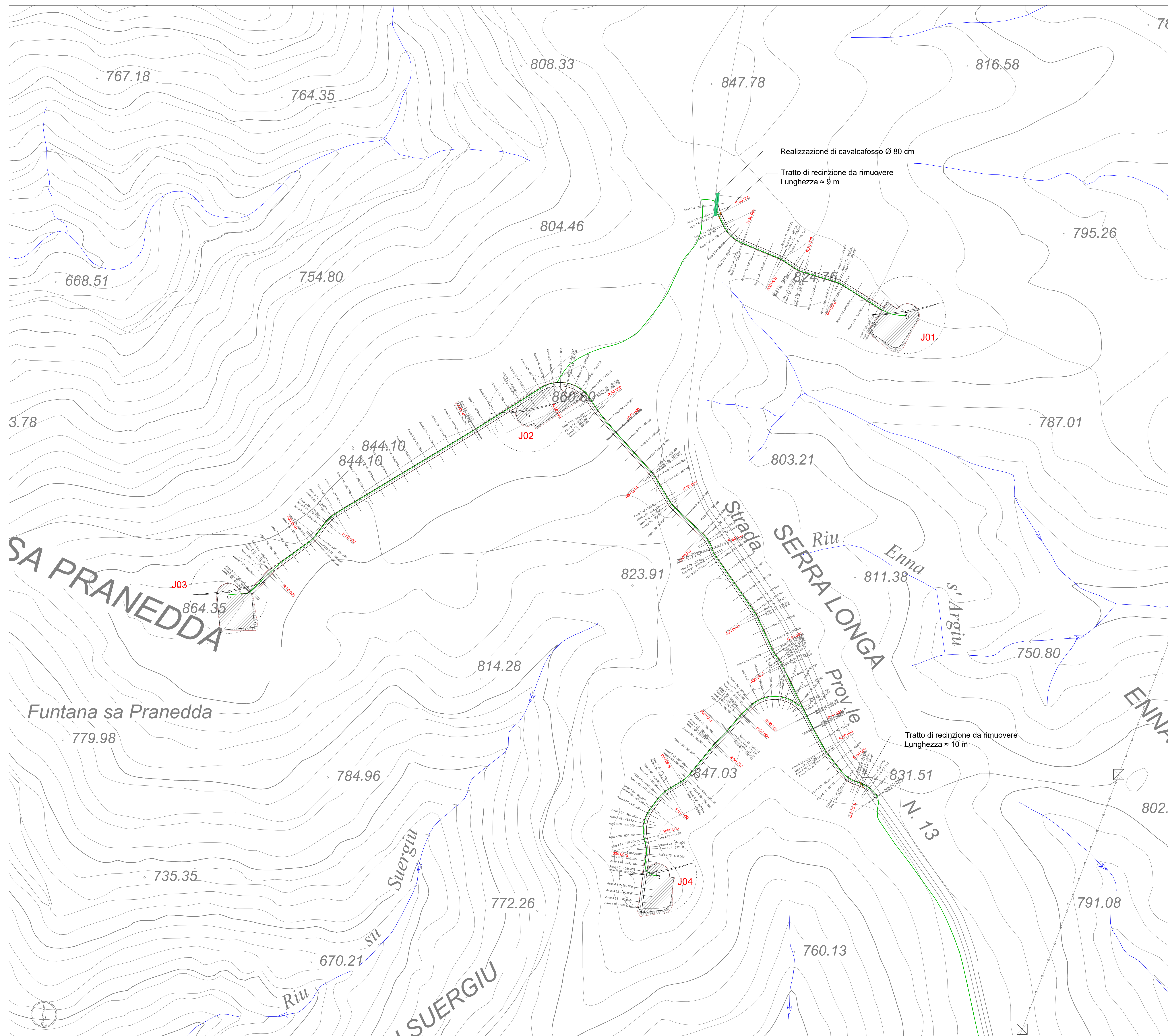
QUADRO A - VIABILITA' E PIAZZOLE - PLANIMETRIA DI PROGETTO - Scala 1:2.000
