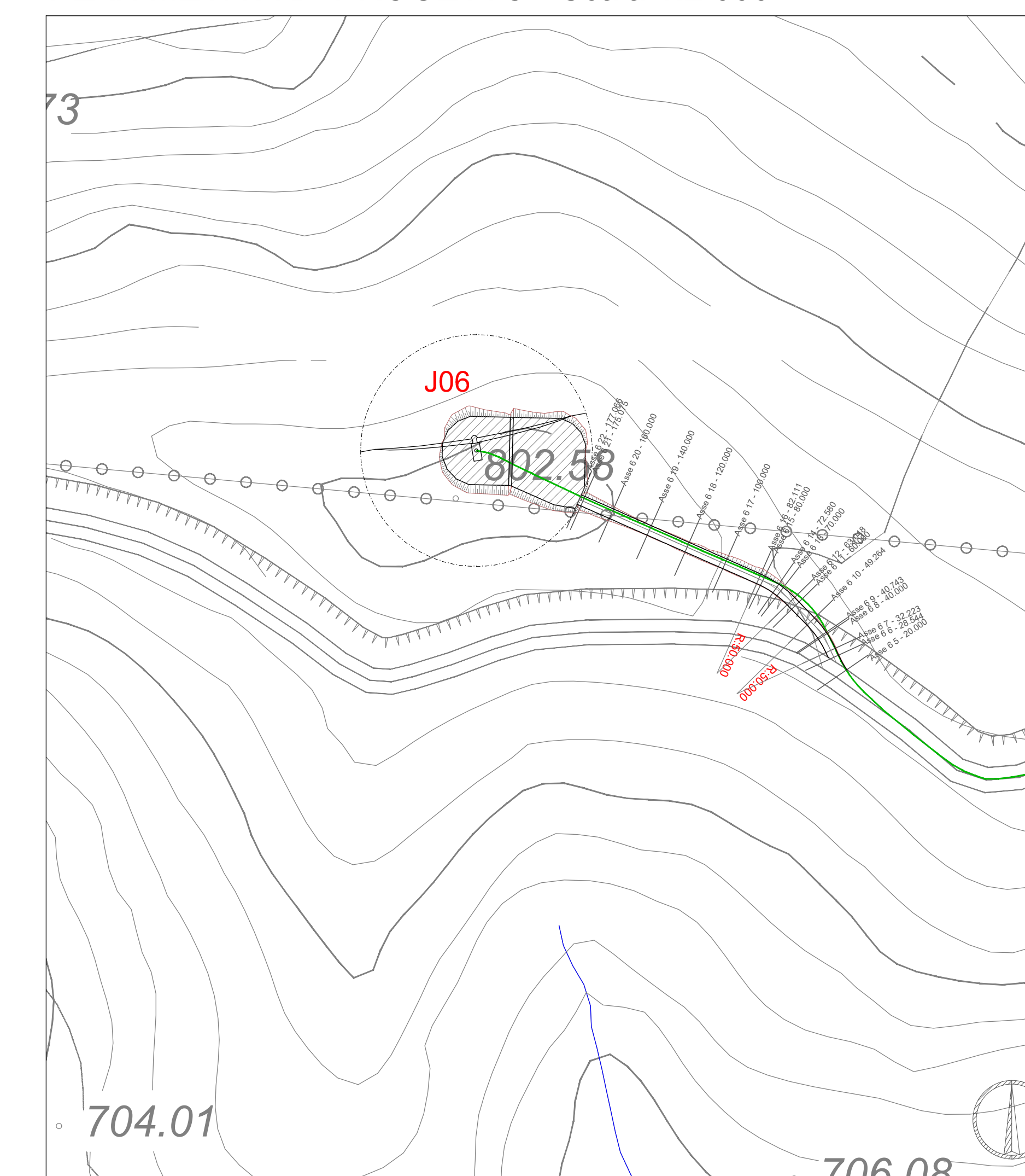
QUADRO B - VIABILITA' E PIAZZOLE - PLANIMETRIA DI PROGETTO - Scala 1:2.000
