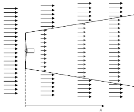
Figura 10 Andamento della scia provocata dalla presenza di un aerogeneratore. [Caffarelli-De Simone Principi di progettazione di impianti eolici Maggioli Editore]
