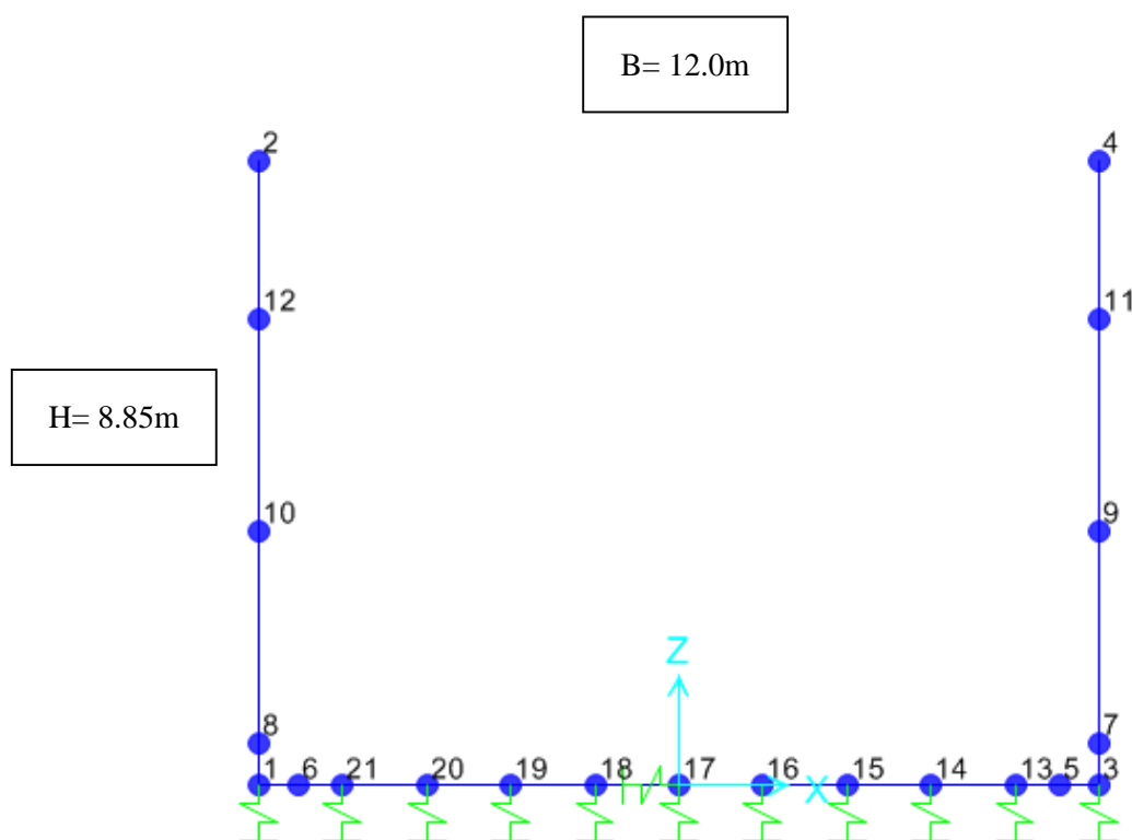
Figura 5: Numerazione dei nodi nel modello strutturale
