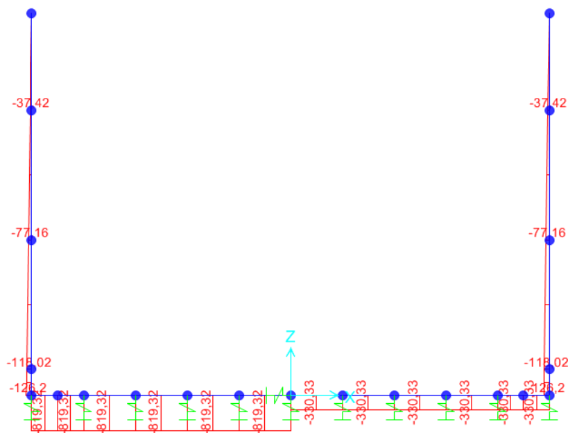
Figura 13: N - SISMA
