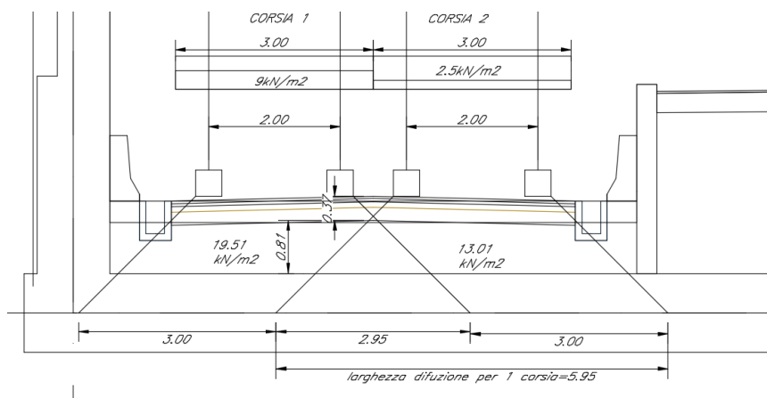
Figura 8: Schema di distribuzione del carico mobile considerato ACC1
