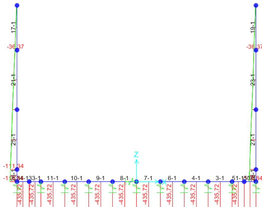
Figura 16: N - SLE RARA
