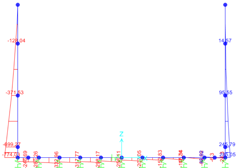
Figura 14: T - SISMA
