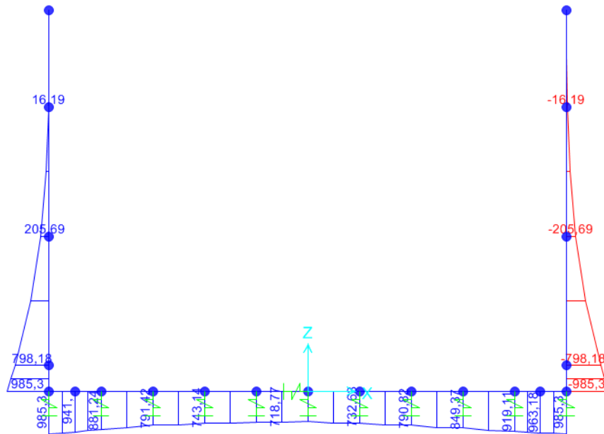
Figura 21: M – SLE QP
