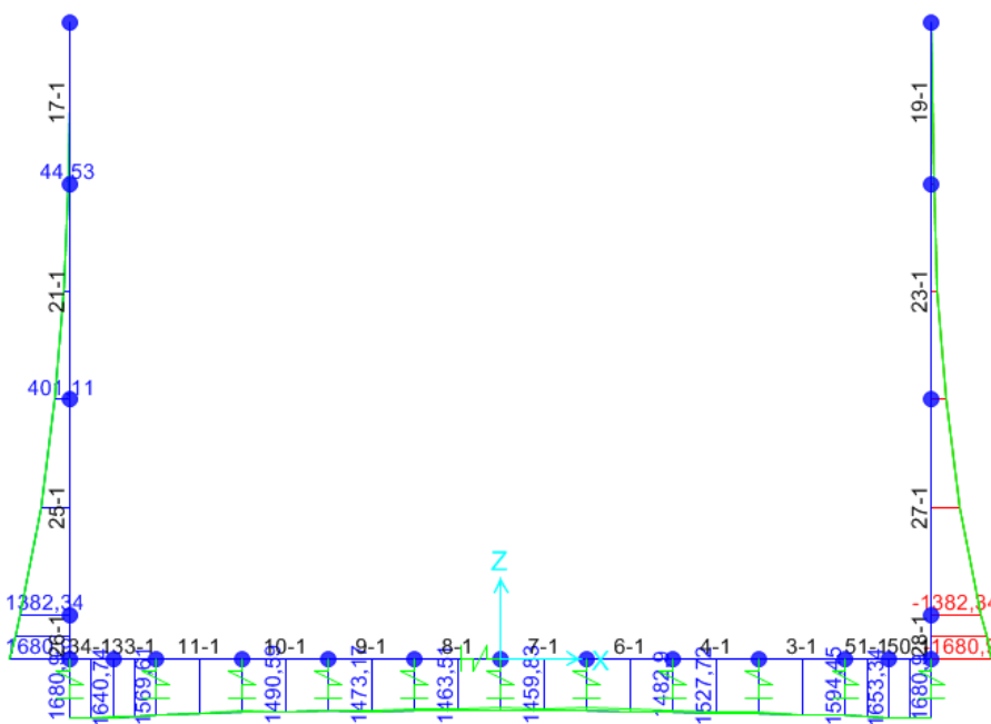
Figura 12: M - SLU
