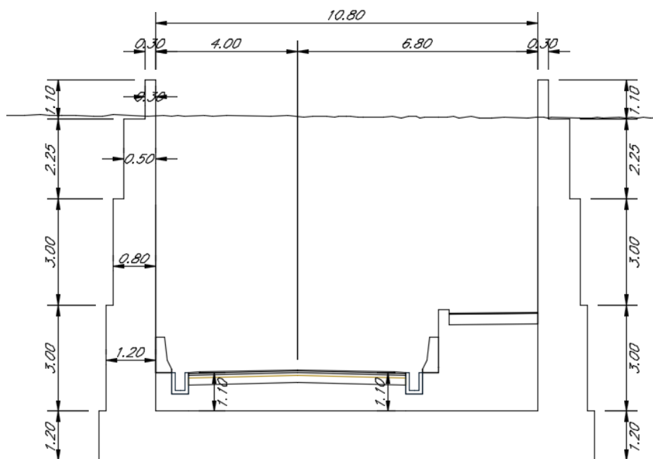
Figura 1: Sezione trasversale ( muro ad U)
