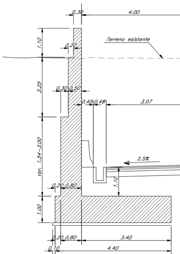
Figura 3: Sezione trasversale ( muro di sostegno Tipo 2)
