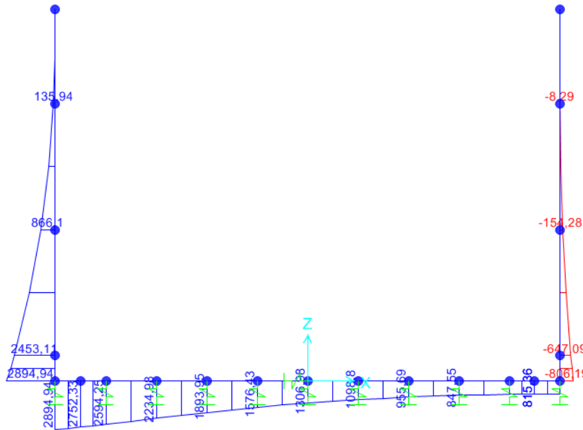
Figura 15: M - SISNA
