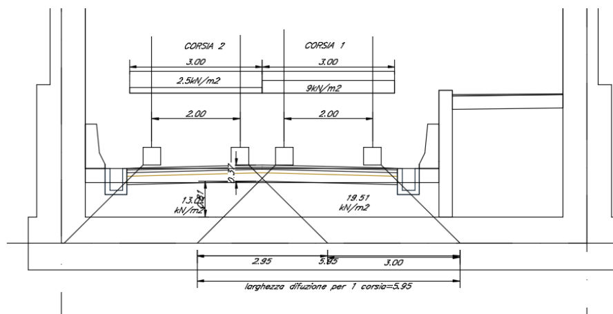
Figura 9: Schema di distribuzione del carico mobile considerato ACC2
