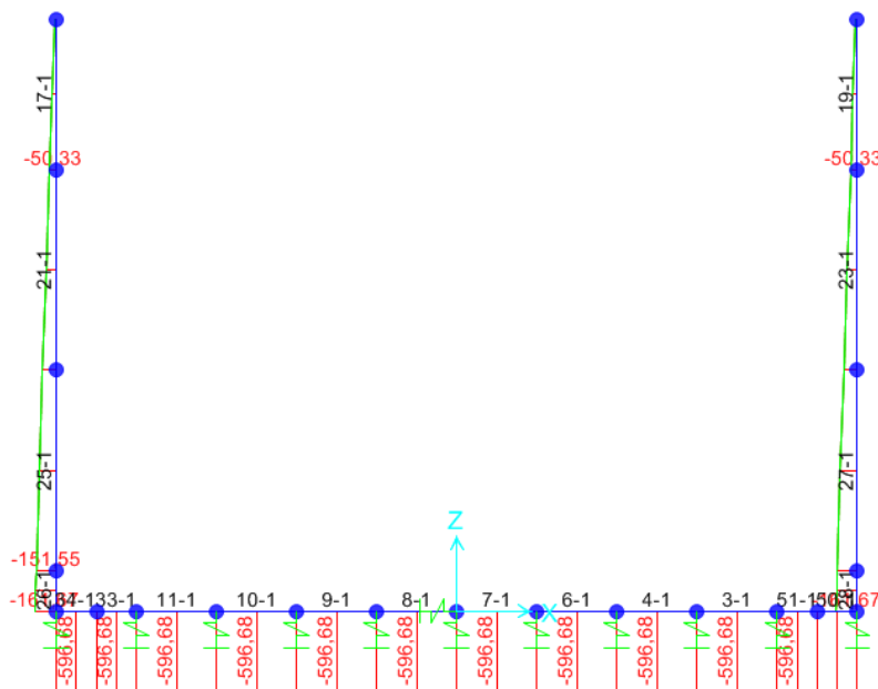
Figura 10: N - SLU
