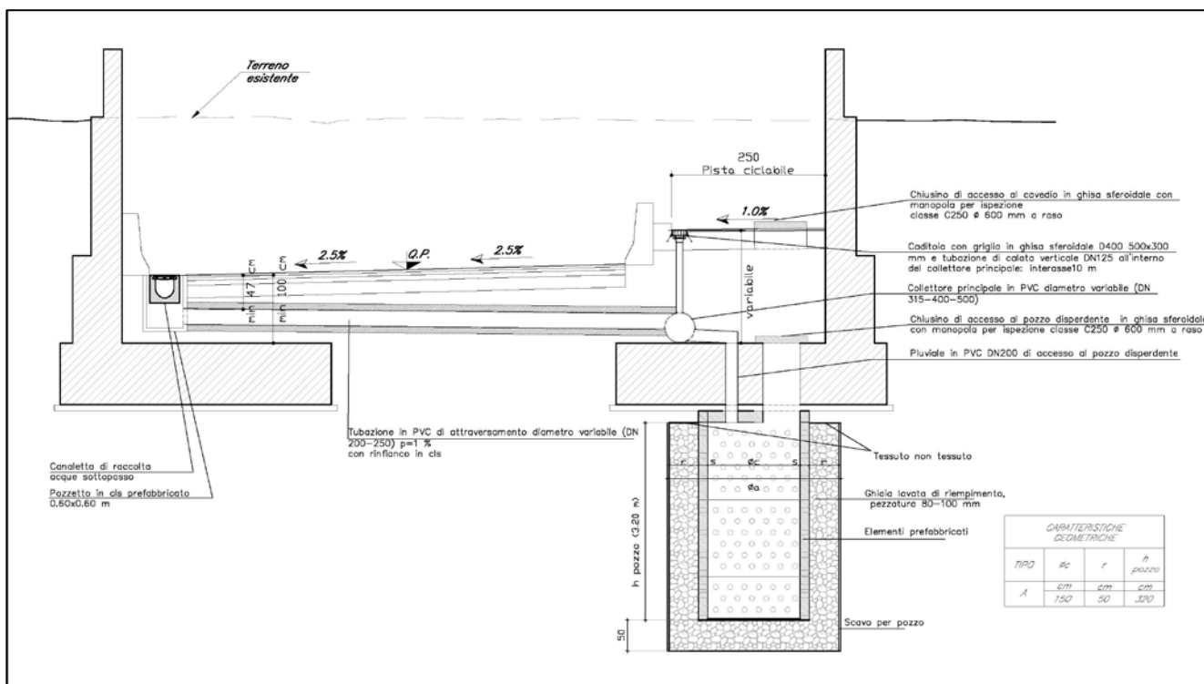
Figura 5-1- Sezione tipologica smaltimento acque meteoriche sottopasso
