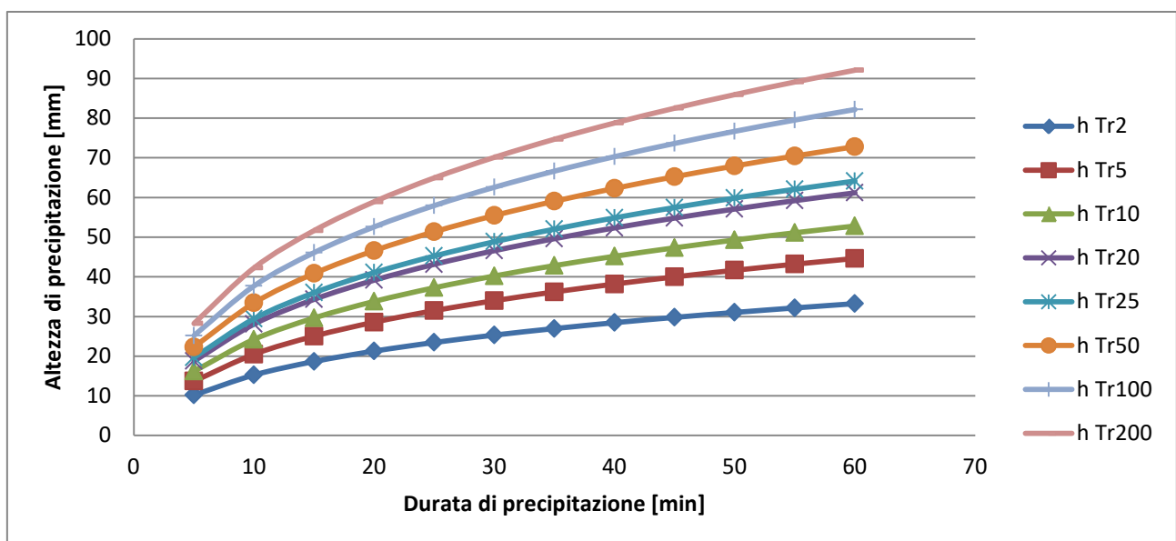
Figura 4-3- Curve di possibilità pluviometrica di durata inferiore ad un'ora
