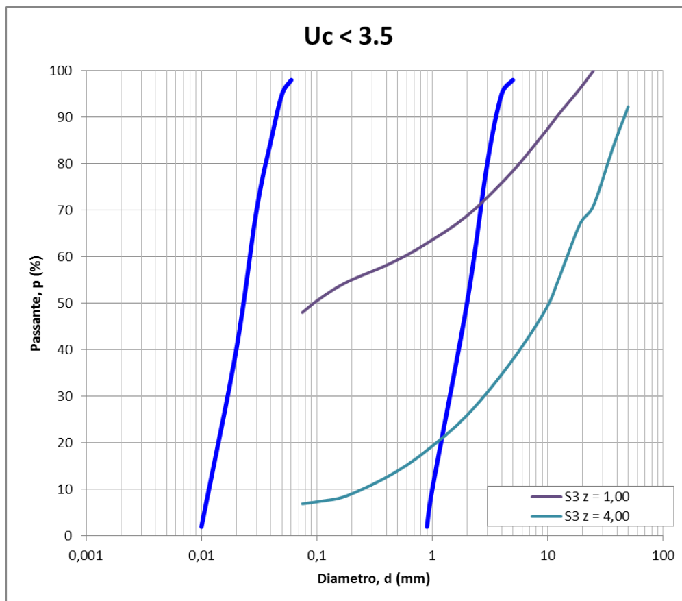
Figura 19 - Fusi granulometrici di terreni suscettibili di liquefazione dei due campioni alle profondità di 1m e 4m da piano campagna.
