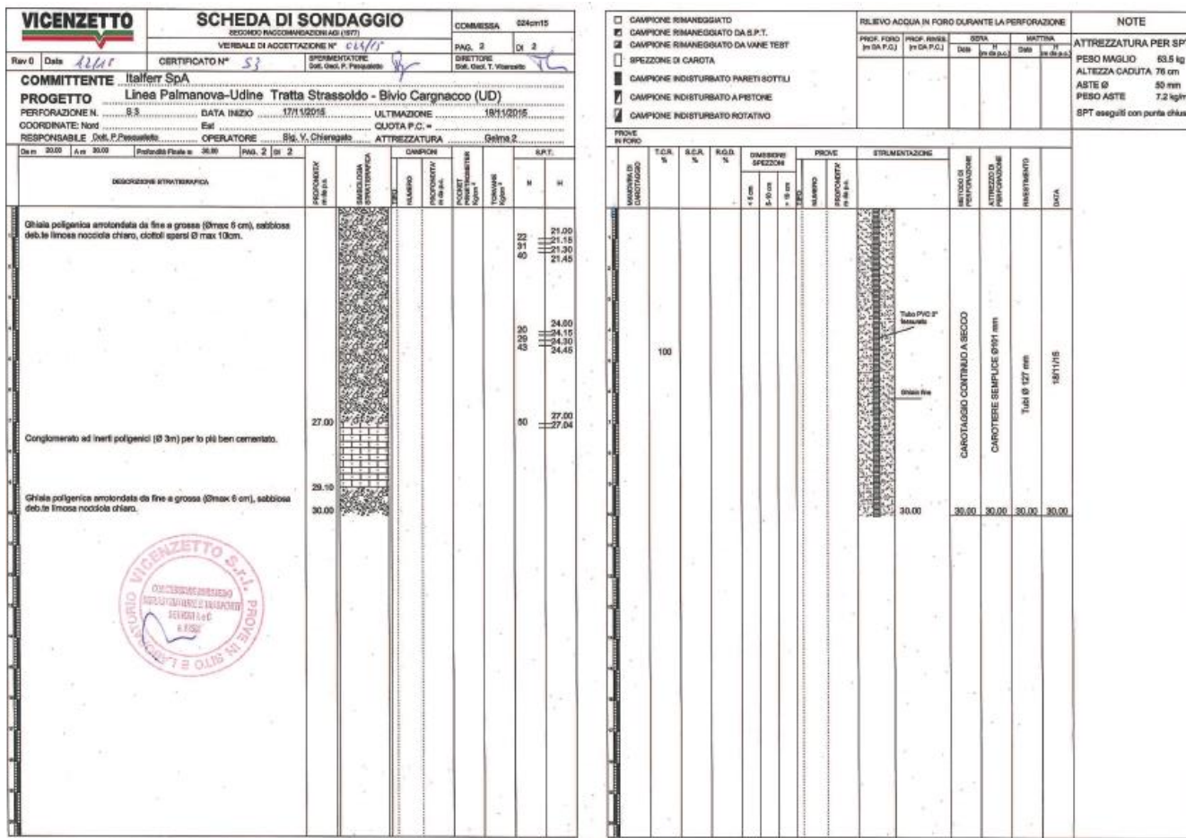
Figura 8 – Stratigrafia del sondaggio S3.
