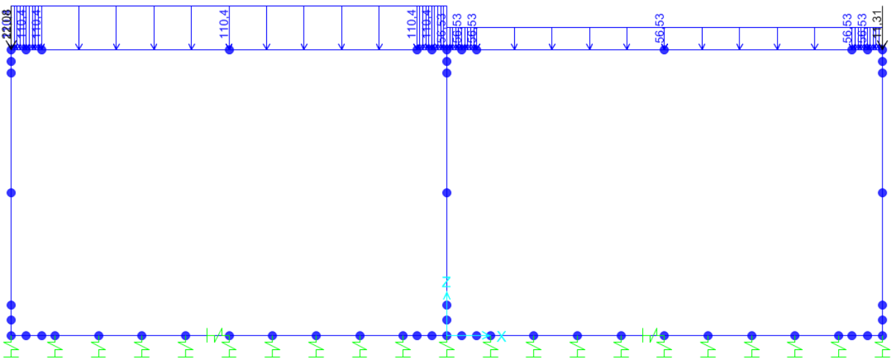
Figura 14: Carichi Treno LM71 condizione Taglio massimo ACC2
