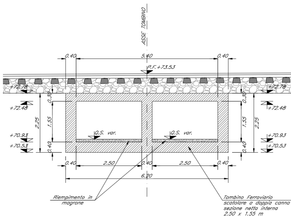
Figura 1: Sezione trasversale- tombino ferroviario
