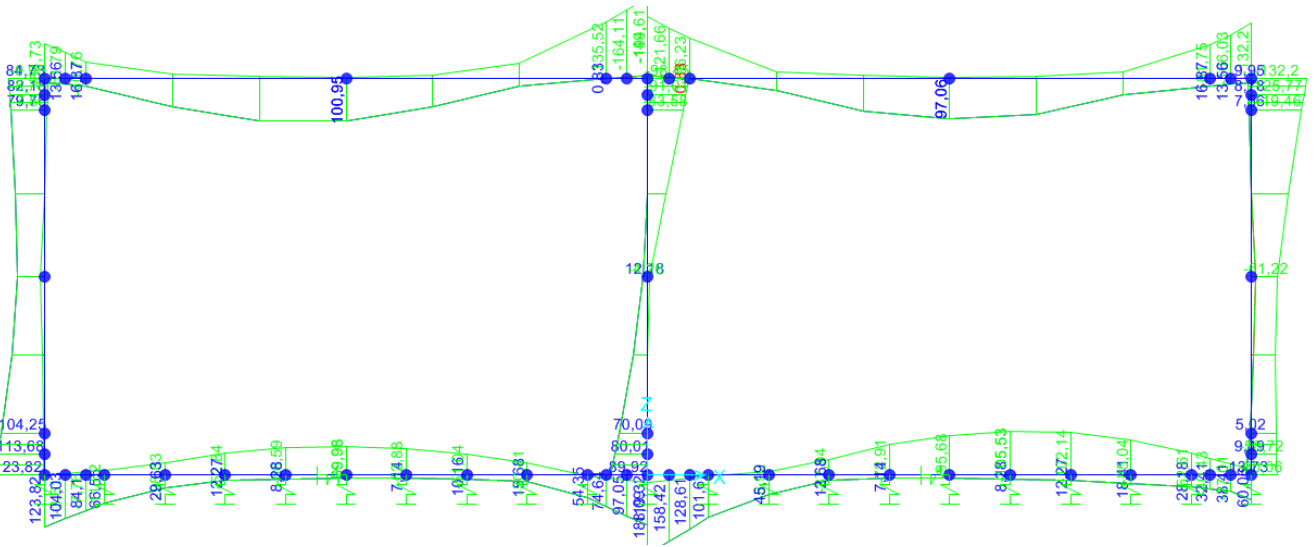
Figura 22: Involuppo M - SLU
