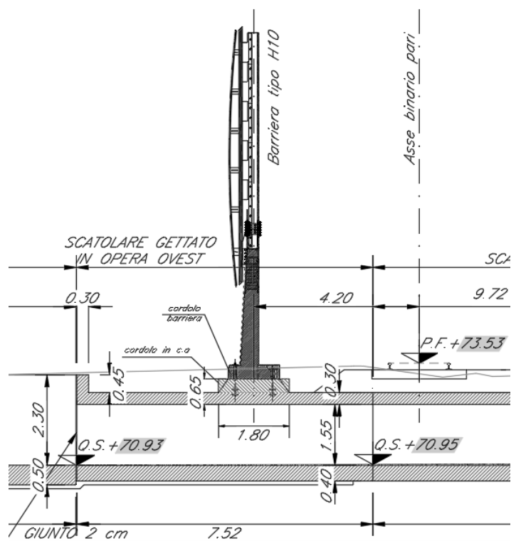
Figura 48 – Barriera su tombino ferroviario IN01
