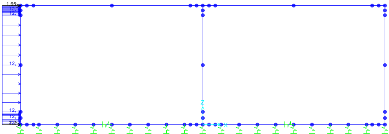
Figura 18: Sovraspinta sismica del terreno
