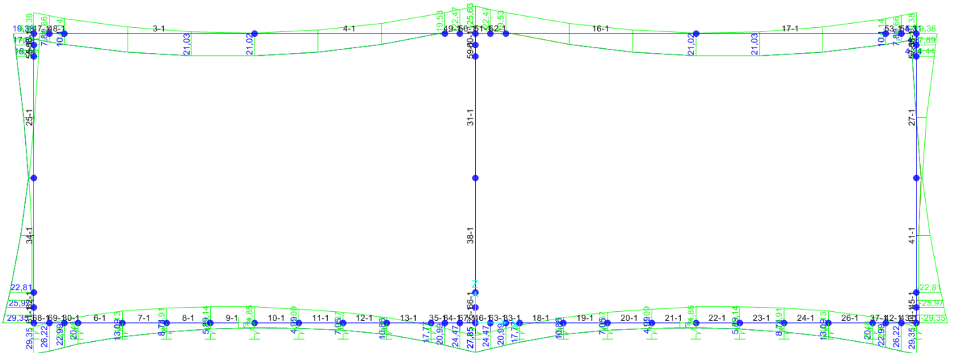
Figura 28: Involuppo M – SLE QP
