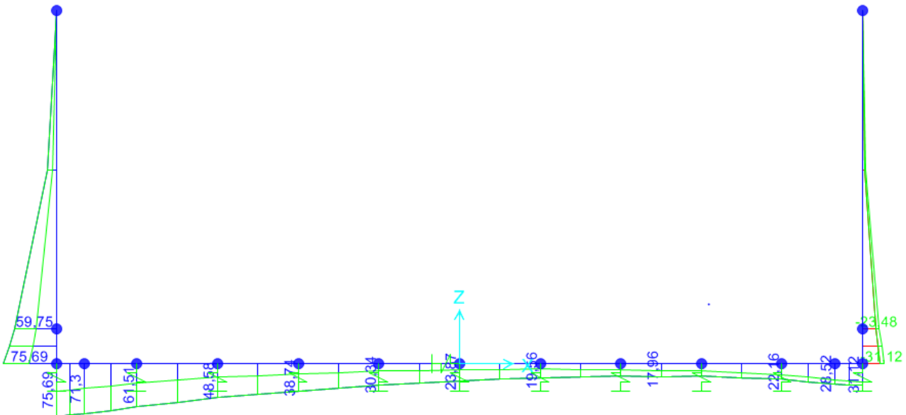
Figura 39: Inviluppo M - SLV
