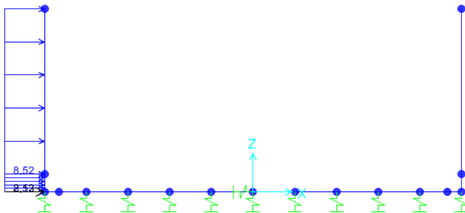
Figura 35:Spinta accidentale traffico
