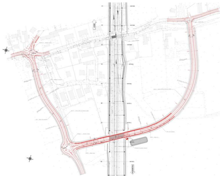
Figura 2: – Intervento SL01
