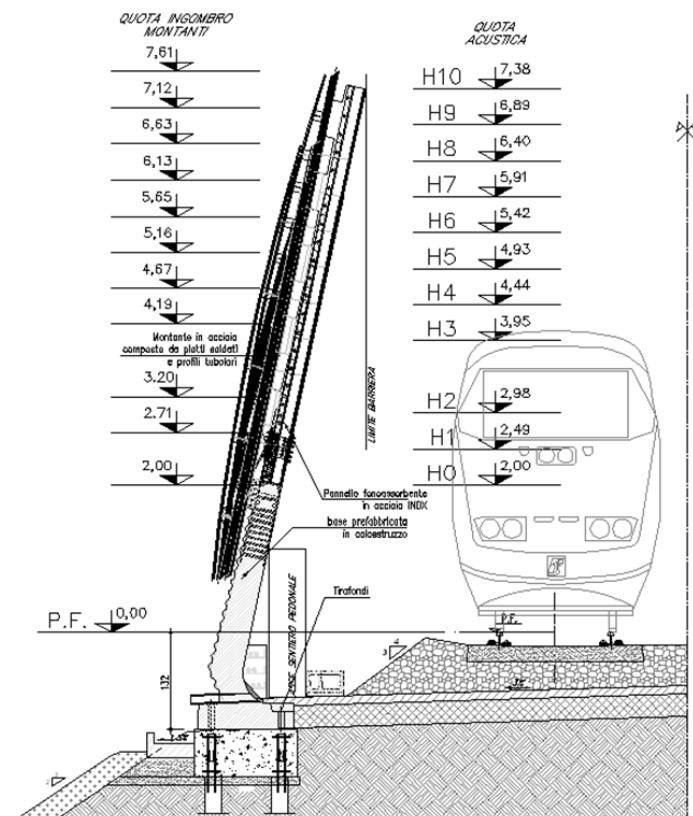
Figura 13: Barriere antirumore
