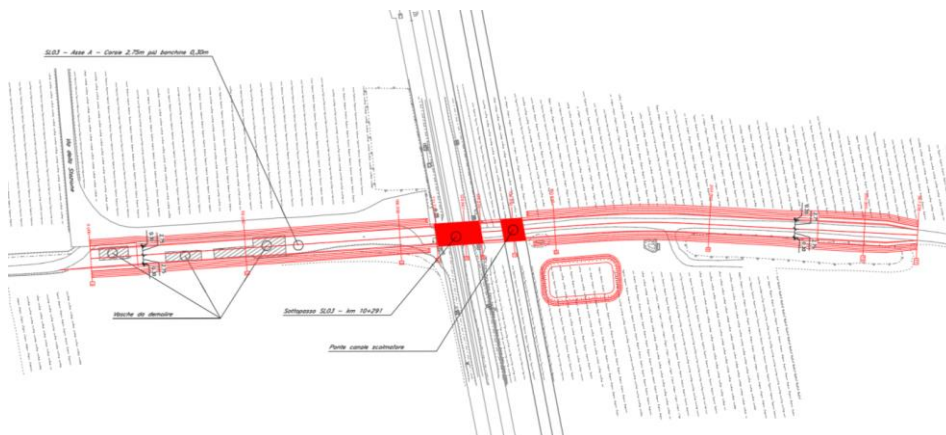
Figura 6: – Intervento SL03
