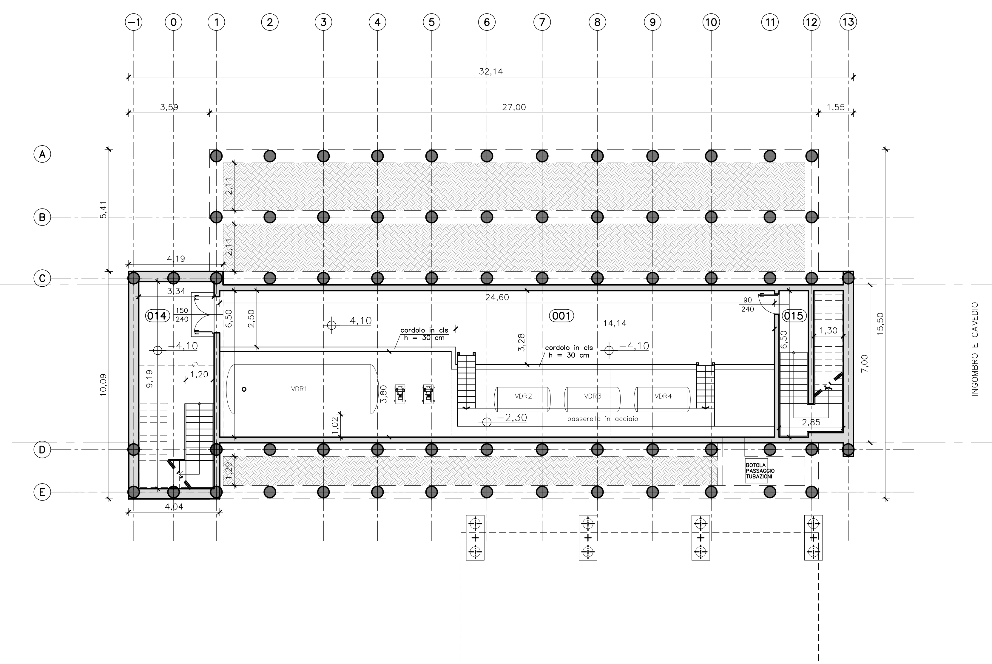
PIANTA QUOTA -4,10 SCALA 1:100
