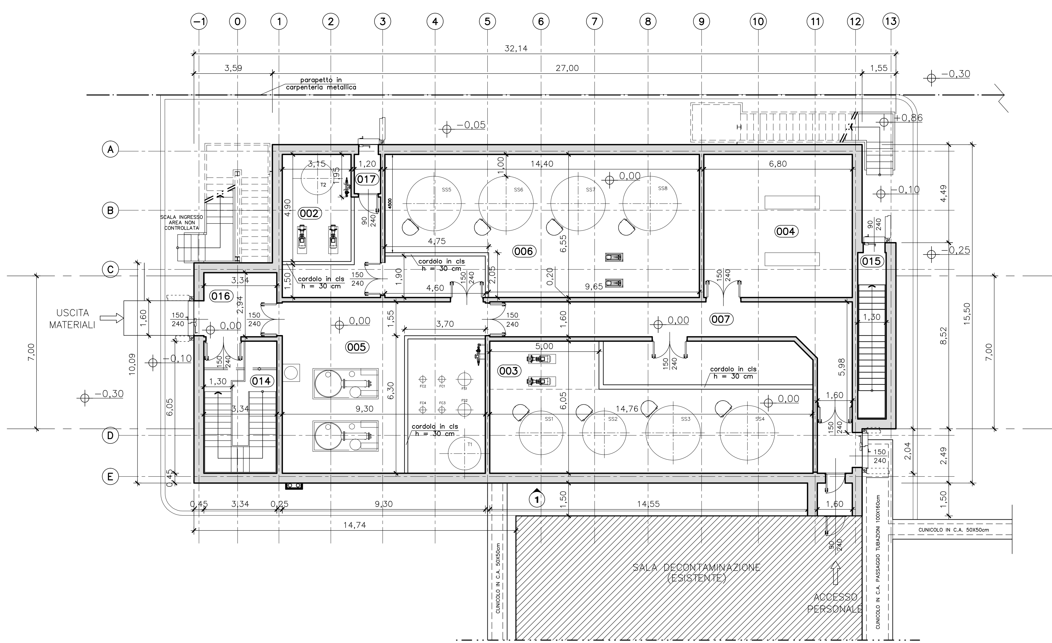
PIANTA QUOTA 0,00 SCALA 1:100
