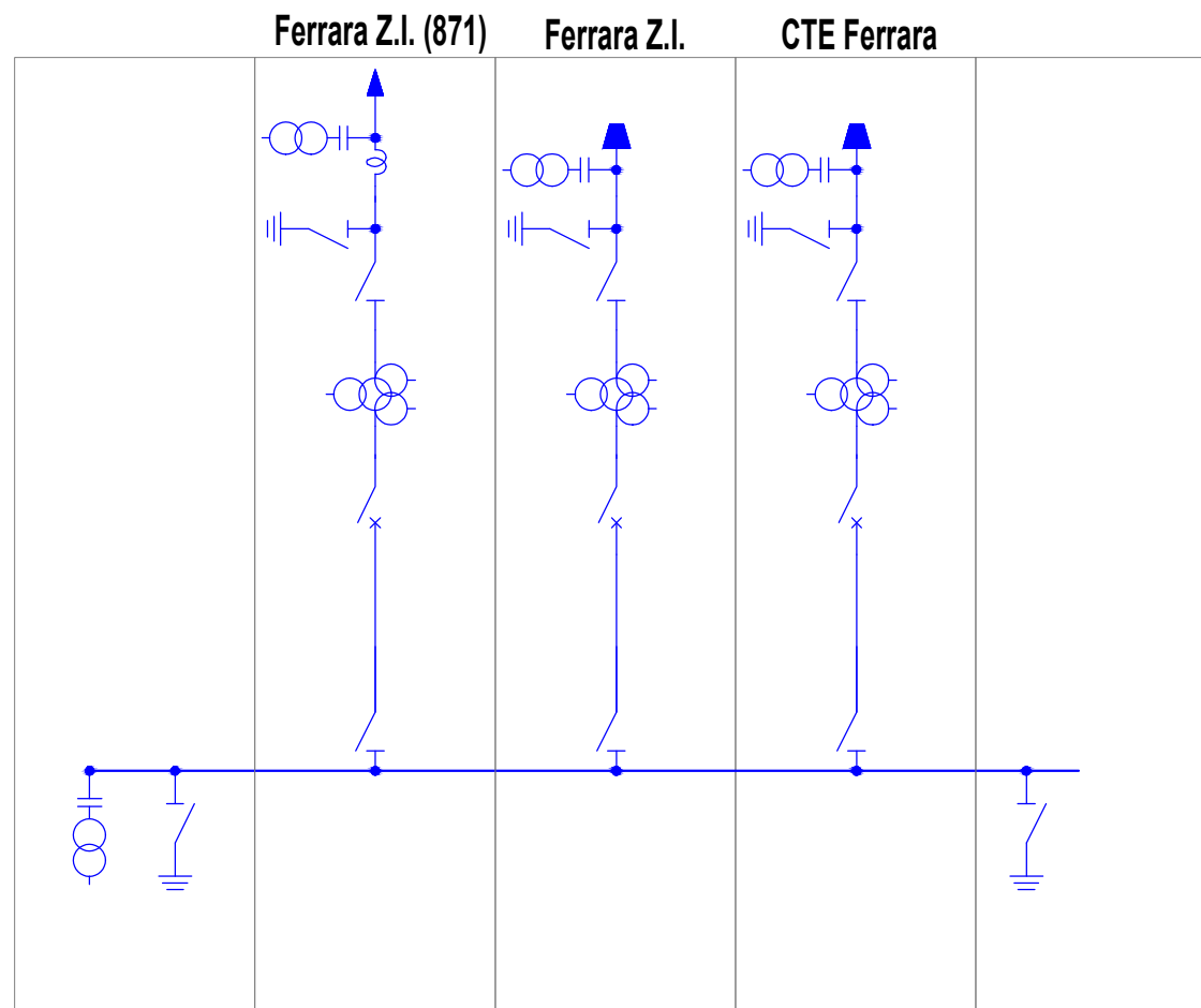
Nuova SE a 132kV di Ferrara – Schema Elettrico Unifilare
