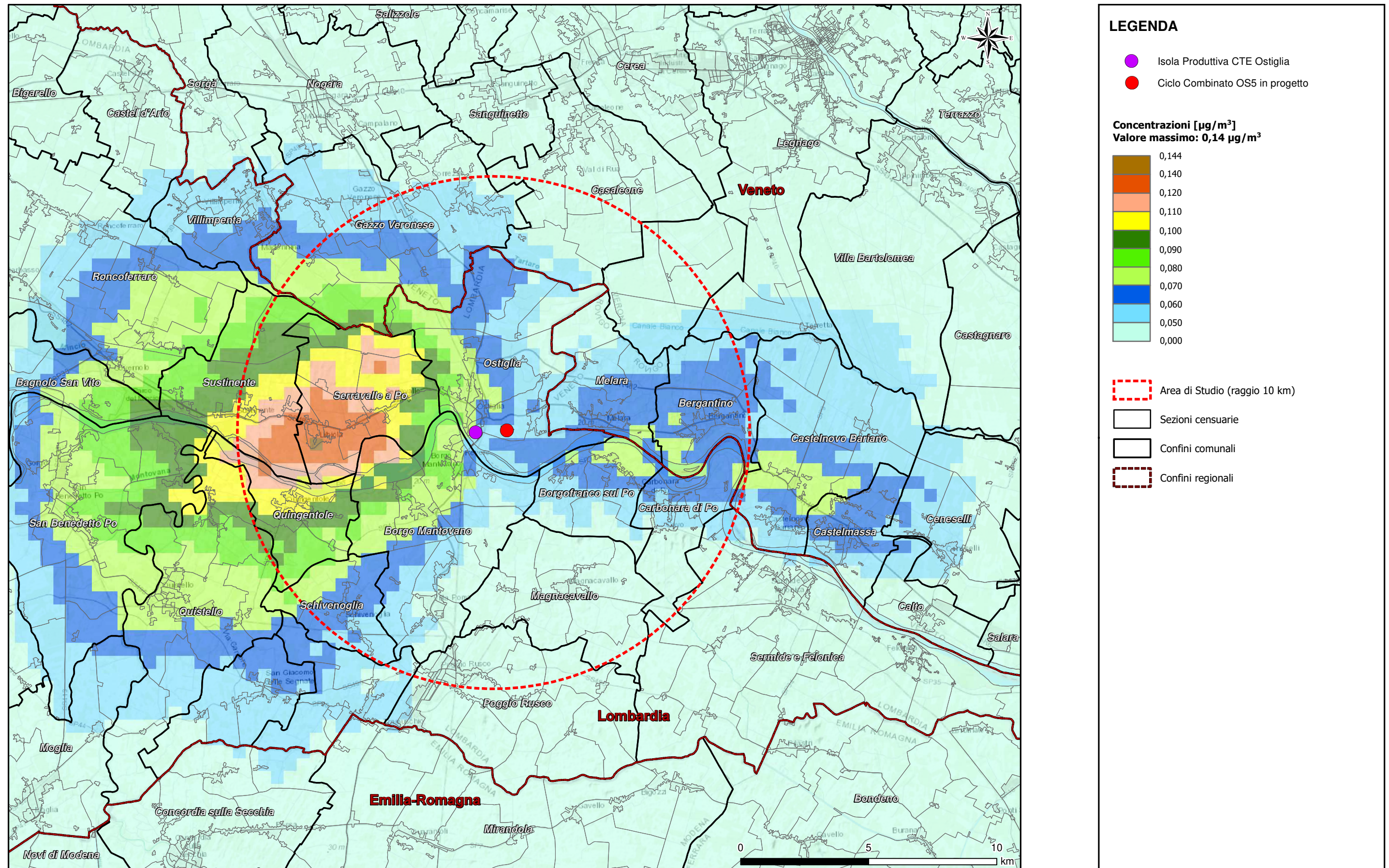
Figura 4a ScENARIO Attuale - 90,4° percentile delle concentrazione medie giornaliere di Particolato secondario
