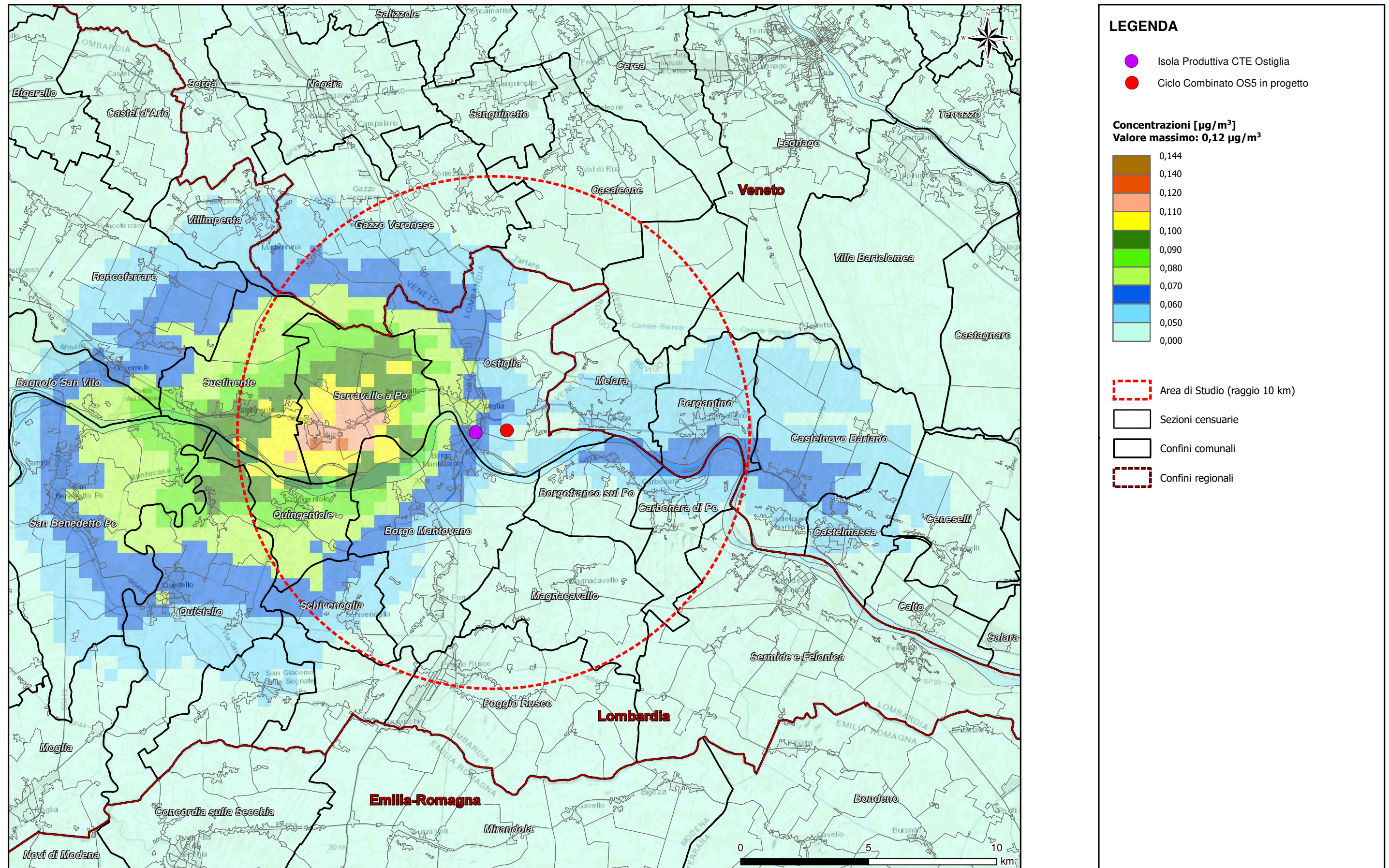
Figura 4c Scenario Futuro - 90,4° percentile delle concentrazione medie giornaliere di Particolato secondario
