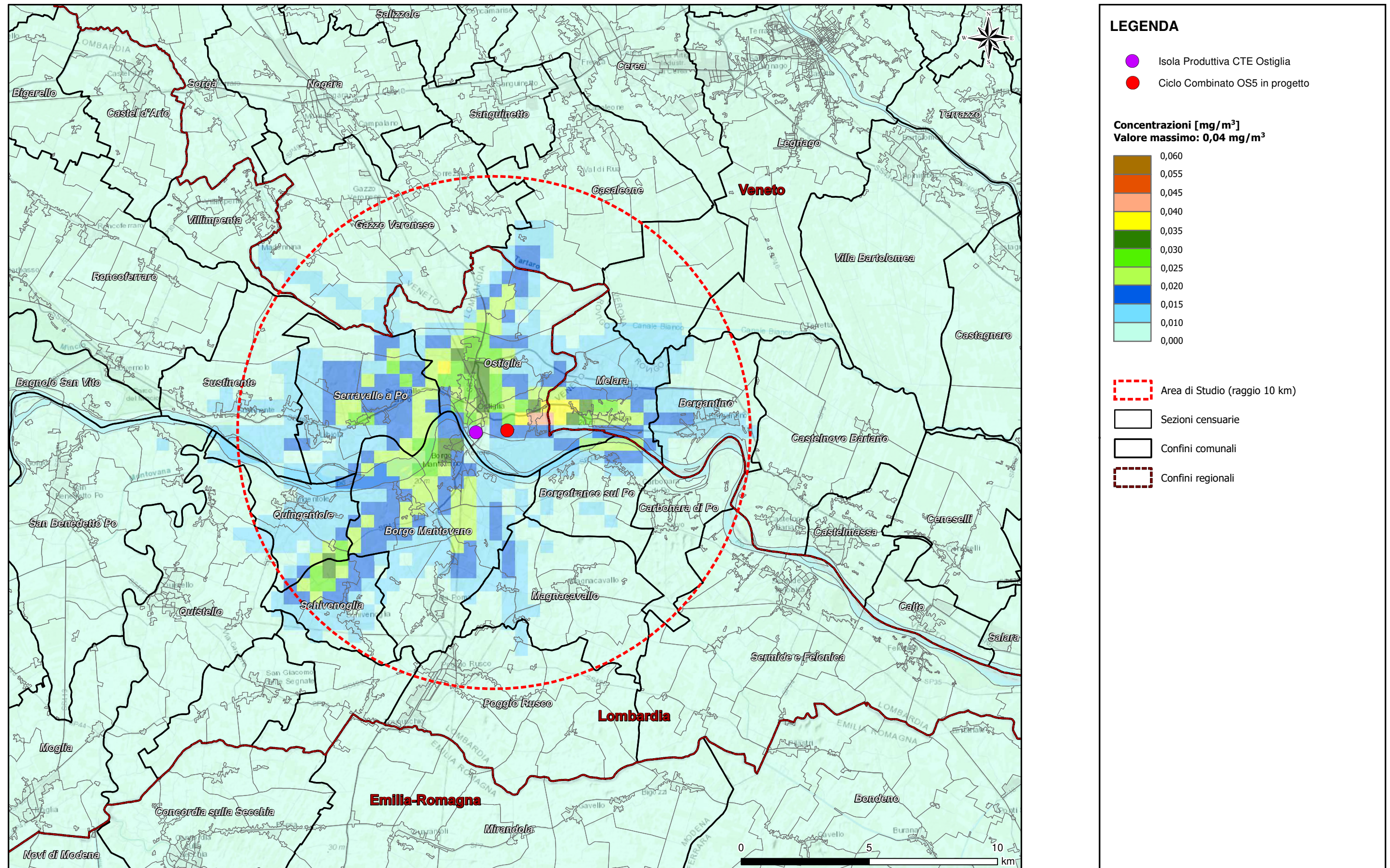
Figura 7.1a ScENARIO ATTUALE - Massime concentrazioni medie su 8 ore di CO
