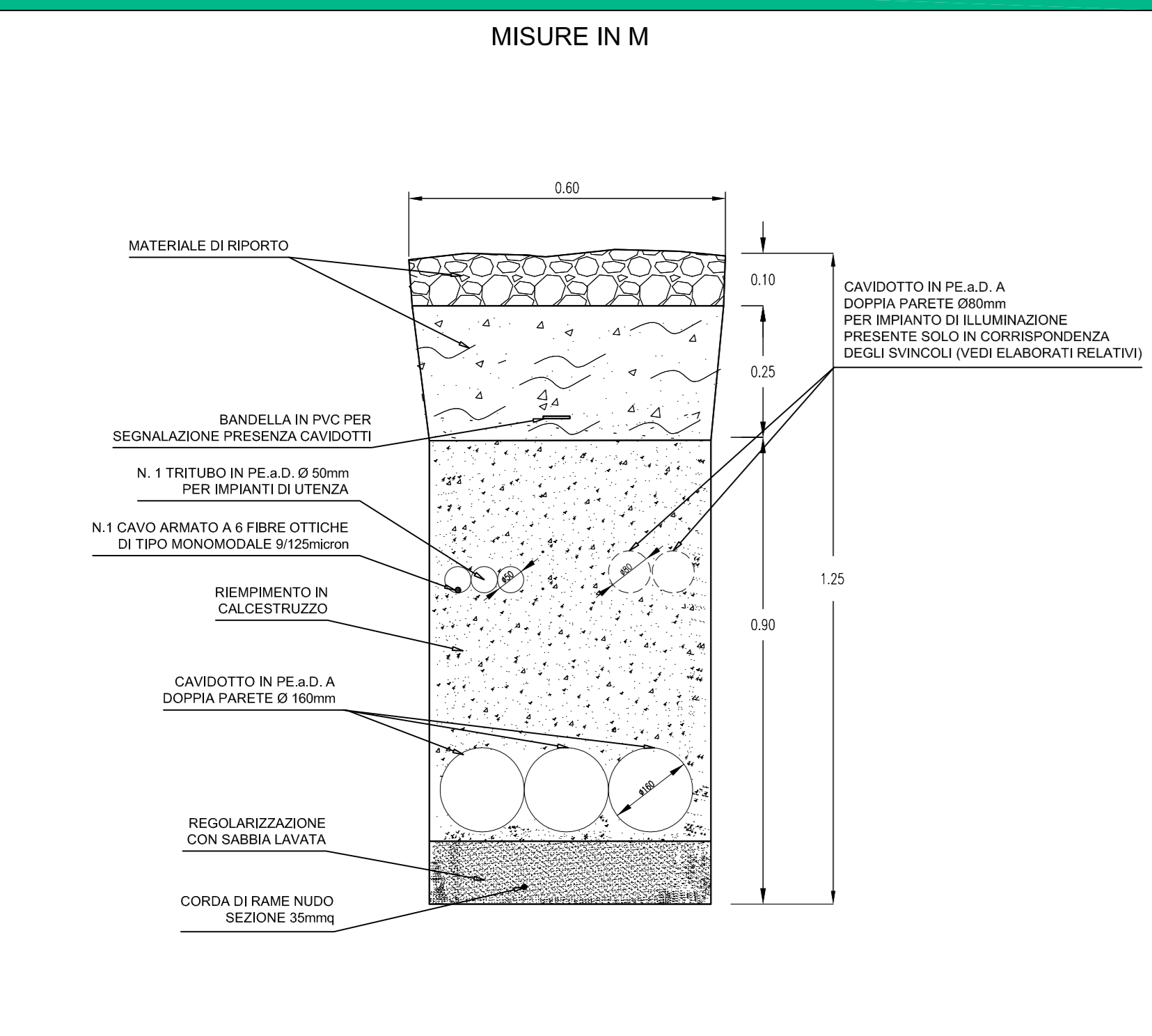
TIPICO SEZIONE DI SCAVO IN BANCHINA DIREZIONE AGRIGENTO - SCALA 1:10
