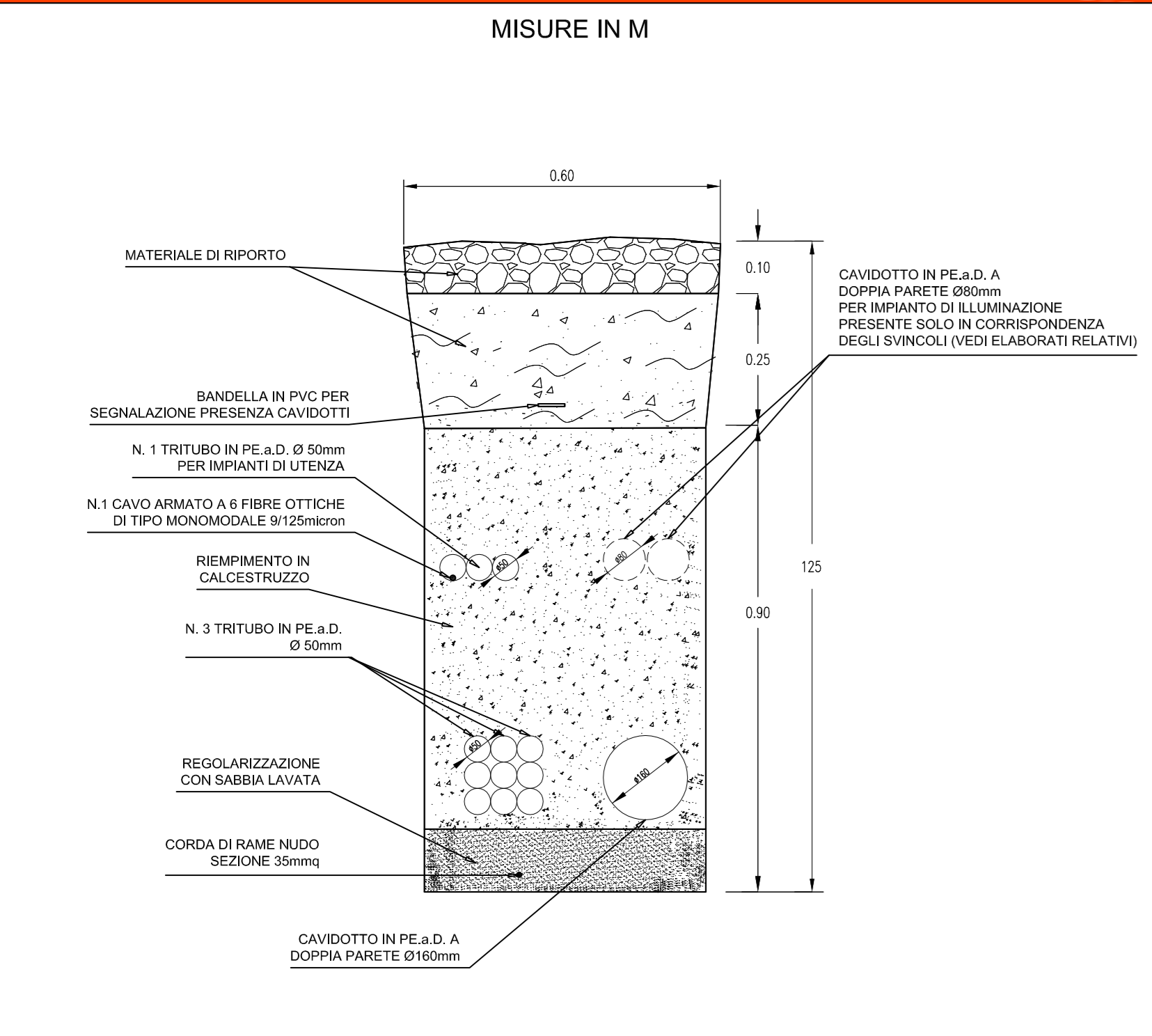
TIPICO SEZIONE DI SCAVO IN BANCHINA DIREZIONE AUTOSTRADA A19 - SCALA 1:10
