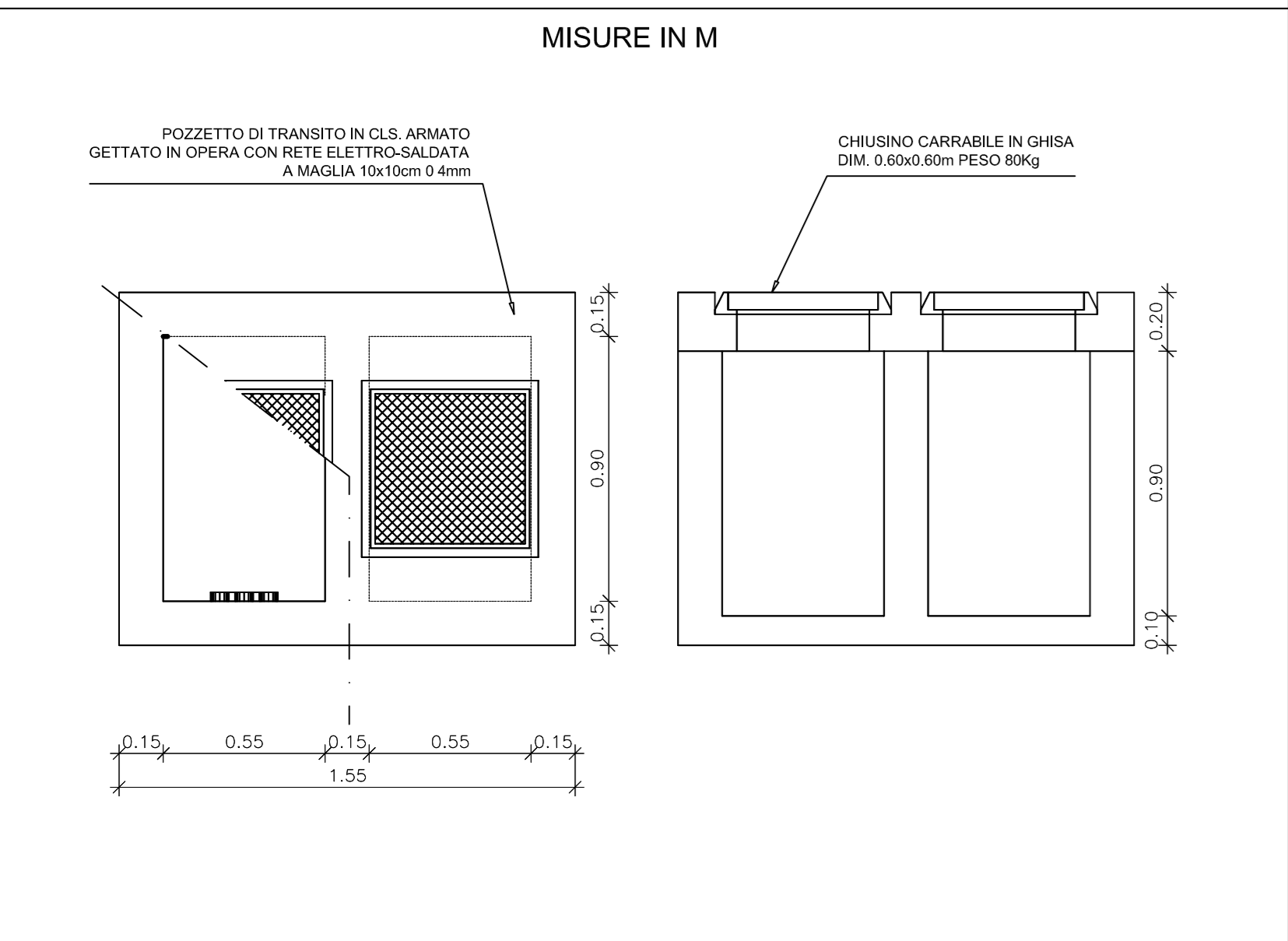
POZZETTO CON SETTO DIVISORIO INTERNO - SCALA 1:20
