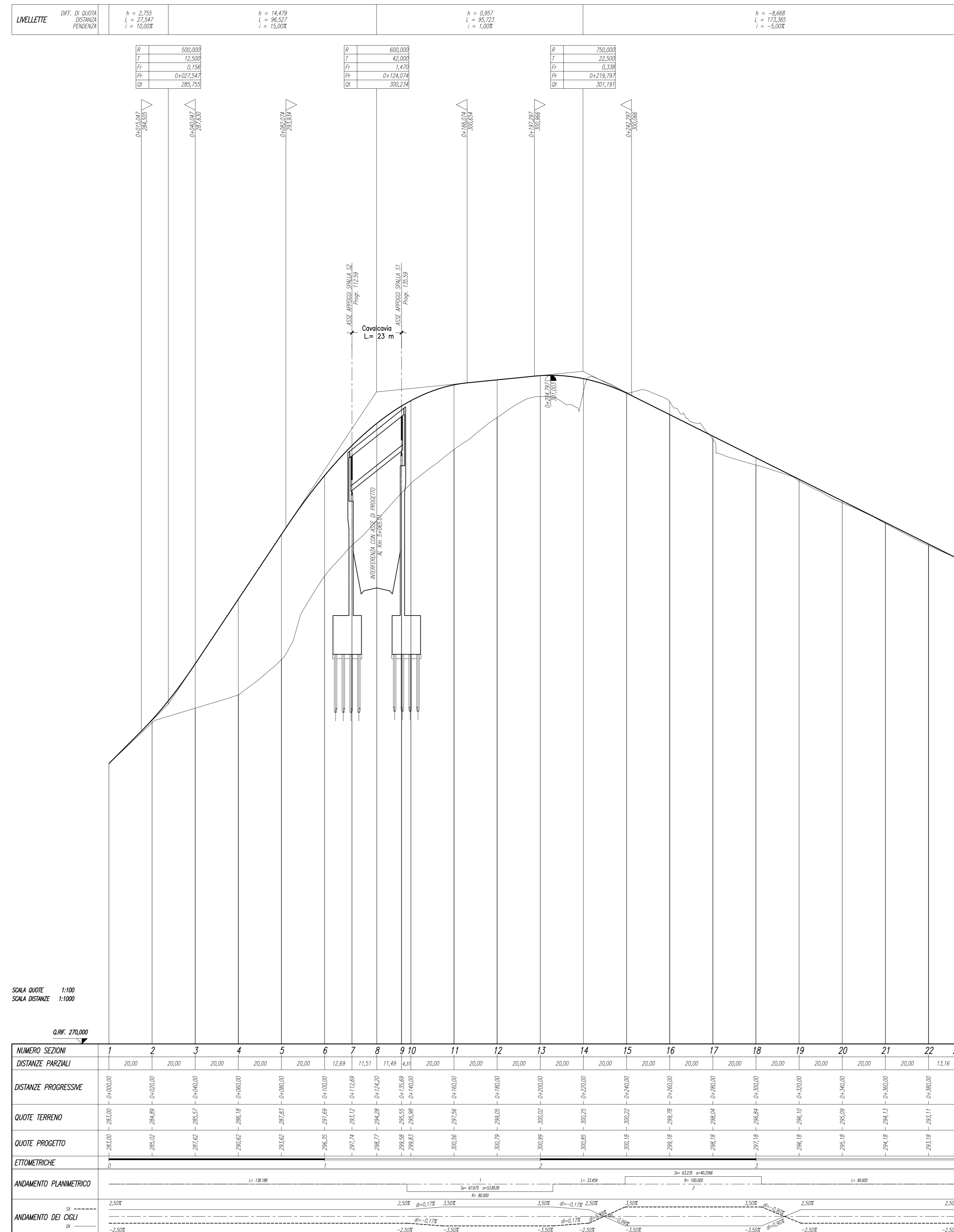
PROFILO LONGITUDINALE VIABILITA' n.6 Km 5+065.01 - Scala 1:1000/100
