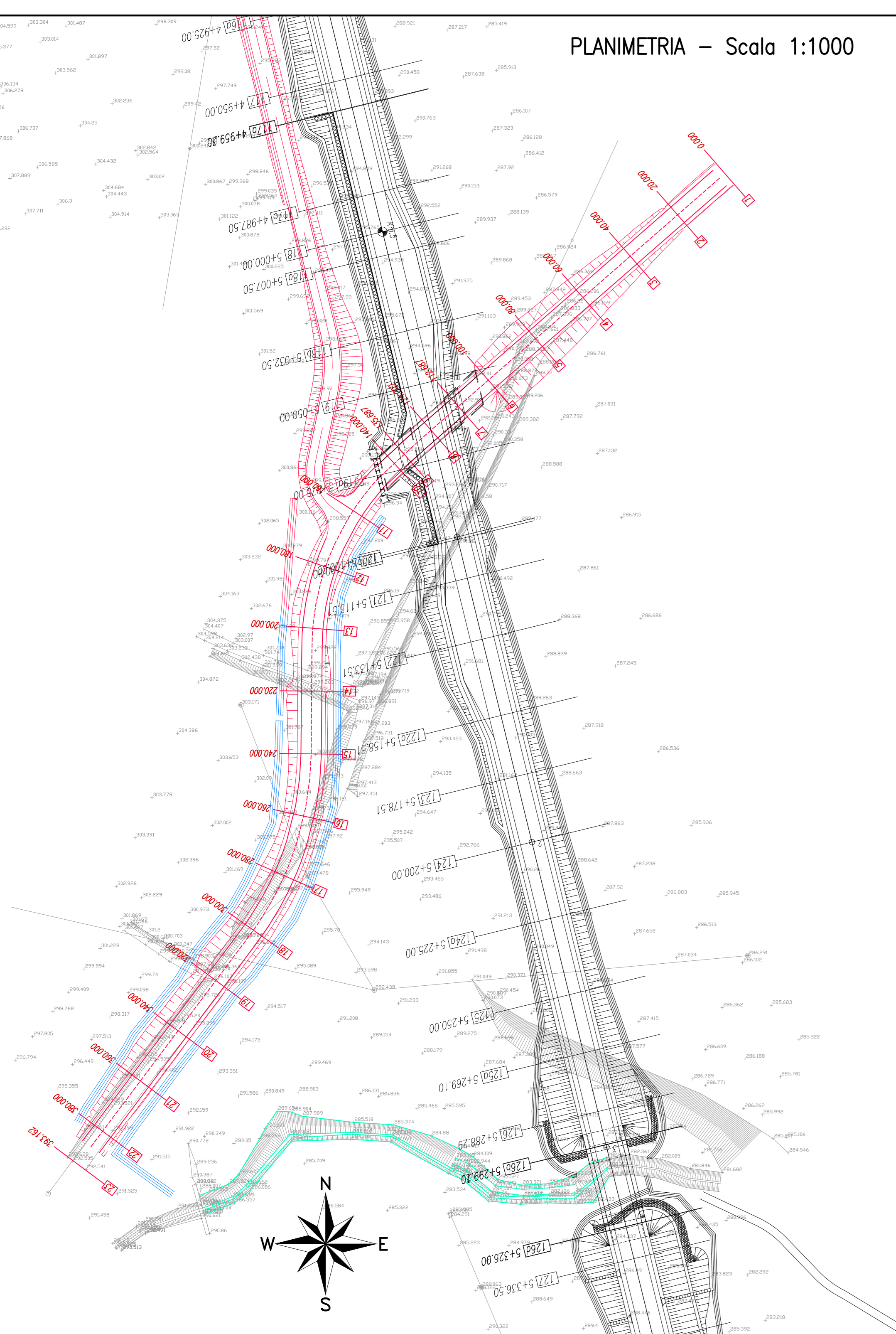
PLANIMETRIA DI TRACCIAMENTO VIABILITA' n.6 Km 5+065.01 - Scala 1:1000
