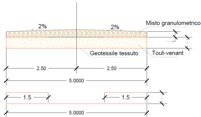
Fig.7.1 – Sezione stradale tipo
