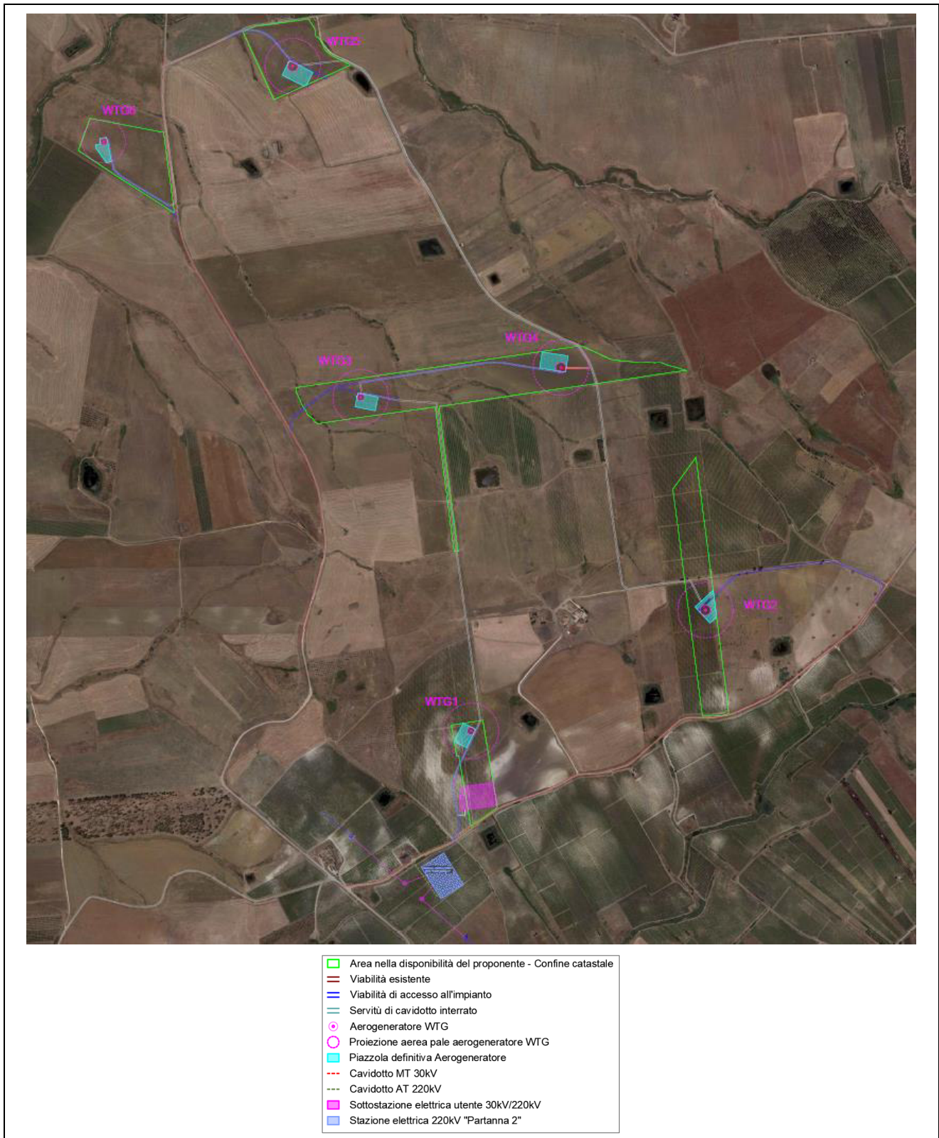
Fig. 2.3 - Localizzazione geografica dell'impianto
