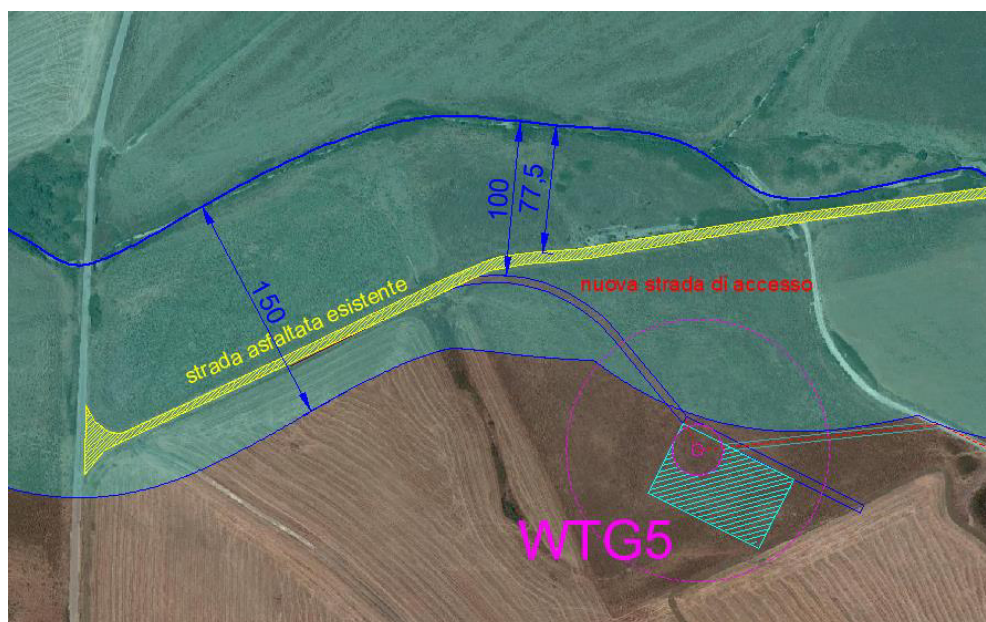
Fig.3.6 – Inquadramento su ortofoto aerea aerogeneratore WTG 5 sull'elaborato "Beni paesaggistici"
