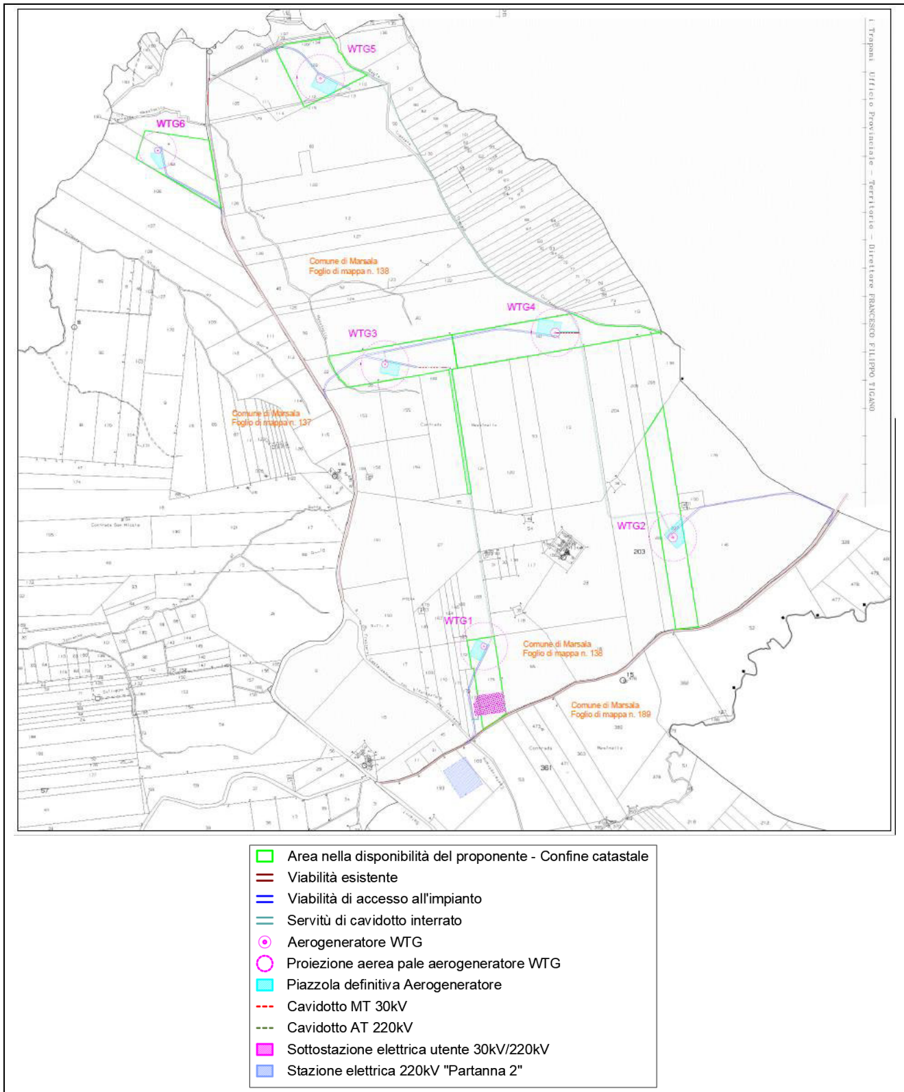
Fig. 2.2 – Inquadramento su stralcio catastale
