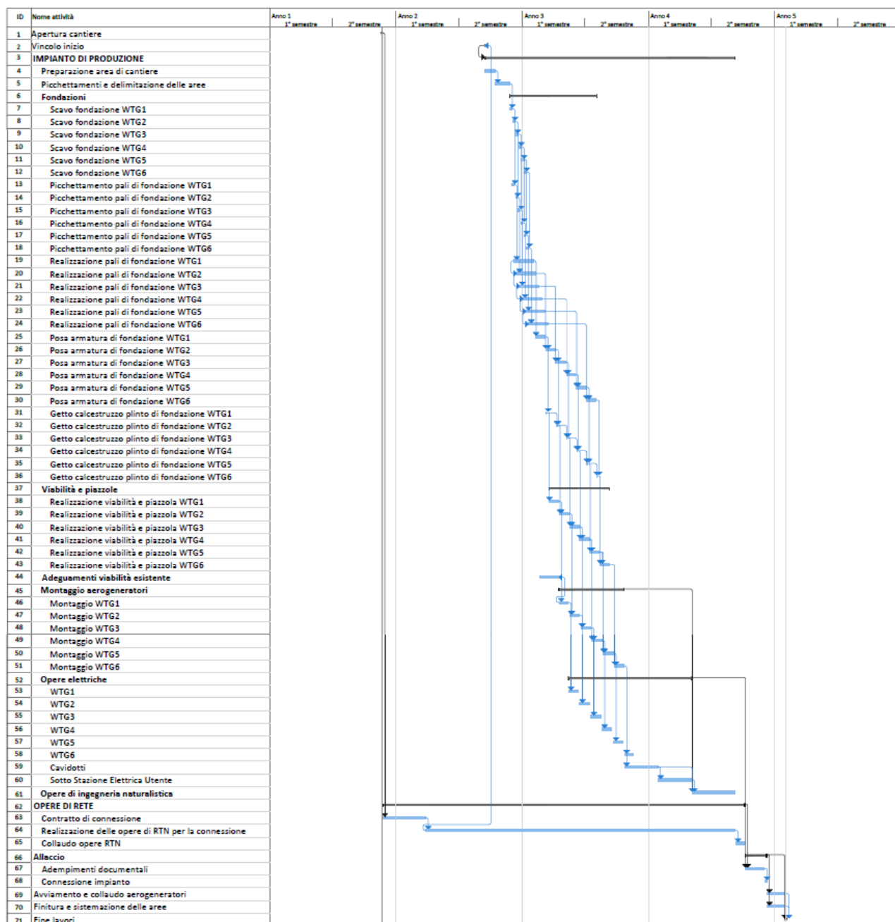
Fig.9.1 - Principali fasi lavorative
