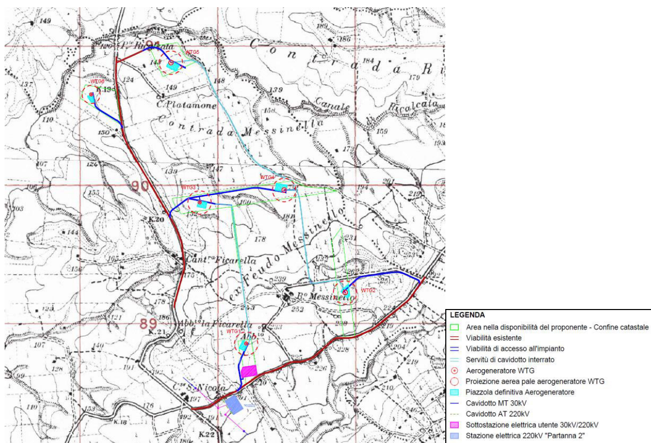
Fig.7.2 — Corografia IGM con indicazione cavidotti
