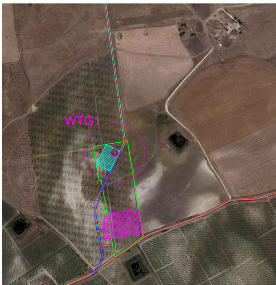
Figura 5-10. Inquadramento dell'area dell'aerogeneratore WTG 1
