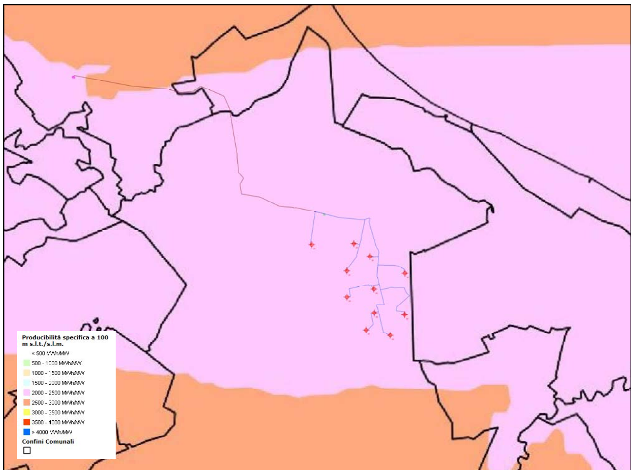
Impianto su Atlante eolico interattivo con producibilità specifica a 100 m s.l.m.
