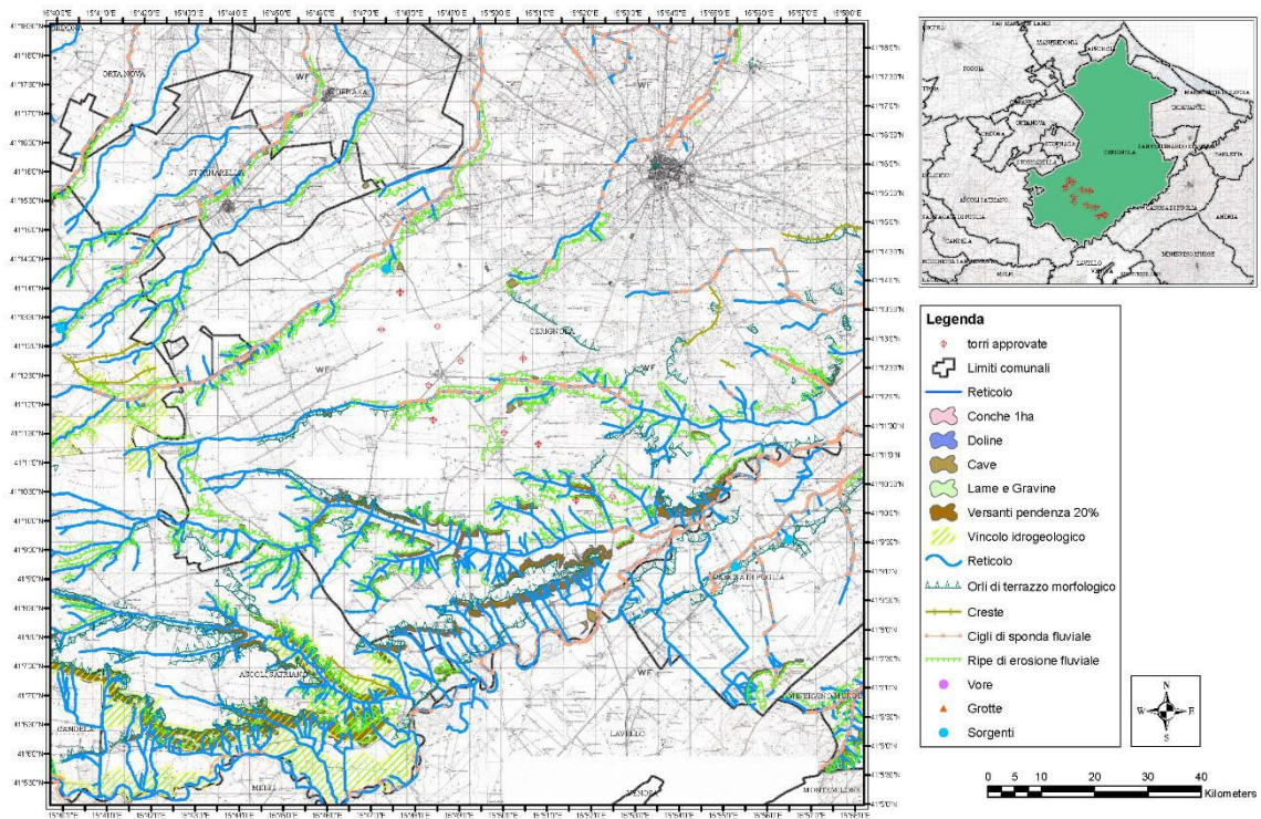
Sistema geomorfoidrogeologico
