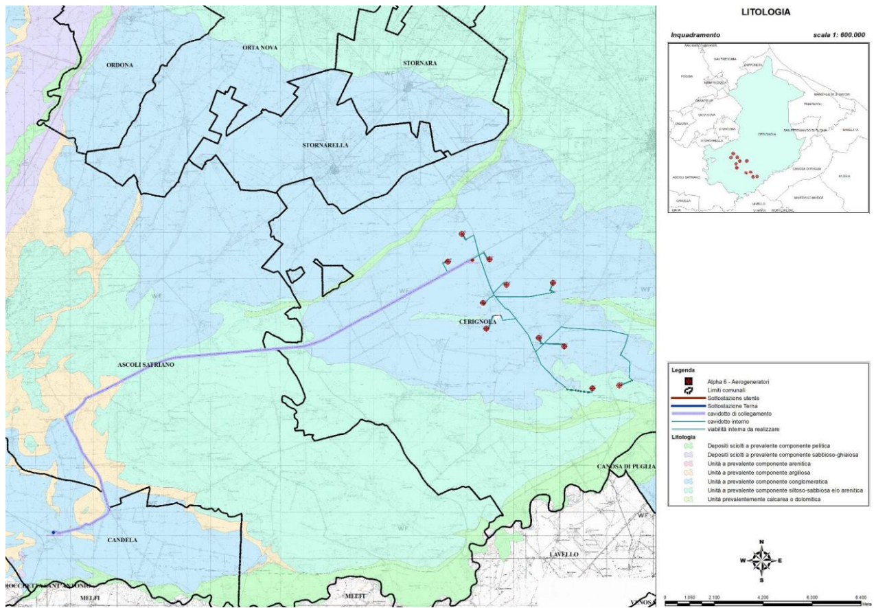
Carta geolitologica
