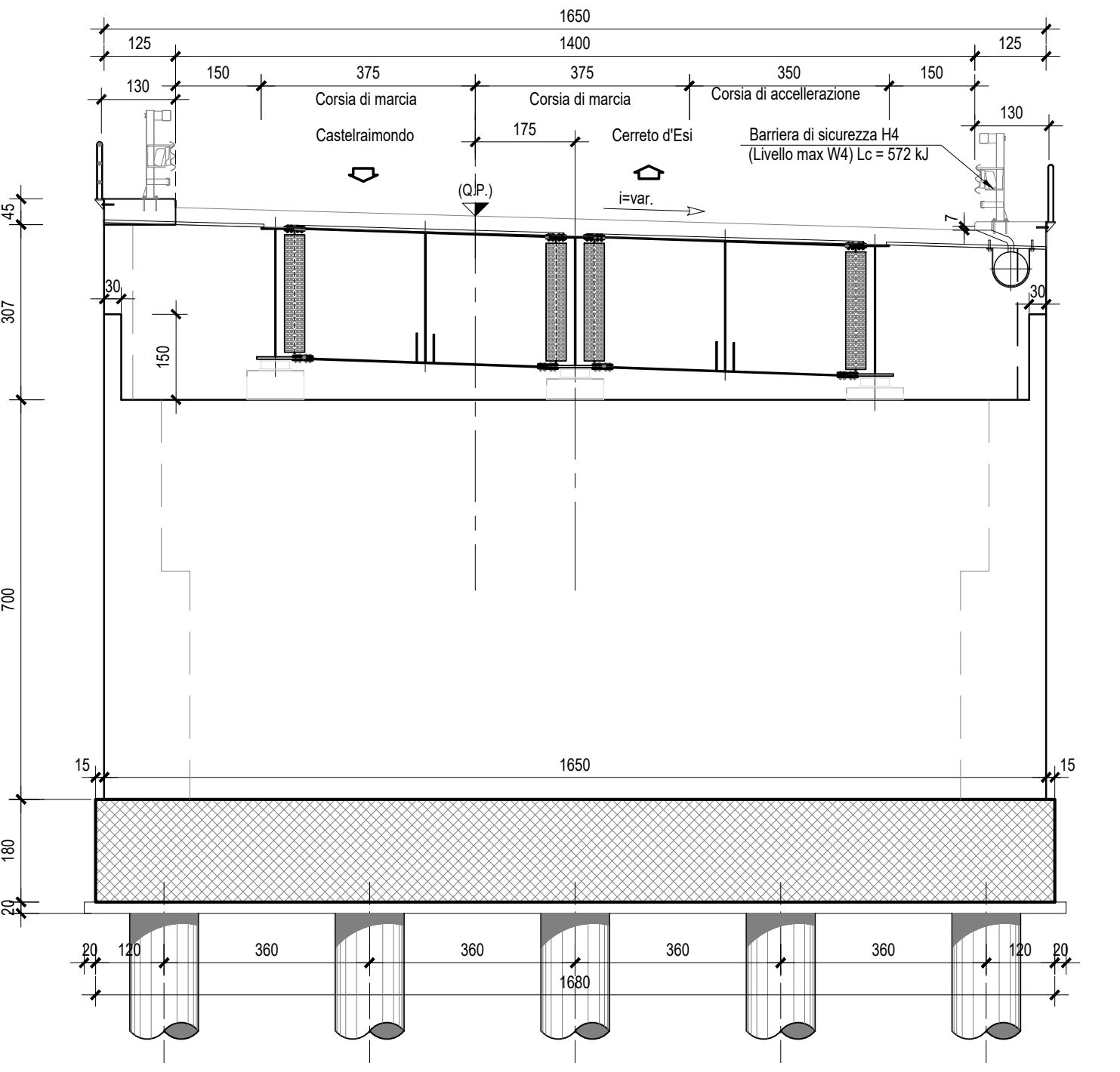
SEZIONE TRASVERSALE-Scala 1:200 (IN CORRISPONDENZA DELLA SPALLA)
