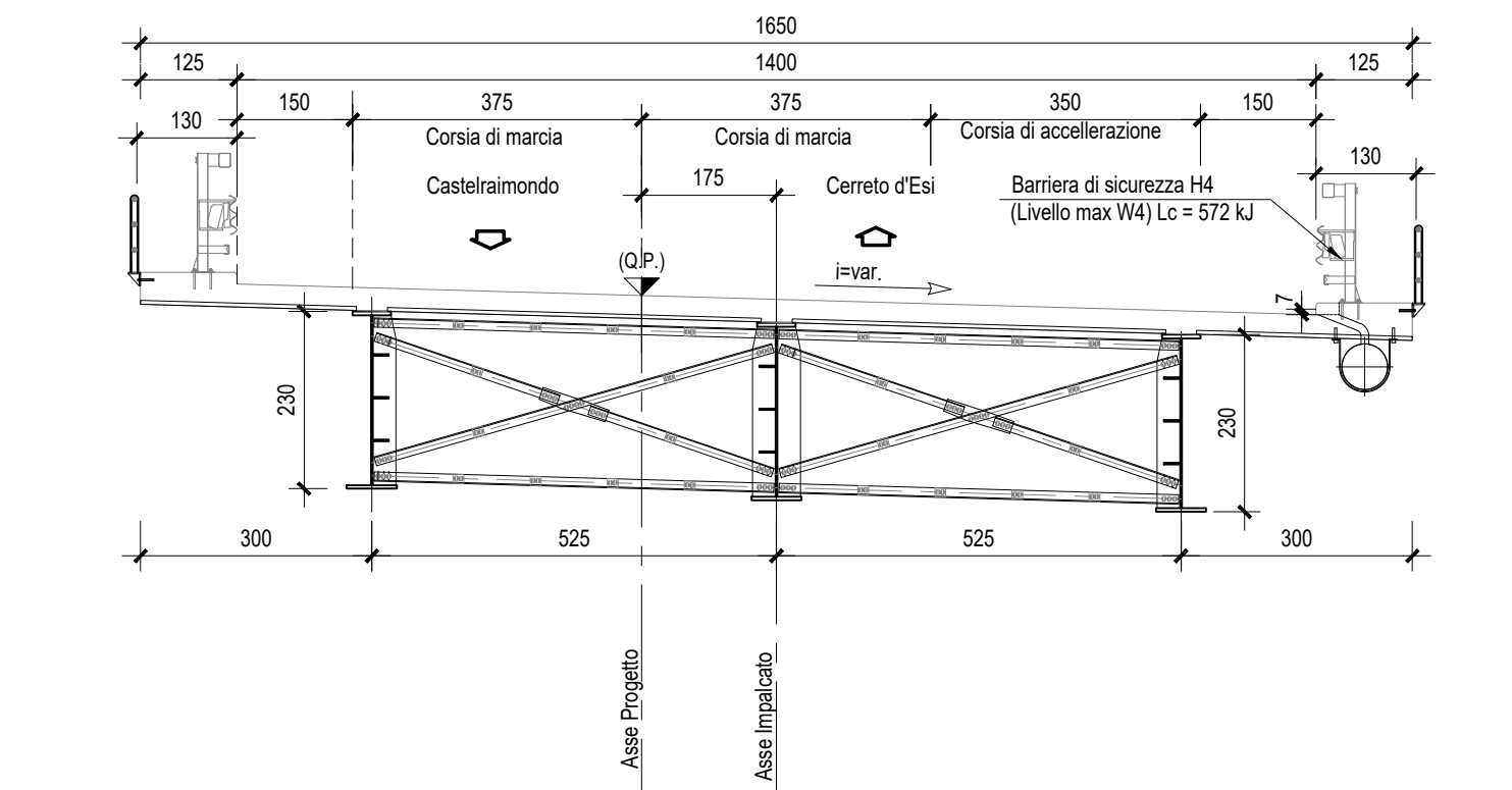
SEZIONE TRASVERSALE-Scala 1:200 (IN ASSE IMPALCATO)
