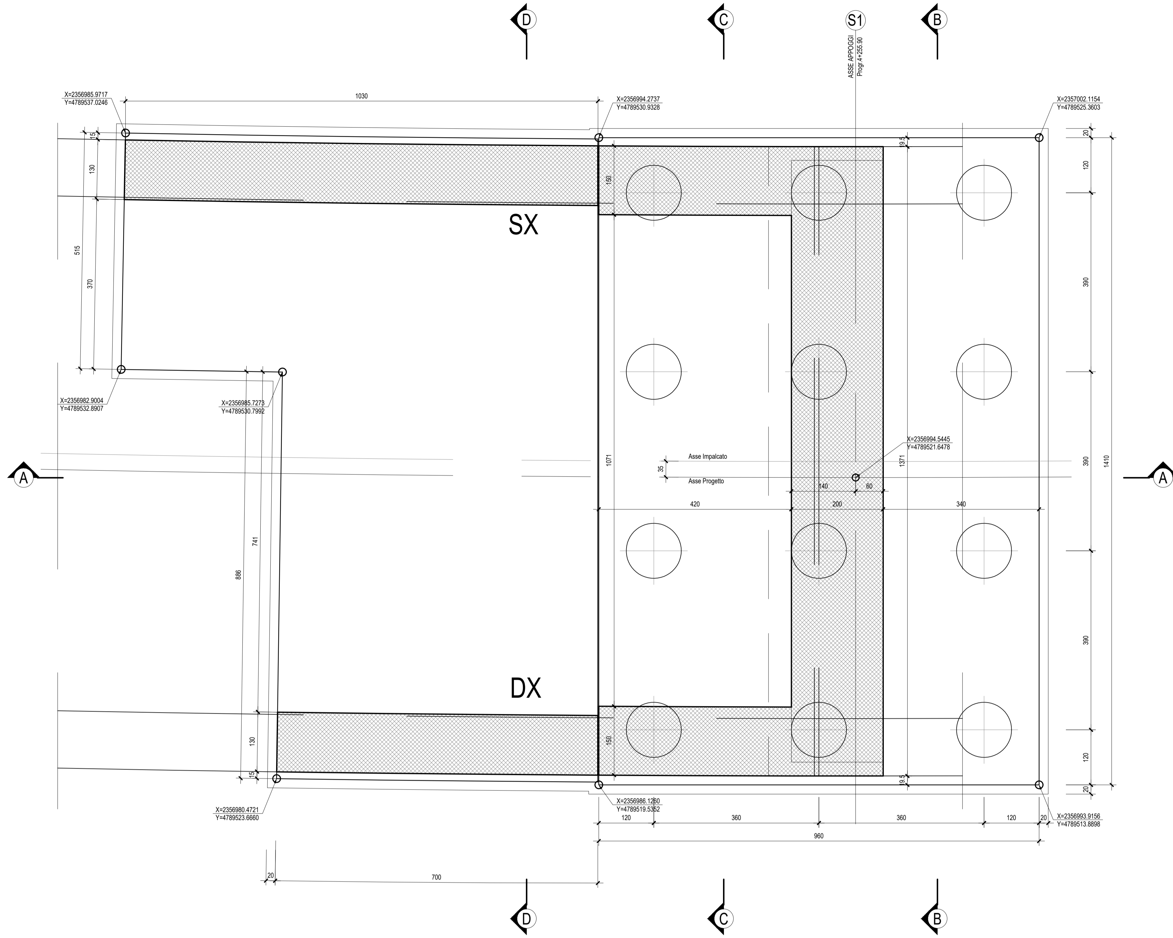
PIANTA FONDAZIONI-Scala 1:50
