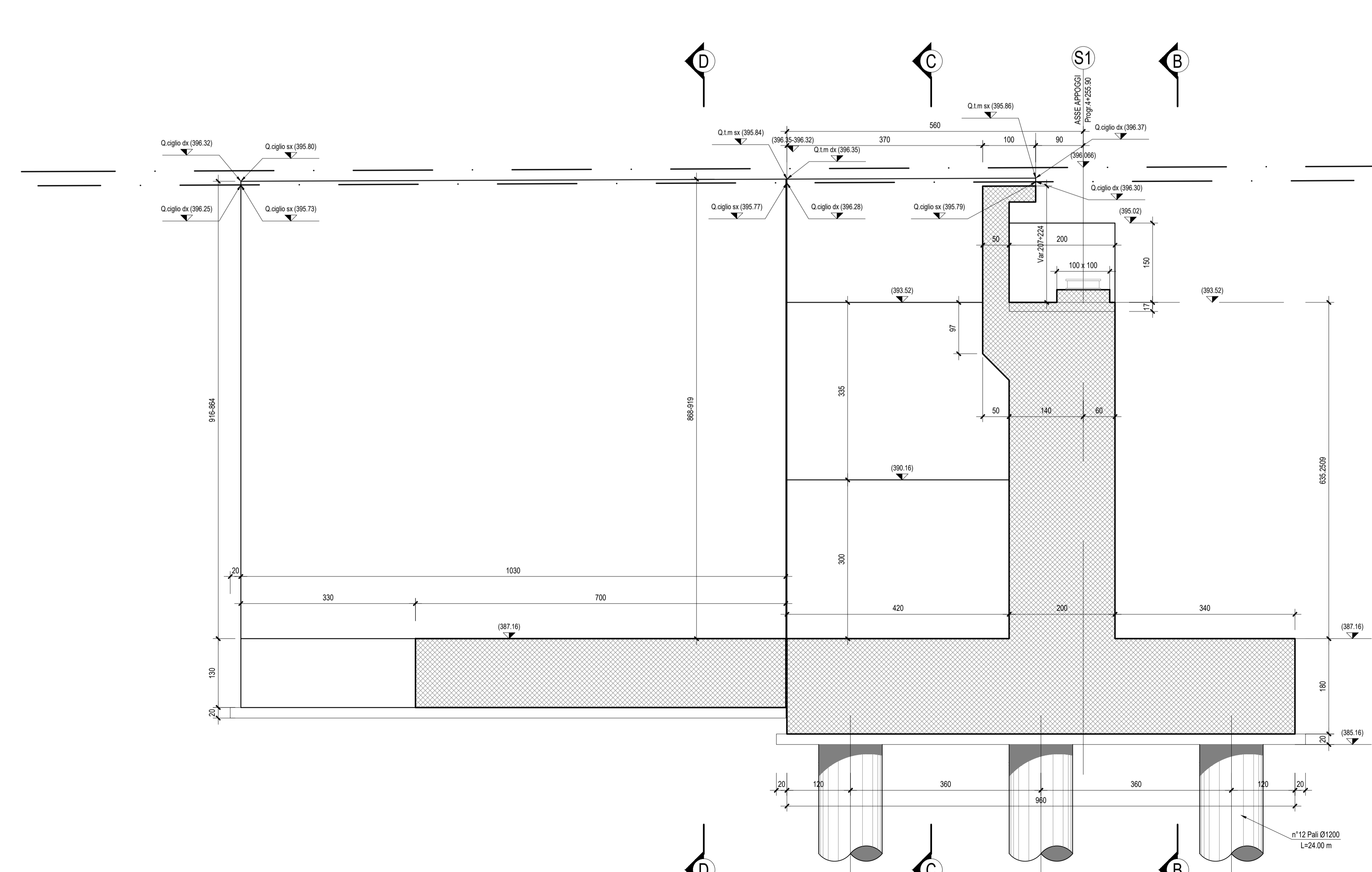
SEZIONE A-A-Scala 1:50
