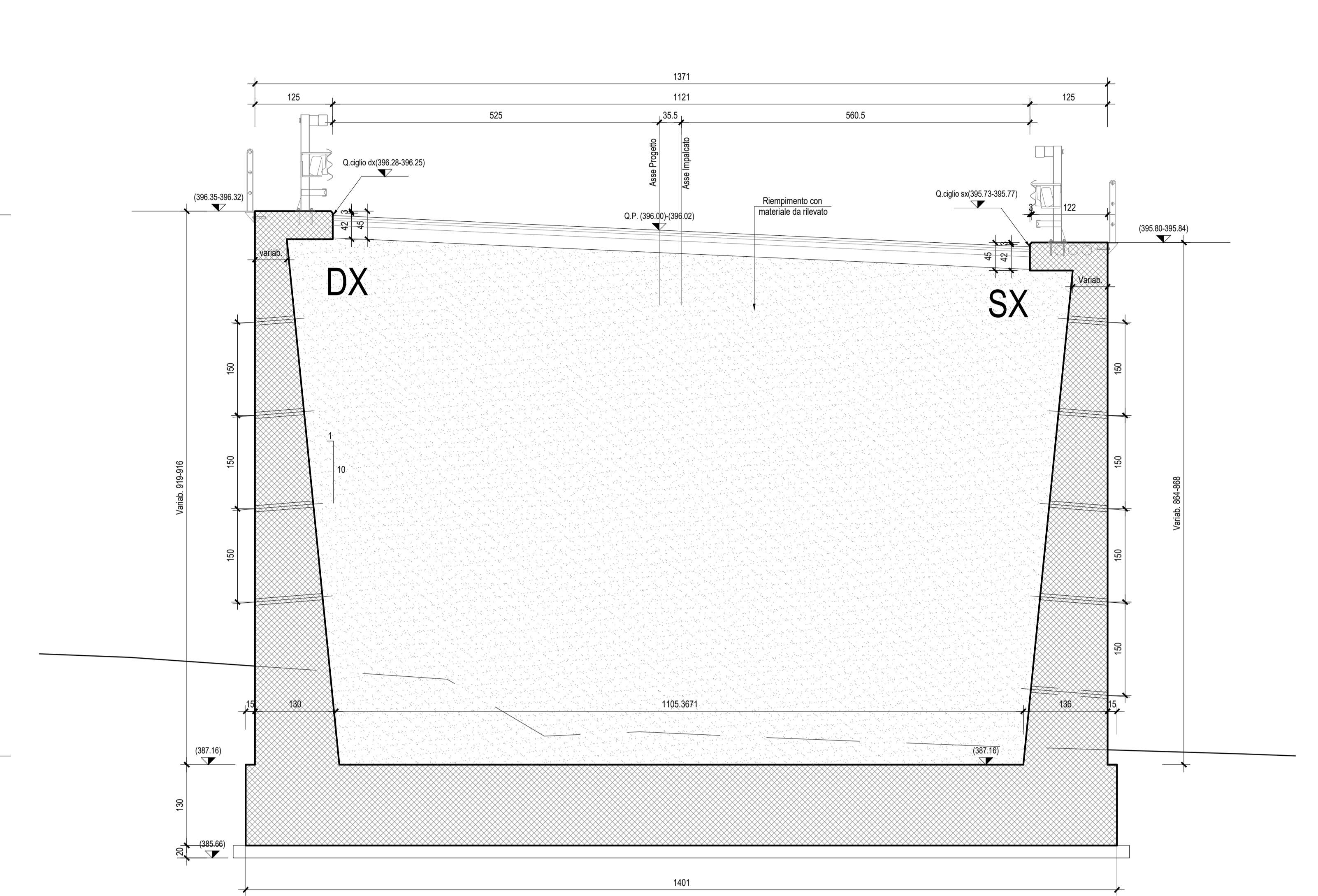
SEZIONE C-C-Scala 1:50
