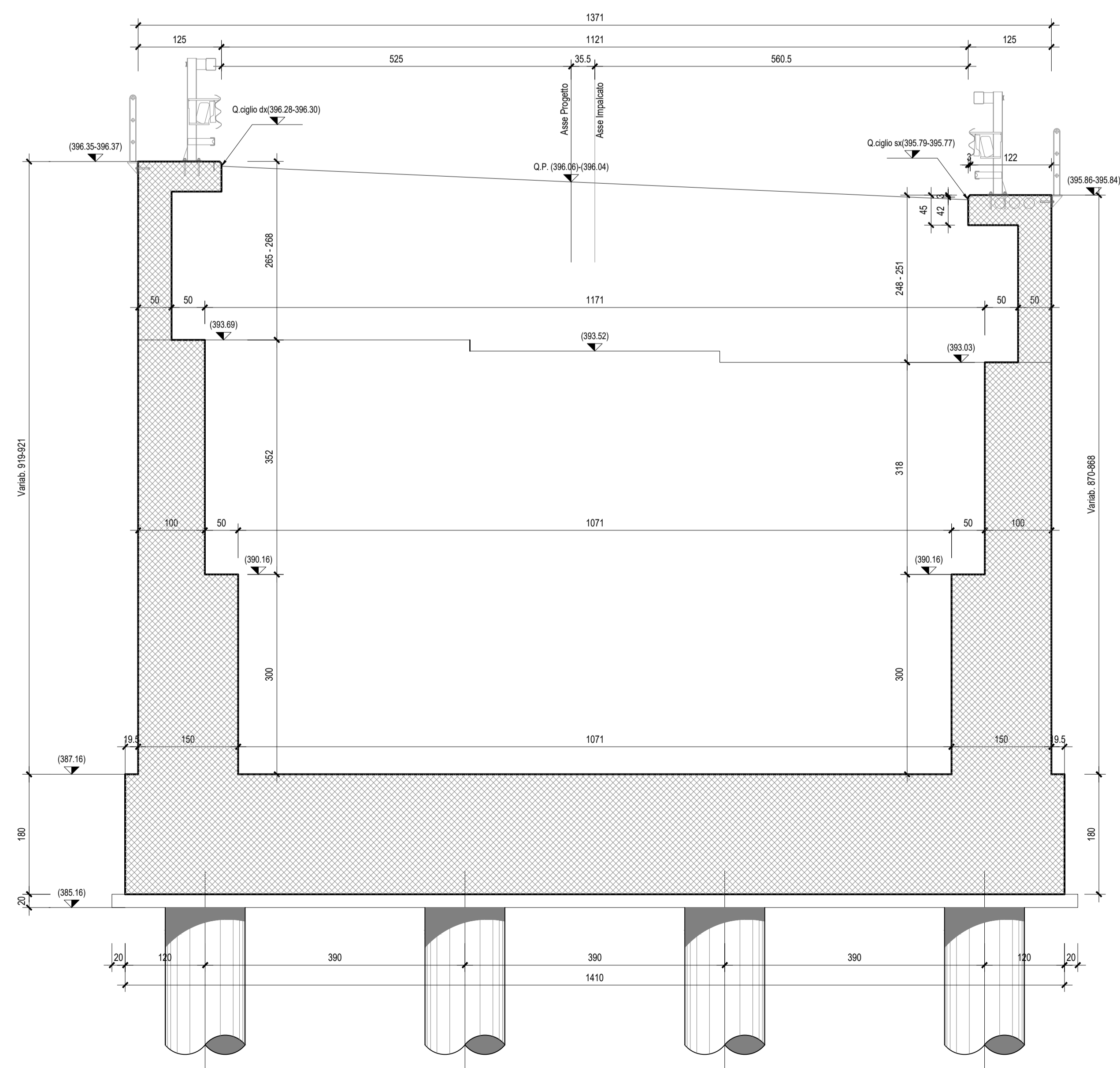
SEZIONE C-C-Scala 1:50
