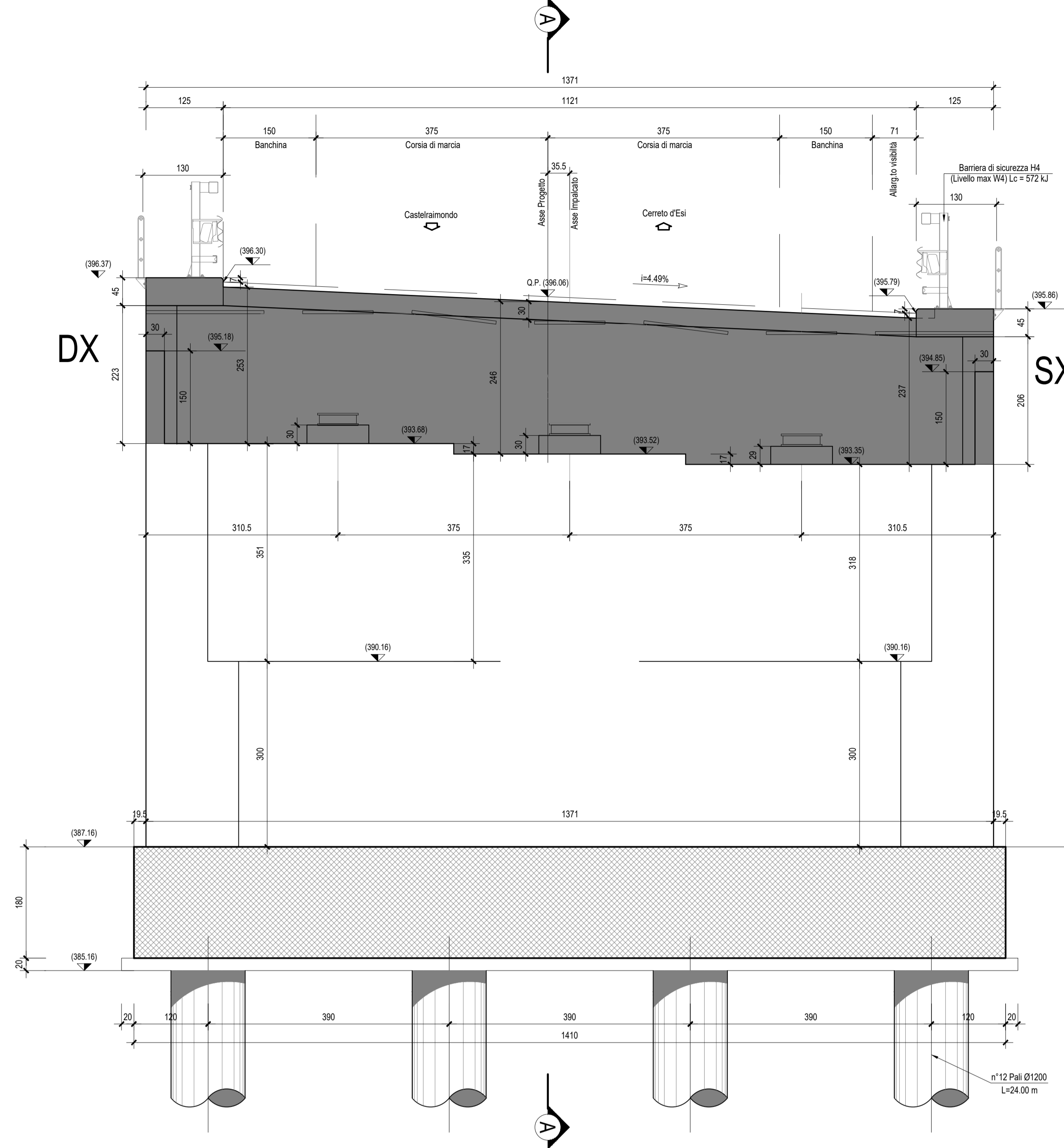
SEZIONE B-B-Scala 1:50
