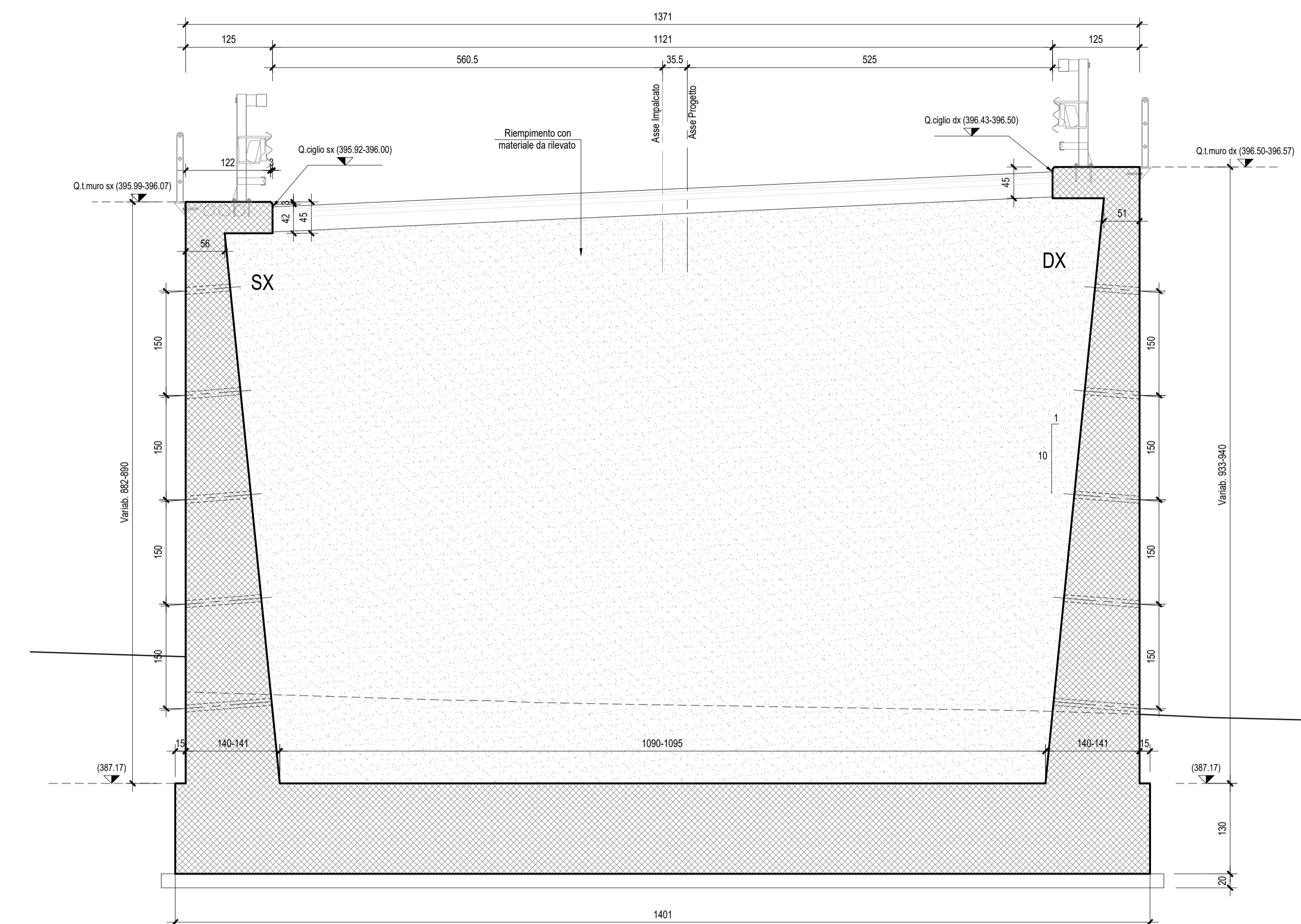
SEZIONE C-C-Scala 1:50
