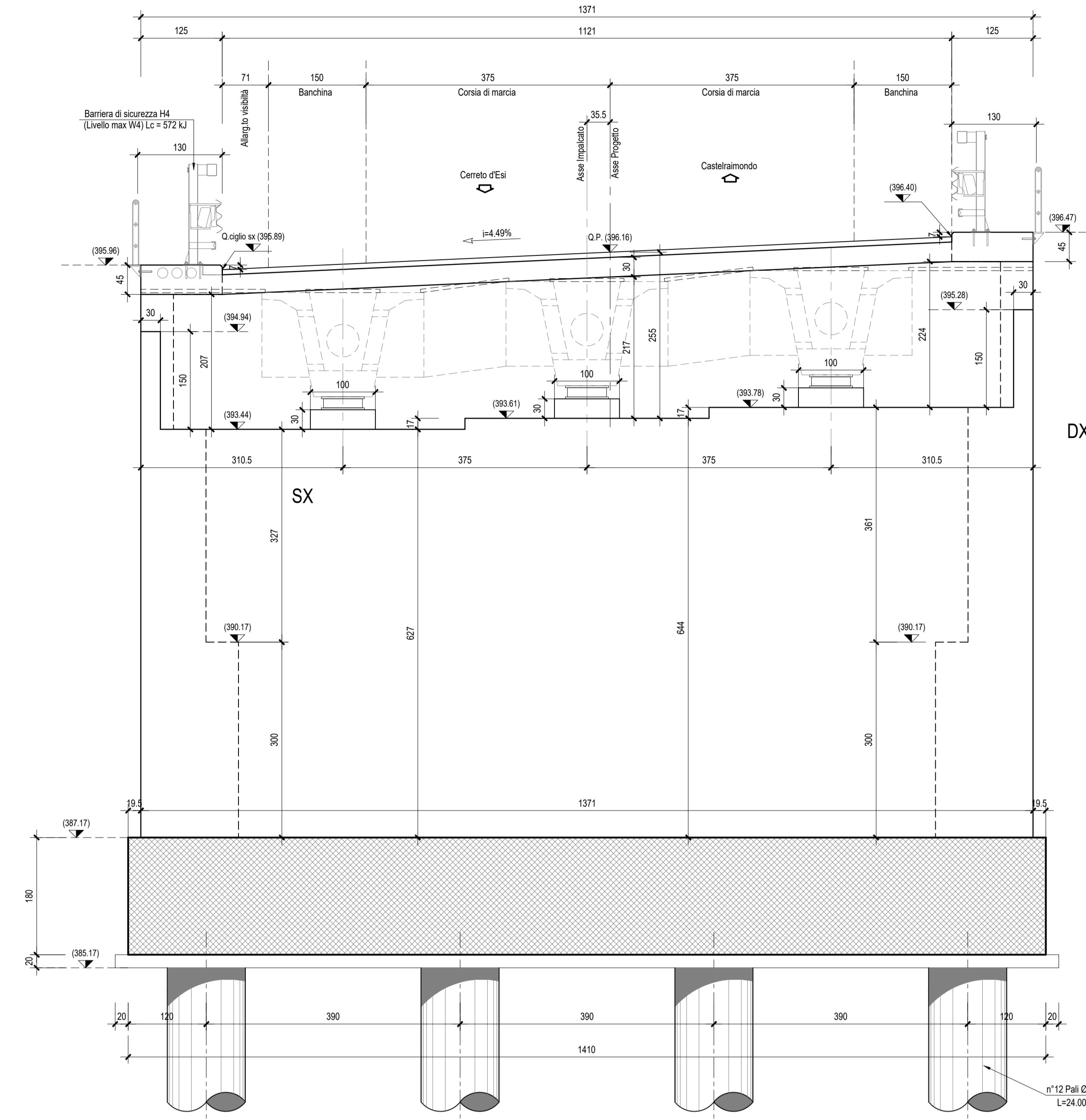
SEZIONE B-B-Scala 1:50
