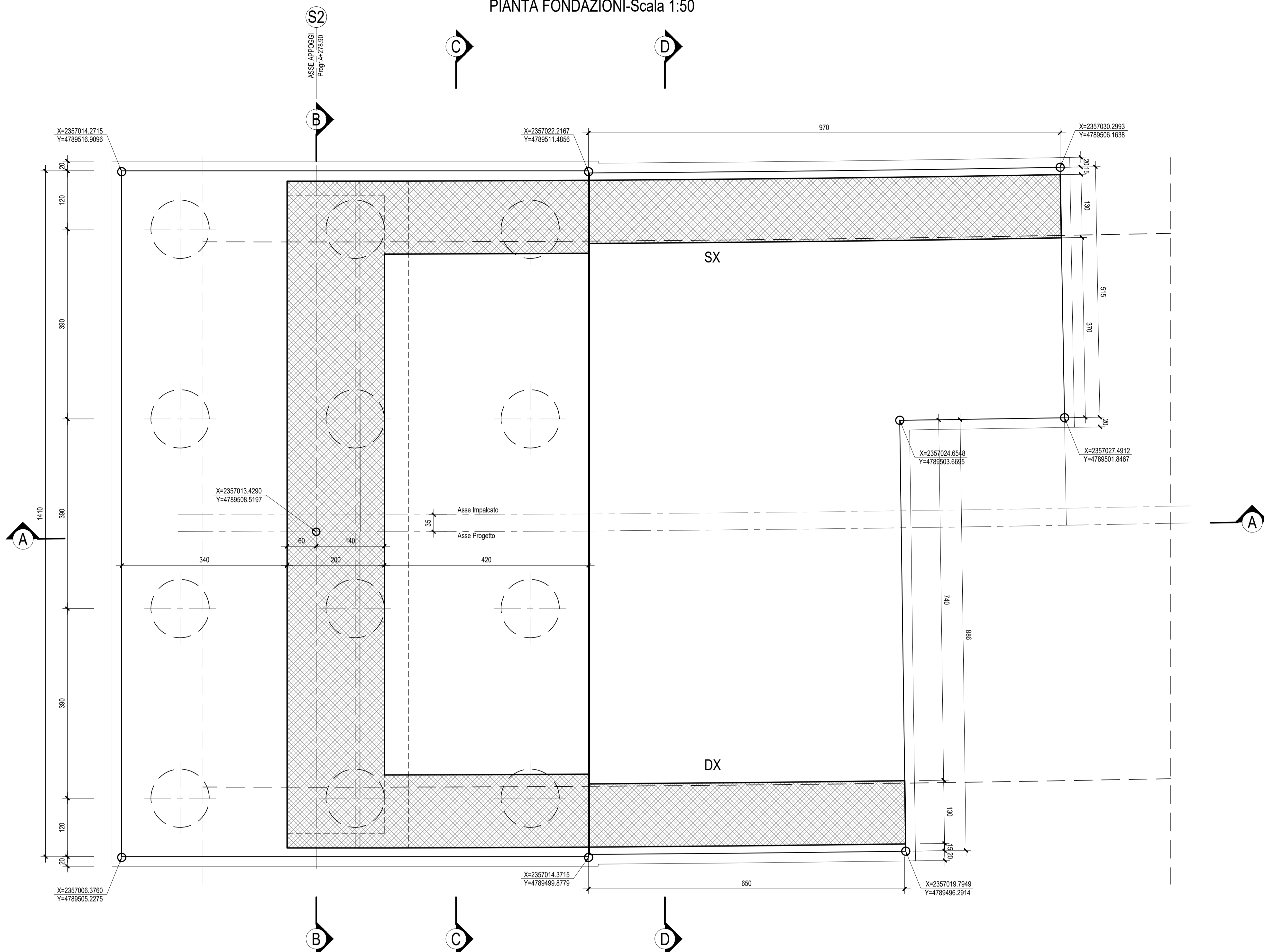
PIANTA FONDAZIONI-Scala 1:50
