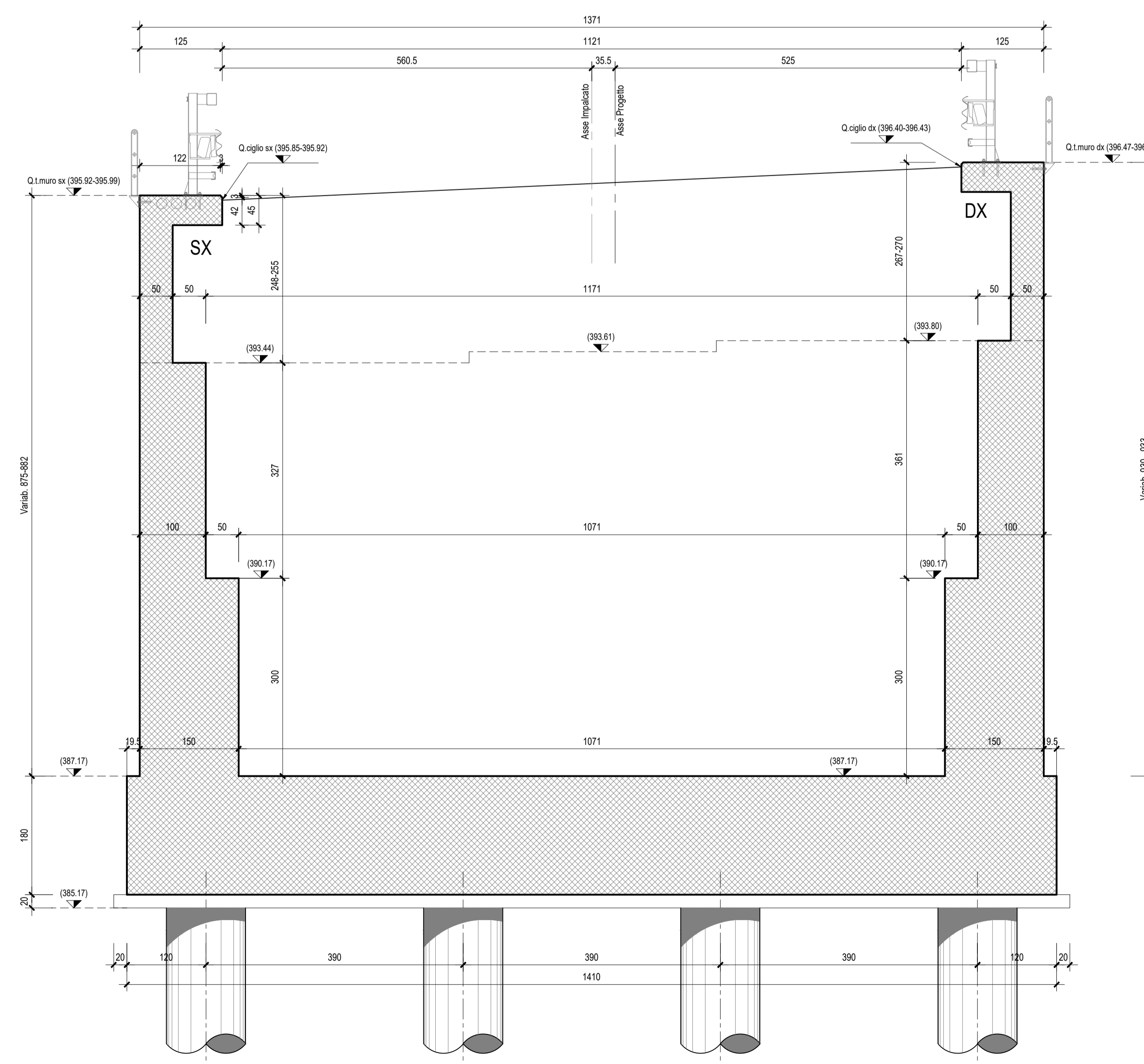
SEZIONE C-C-Scala 1:50
