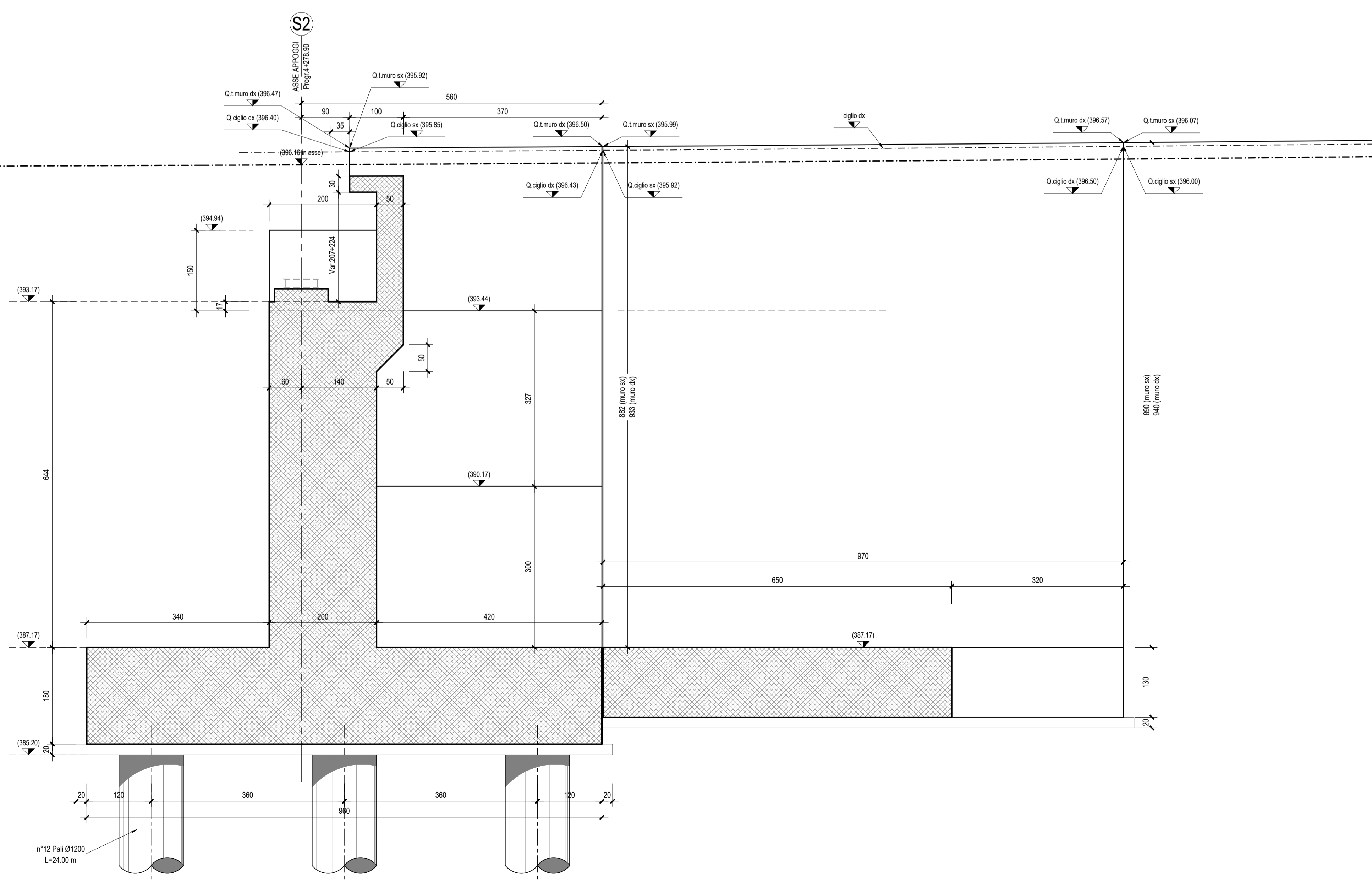
SEZIONE A-A-Scala 1:50
