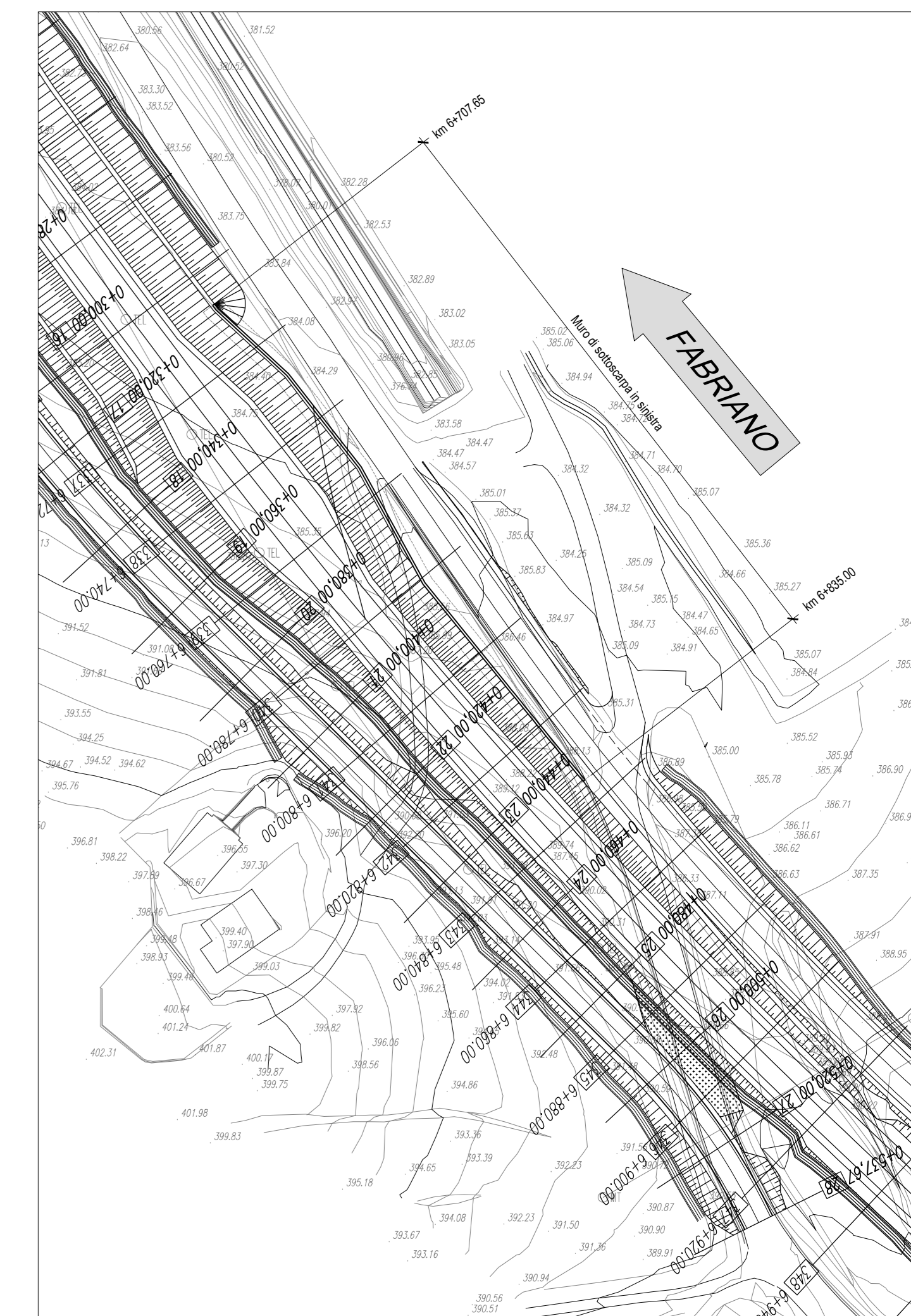
STRALCIO PLANIMETRICO -Scala 1:1000-
