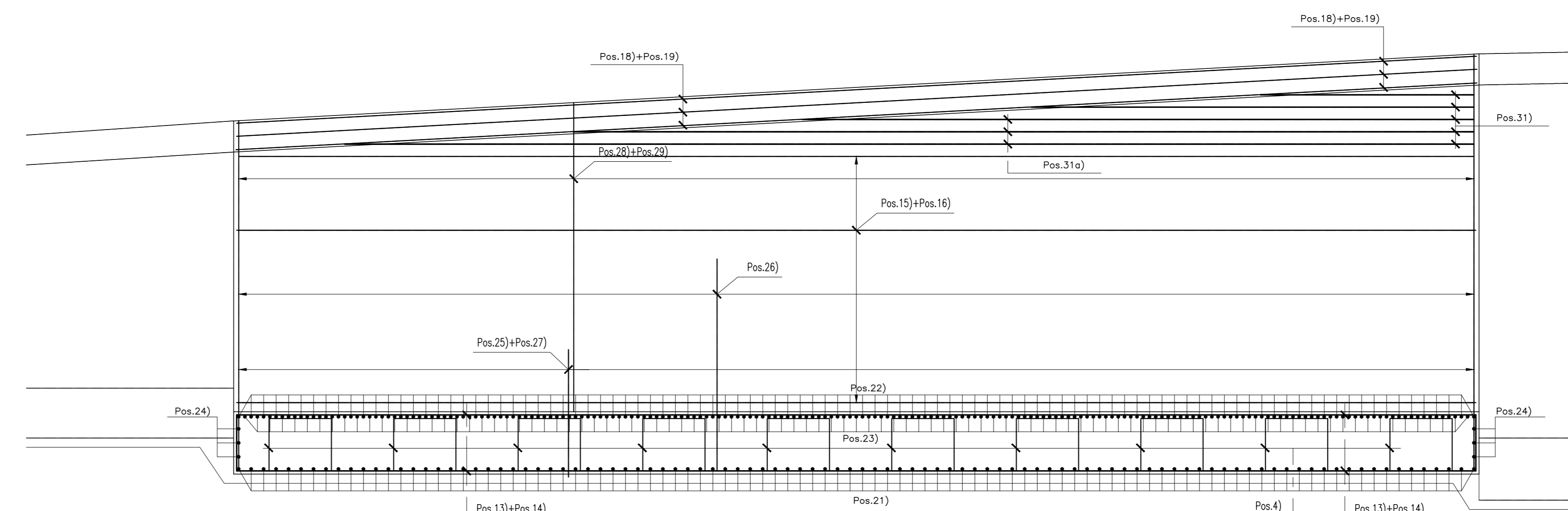
SEZIONE A-A: CONCIO 2 Scala 1:50
