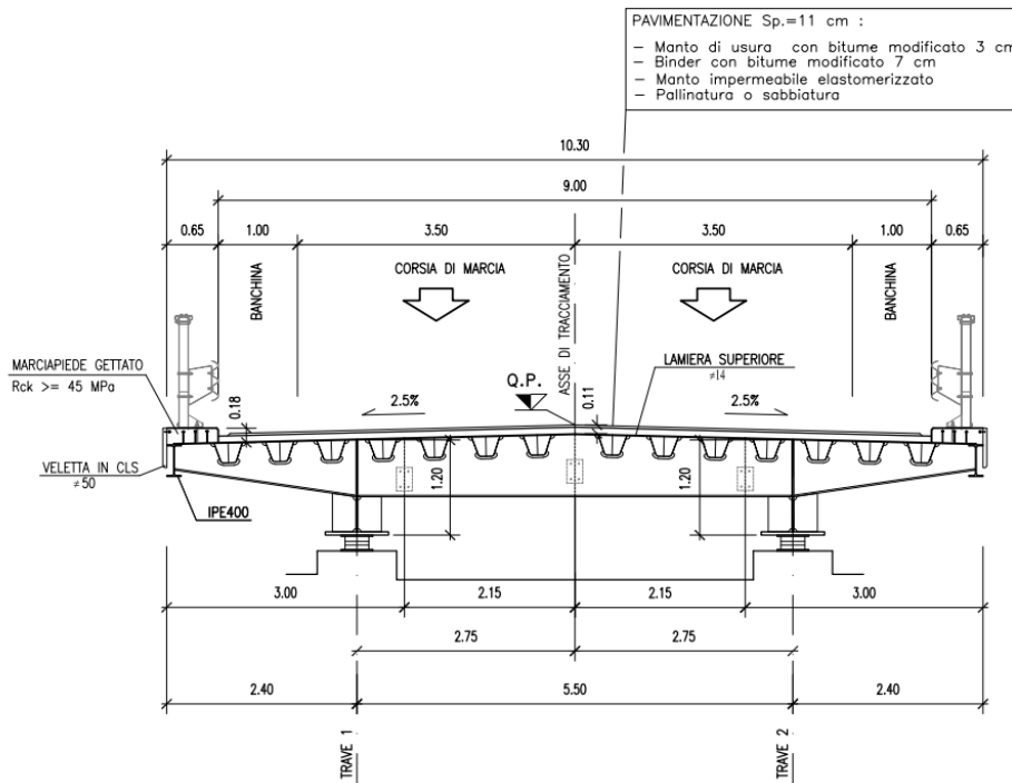
Figura 1: Sezione trasversale impalcato
