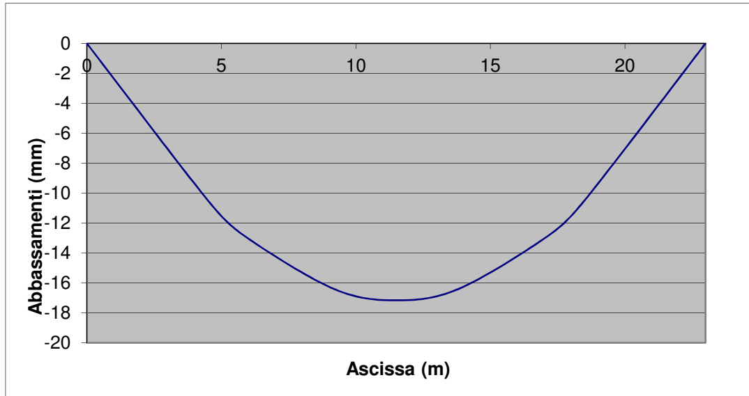
Fig. 7.1 – Abbassamenti verticali per il peso proprio della struttura e le opere di finitura
