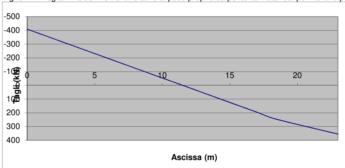
Fig. 6.2 – Diagramma dei tagli relativo al peso proprio carpenteria metallica+permanti portati
