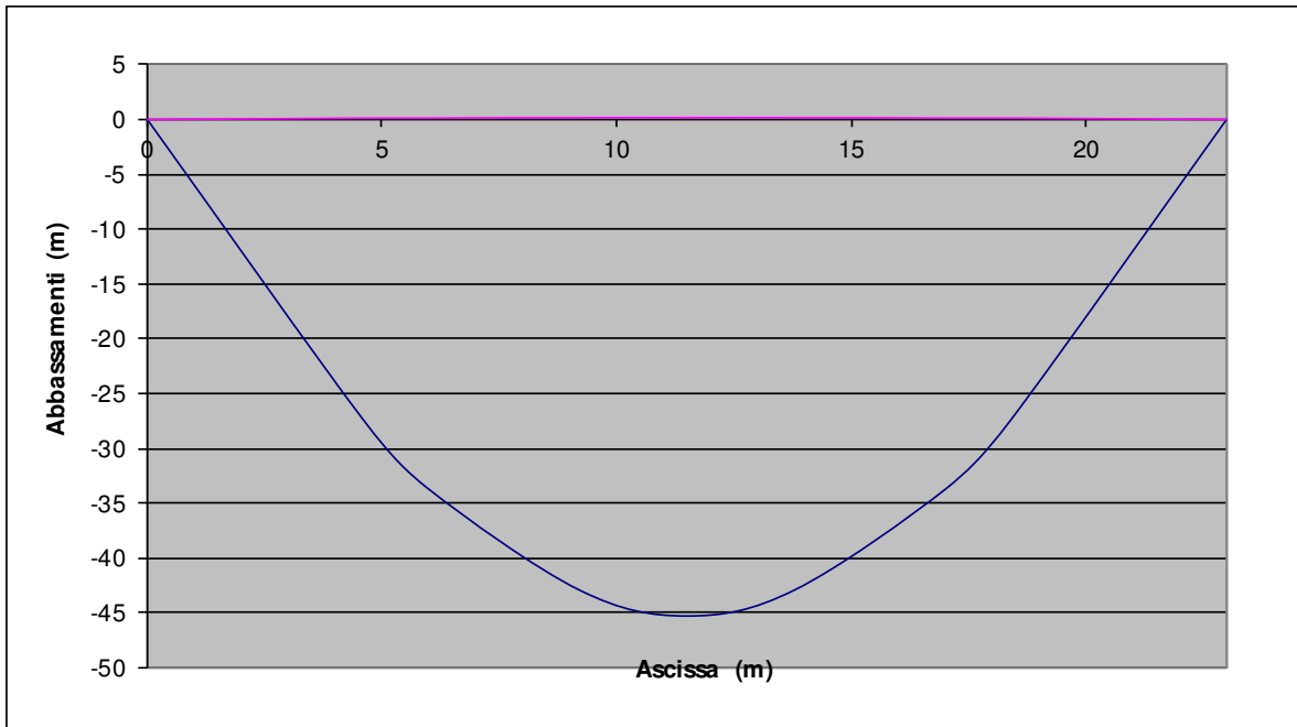
Fig. 14.2 – Abbassamenti verticali per i carichi verticali (fm)
