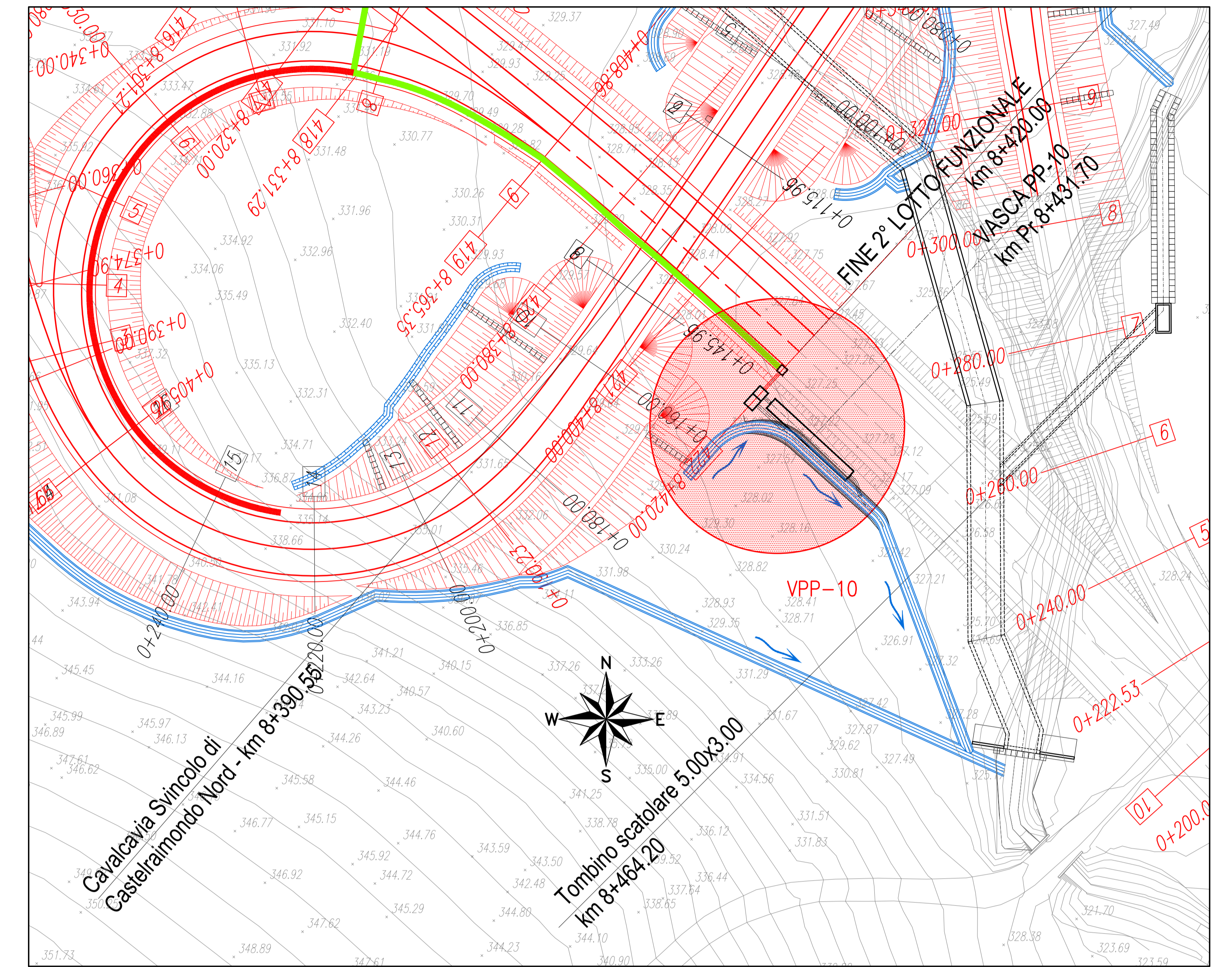
STRALCIO PLANIMETRICO SCALA 1:500
