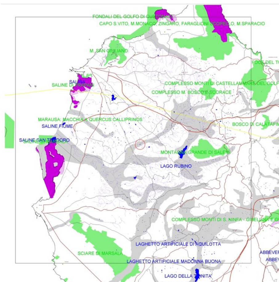
Figura 2-4: Ipotesi di rotte di migrazione lungo i fondo valle (tematismo in grigio) nell'area vasta del trapanese. (circoletto in rosso l'area IBA lghetto Bordino).
