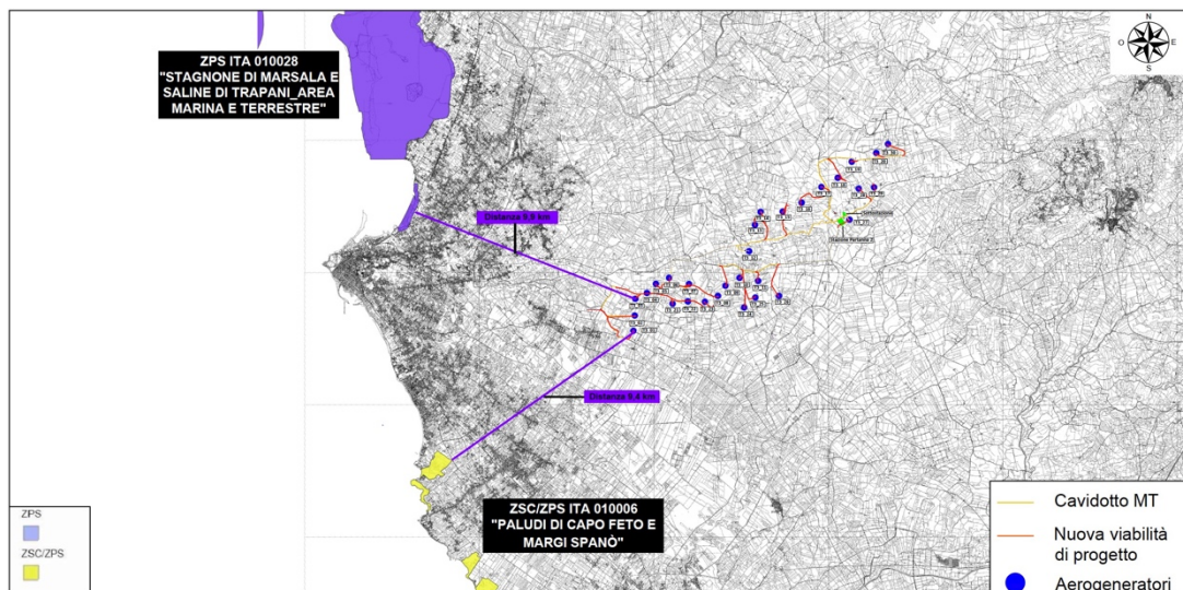
Figura 1-2: Distanze minime tra impianto e ZPS.
