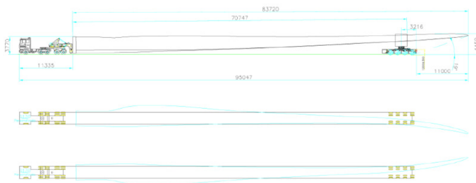
Figura 3-1: Semirimorchio speciale per trasporto pala
