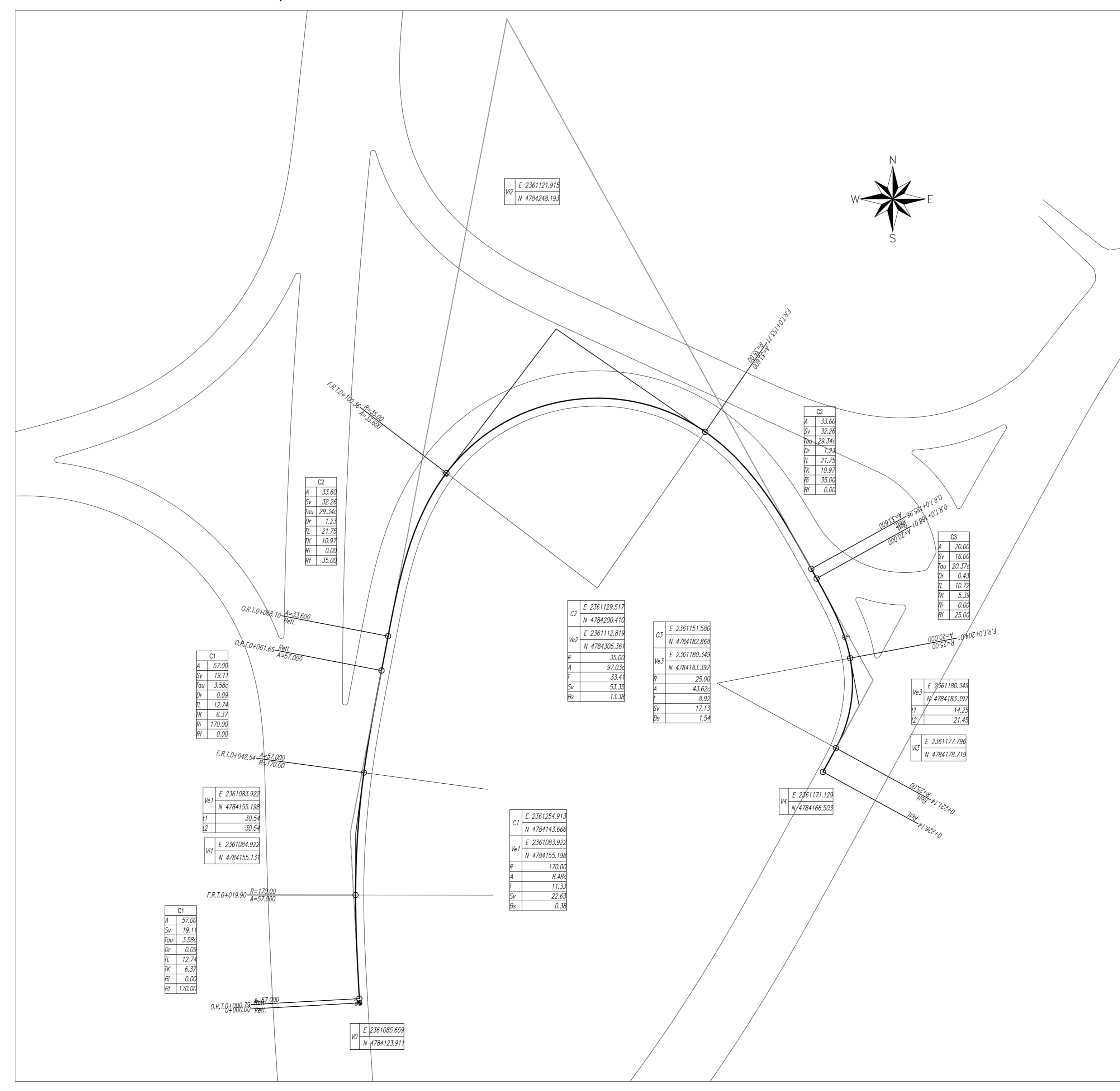
Planimetria di tracciamento rampa "A" - Scala - 1:500
