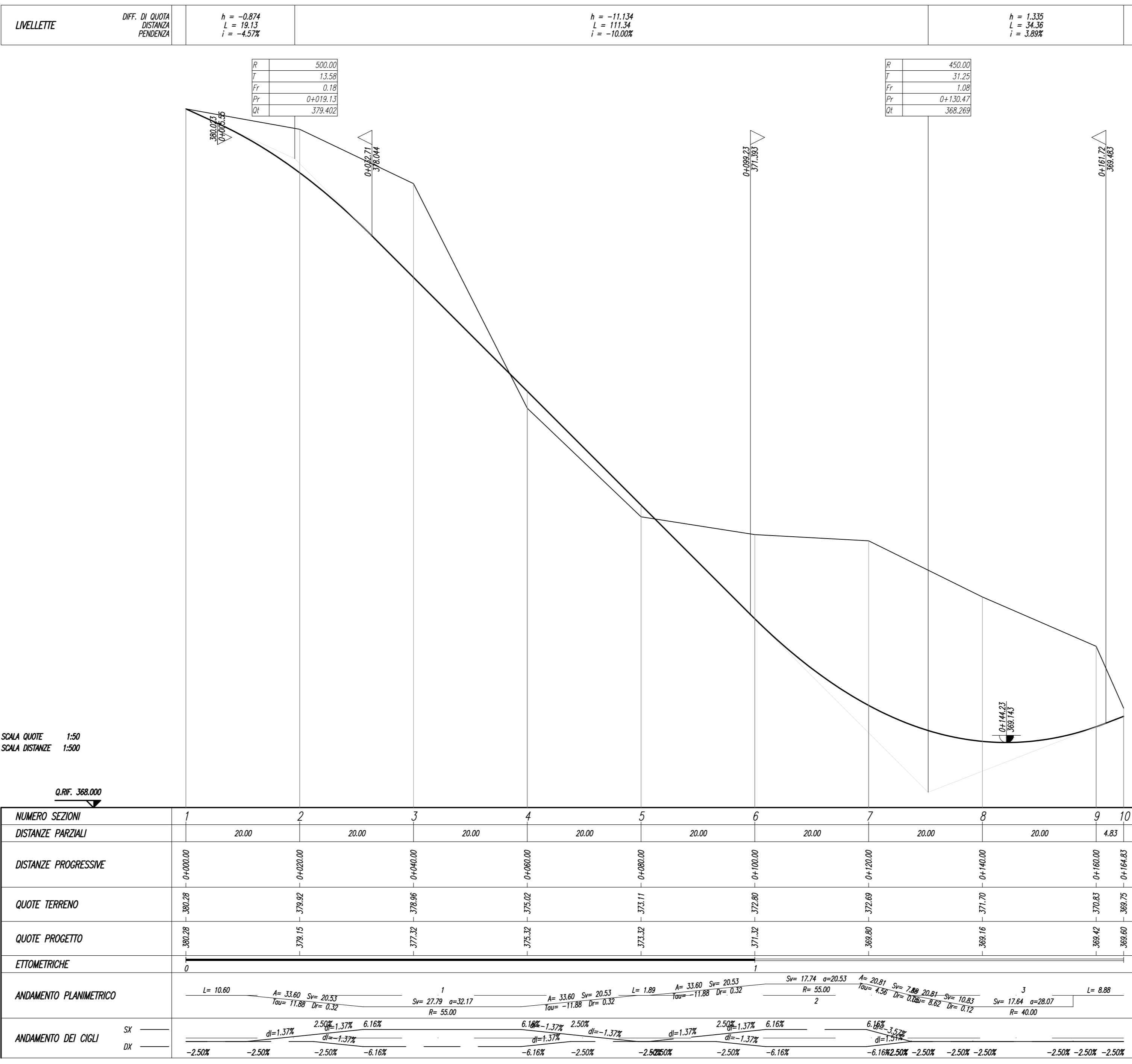
Profilo longitudinale viabilità Est - Scala - 1:500/50
