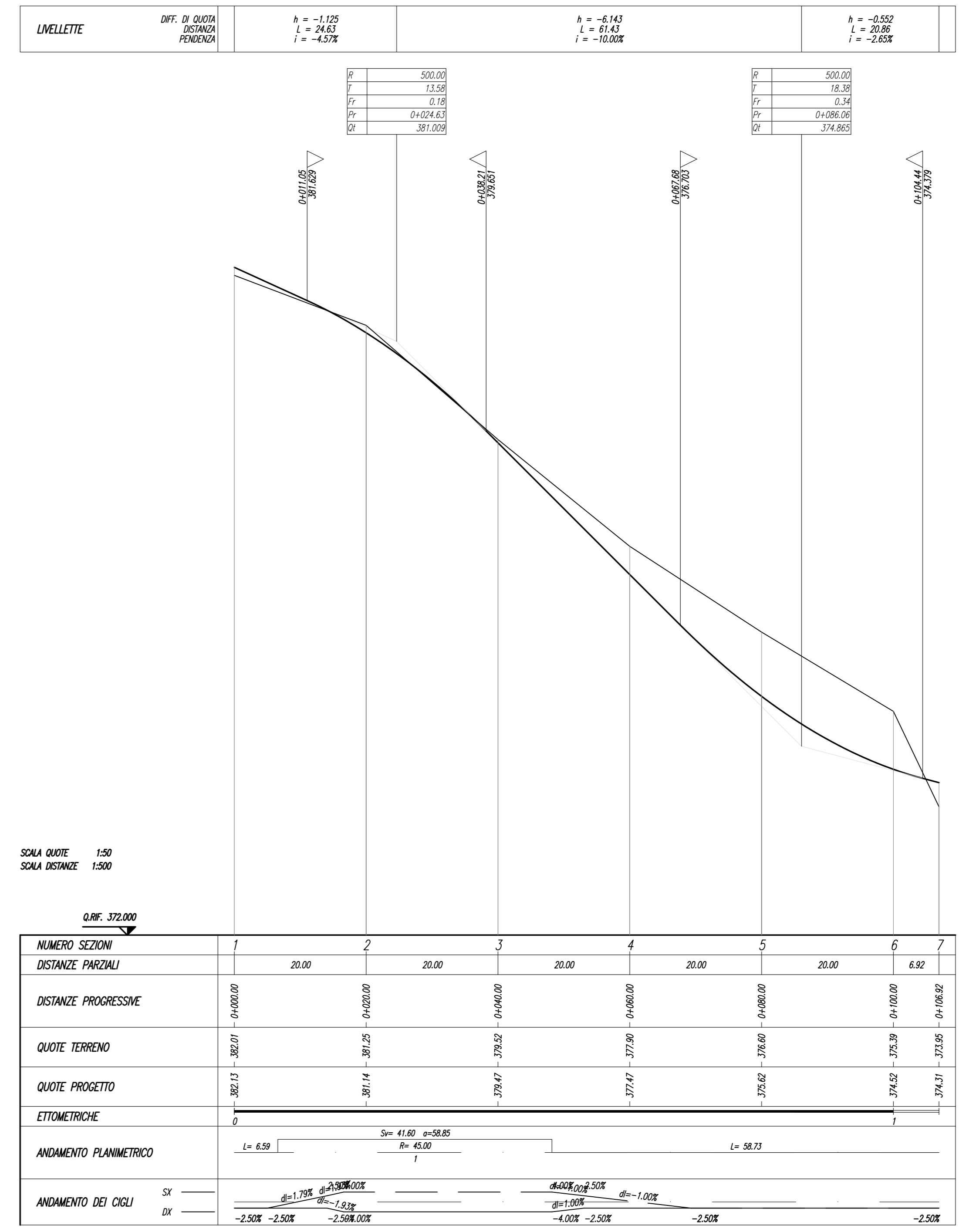
Profilo longitudinale viabilità Ovest - Scala - 1:500/50
