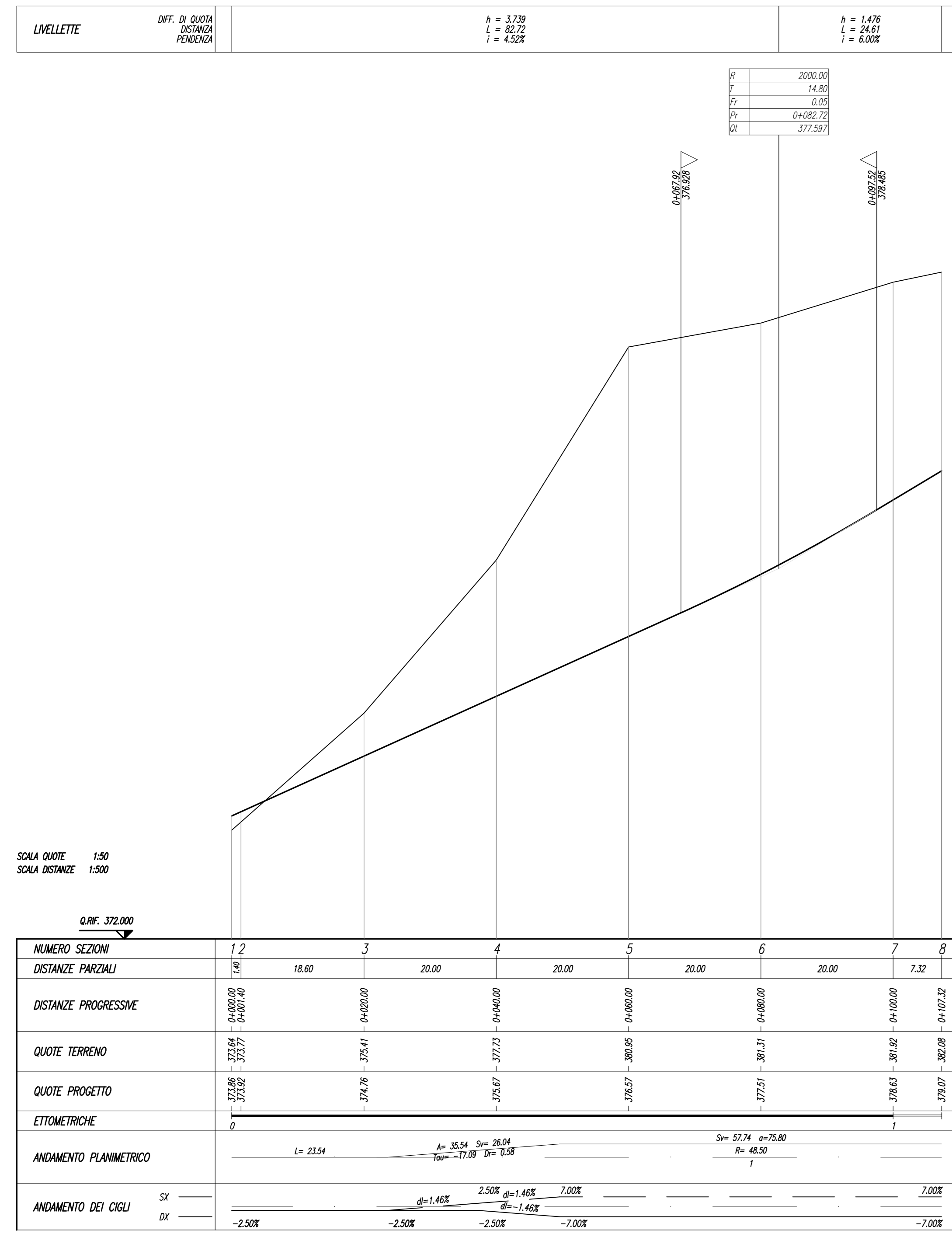
Profilo longitudinale rampa F - Scala - 1:500/50
