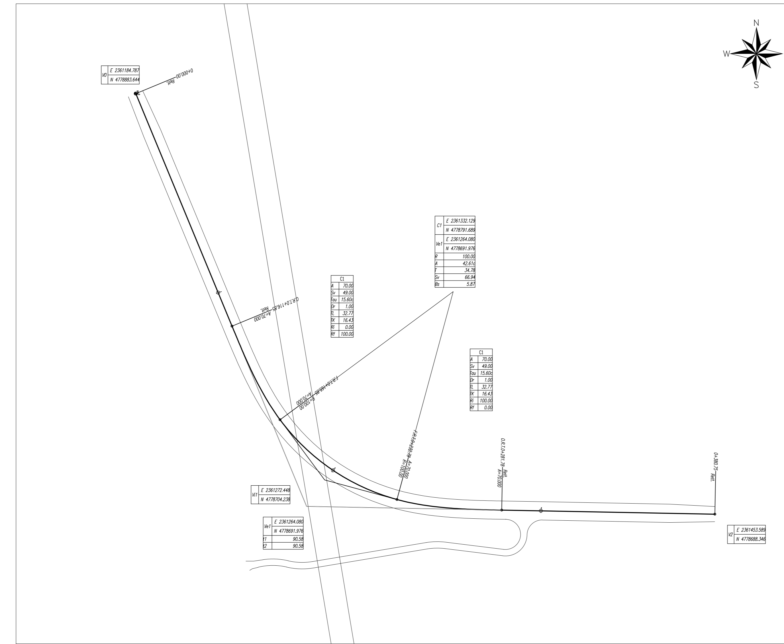
Planimetria di tracciamento strada località Pianello - Scala - 1:1000
