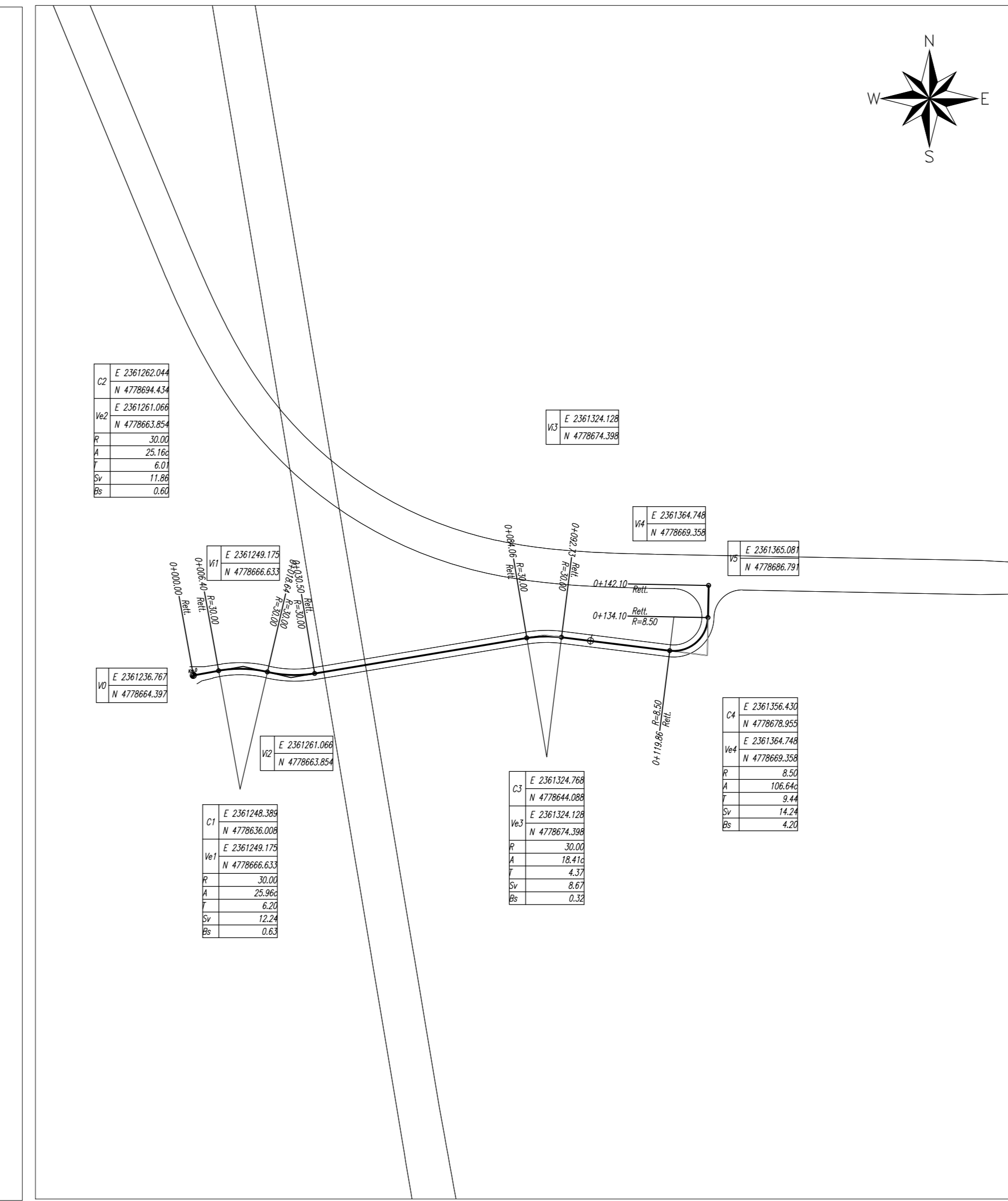
Planimetria di tracciamento strada di accesso al depuratore - Scala - 1:1000
