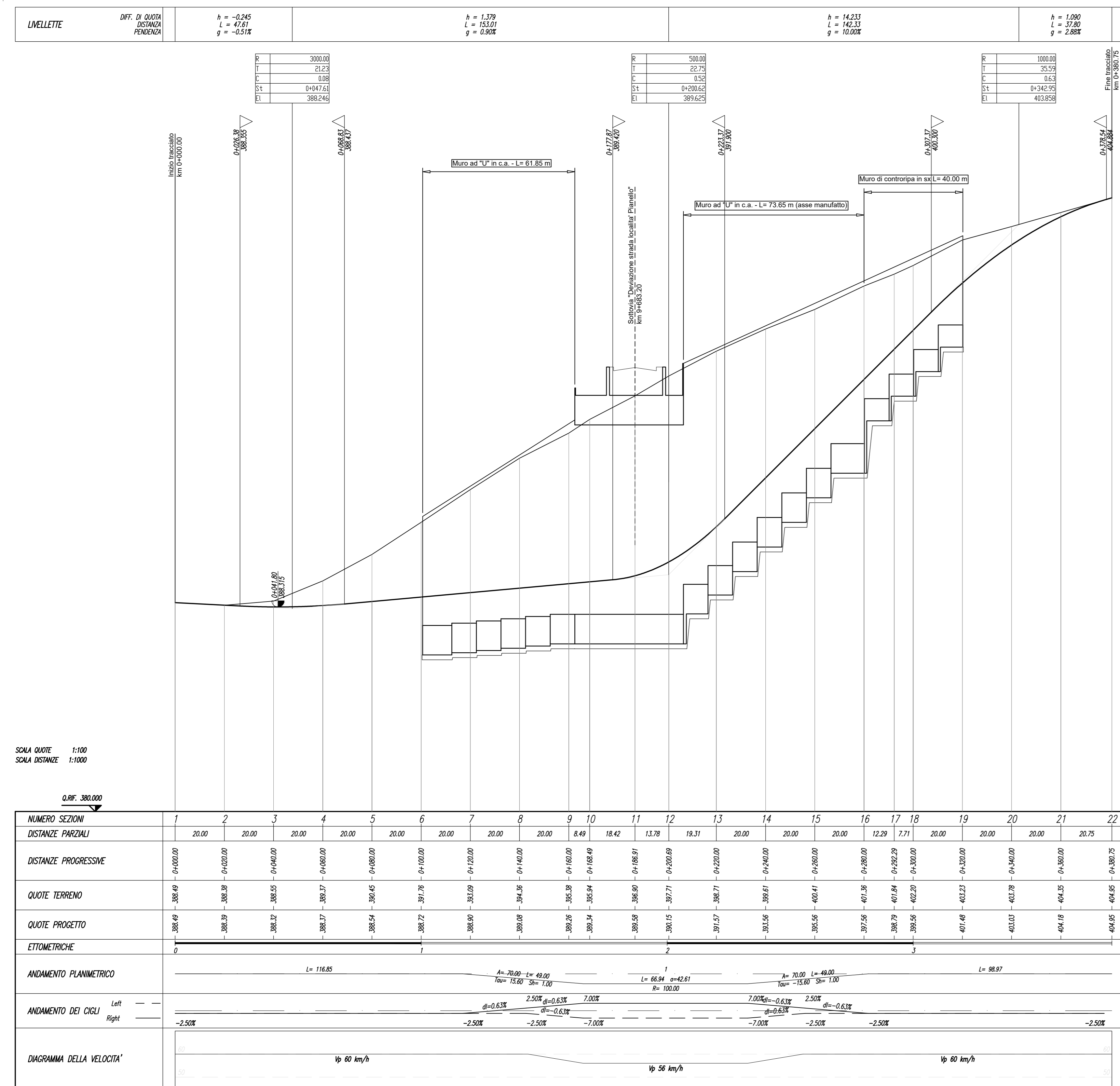
Profilo longitudinale strada strada località Pianello - Scala - 1:1000/100
