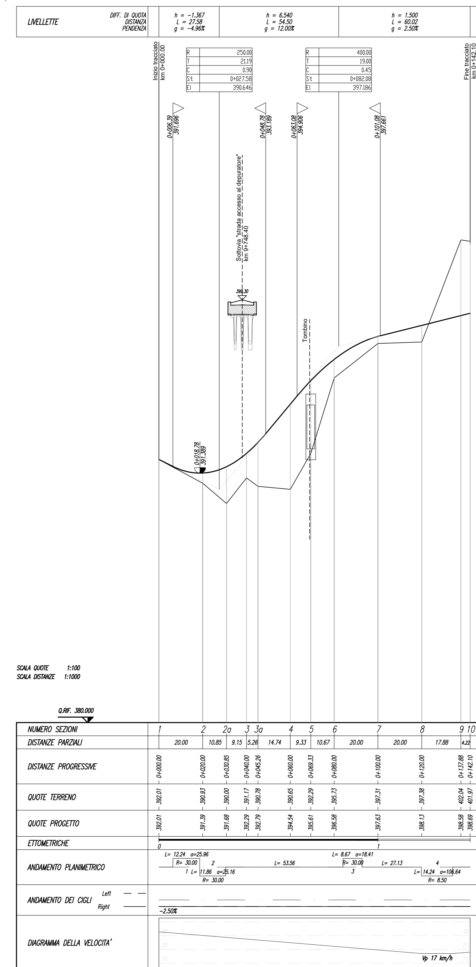
Profilo longitudinale strada di accesso al depuratore - Scala - 1:1000/100
