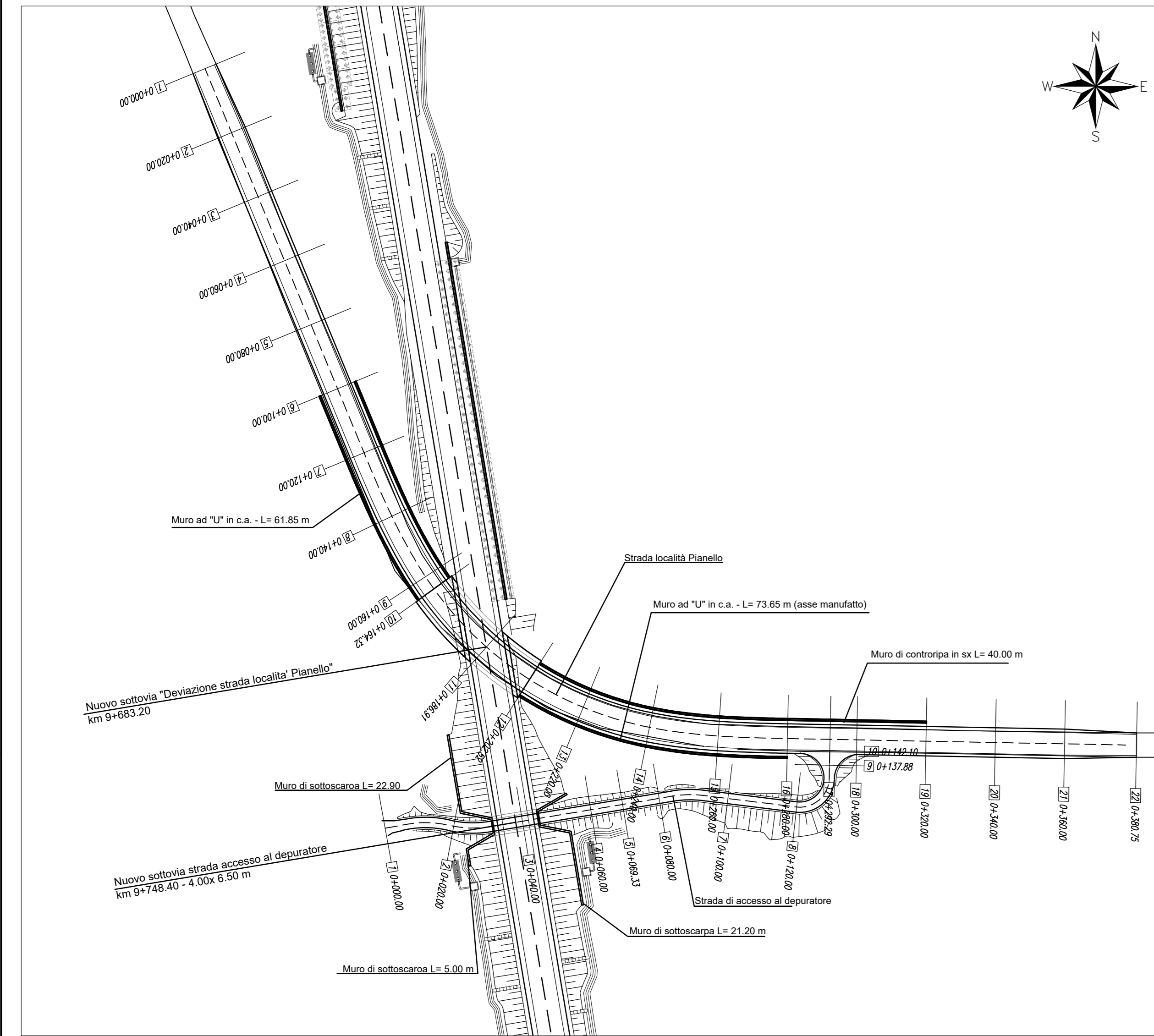
Planimetria di progetto - Scala - 1:1000
