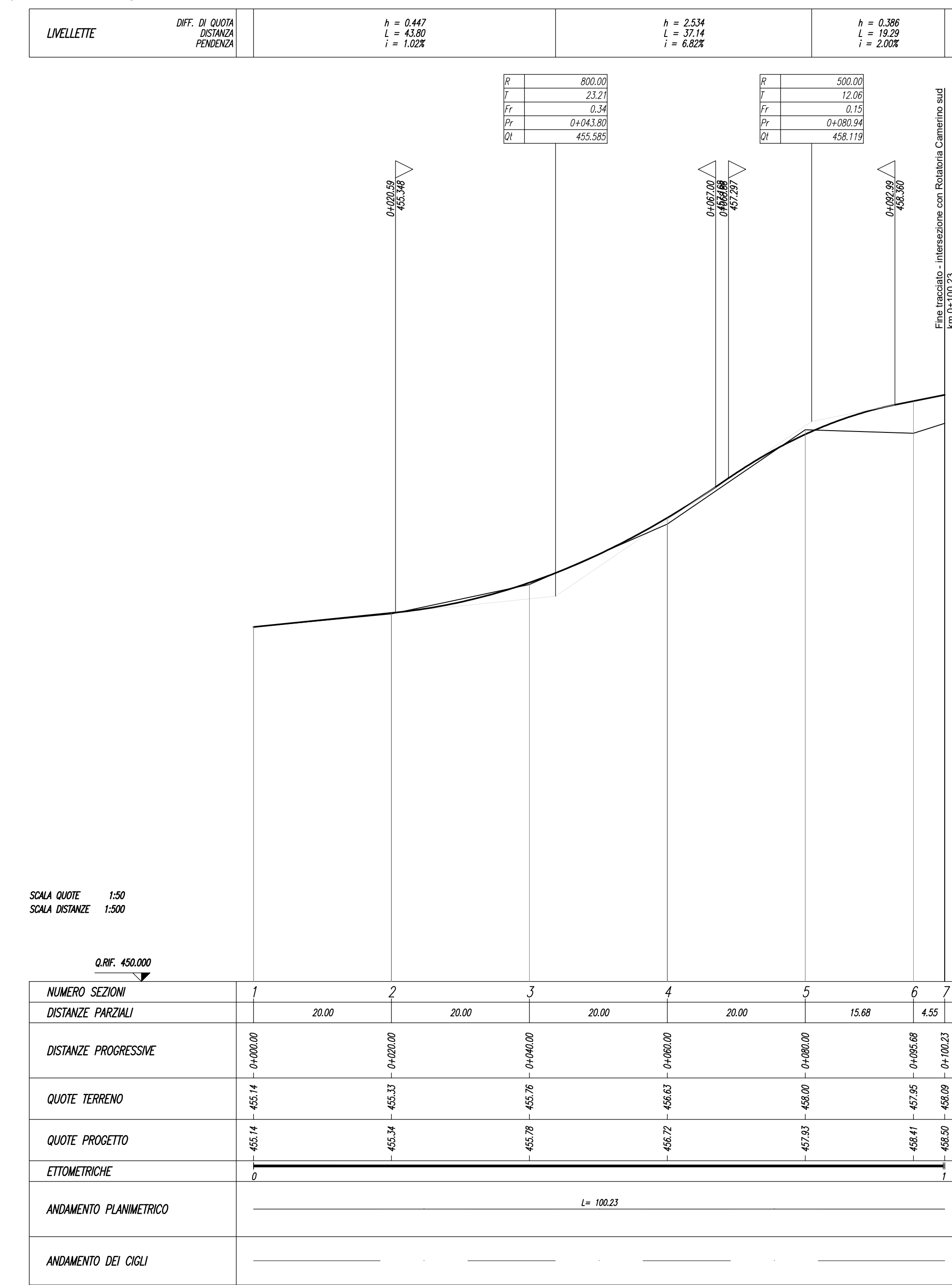
Profilo longitudinale Riabilitazione tratto S.P 256 - Scala - 1:1000/100
