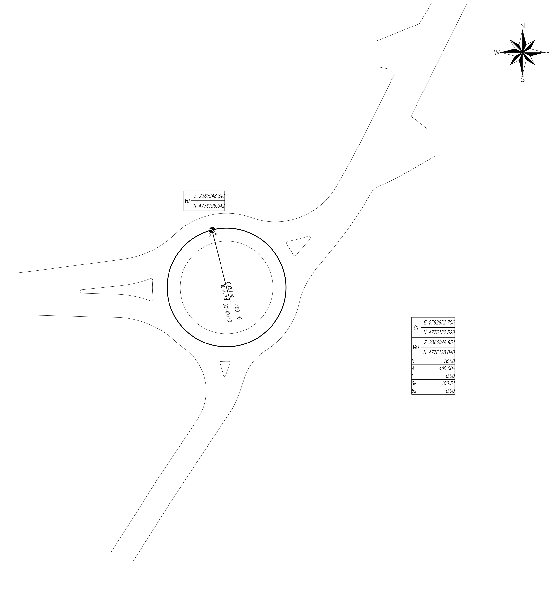
Planimetria di tracciamento Rotatoria Muccia - Scala - 1:500
