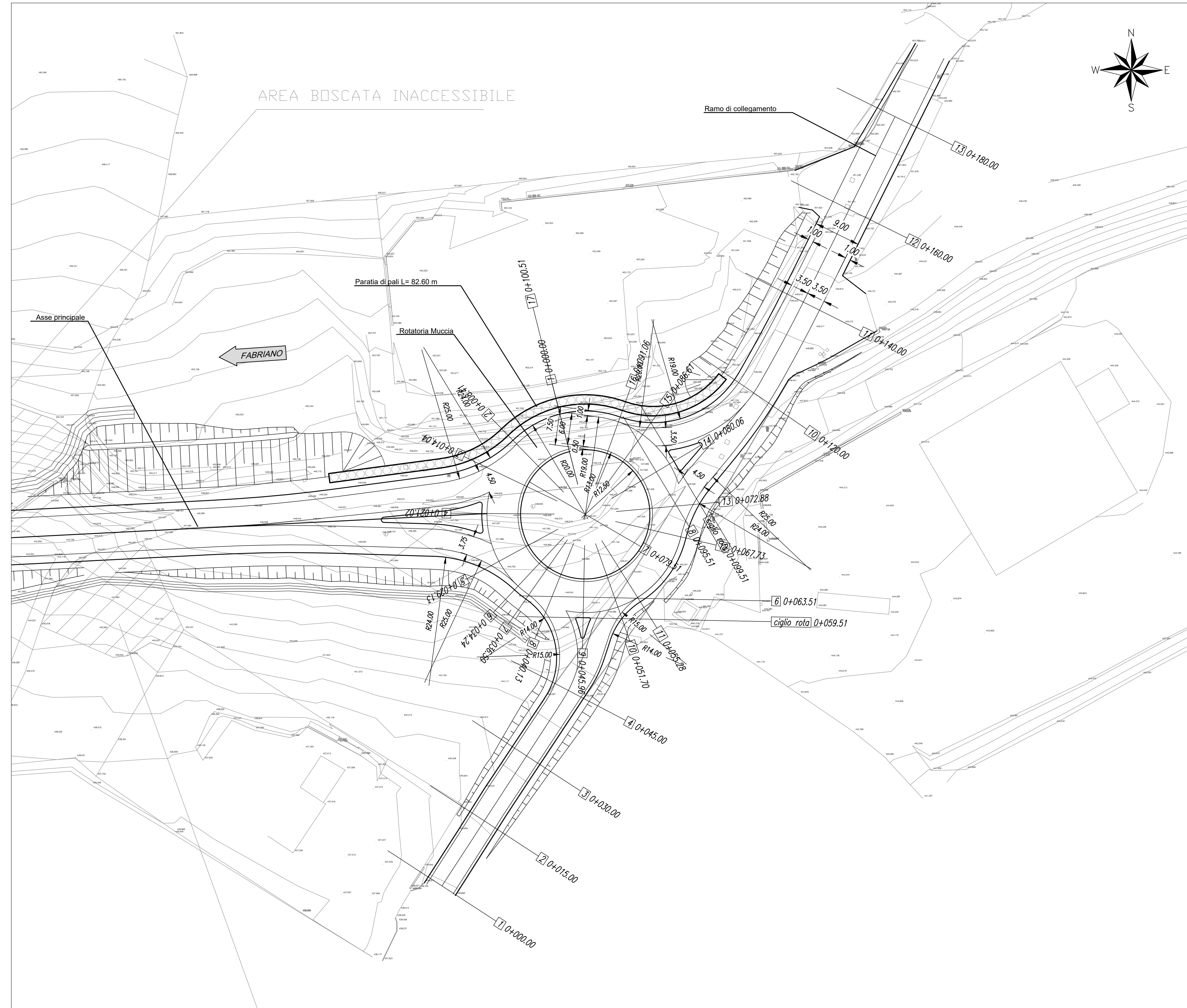
Planimetria di progetto - Scala - 1:500
