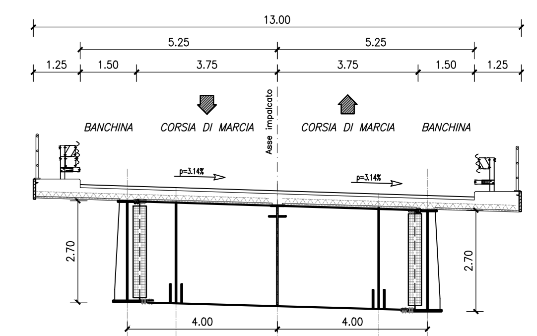
SEZIONE TRASVERSALE CORRENTE – Scala 1:100
