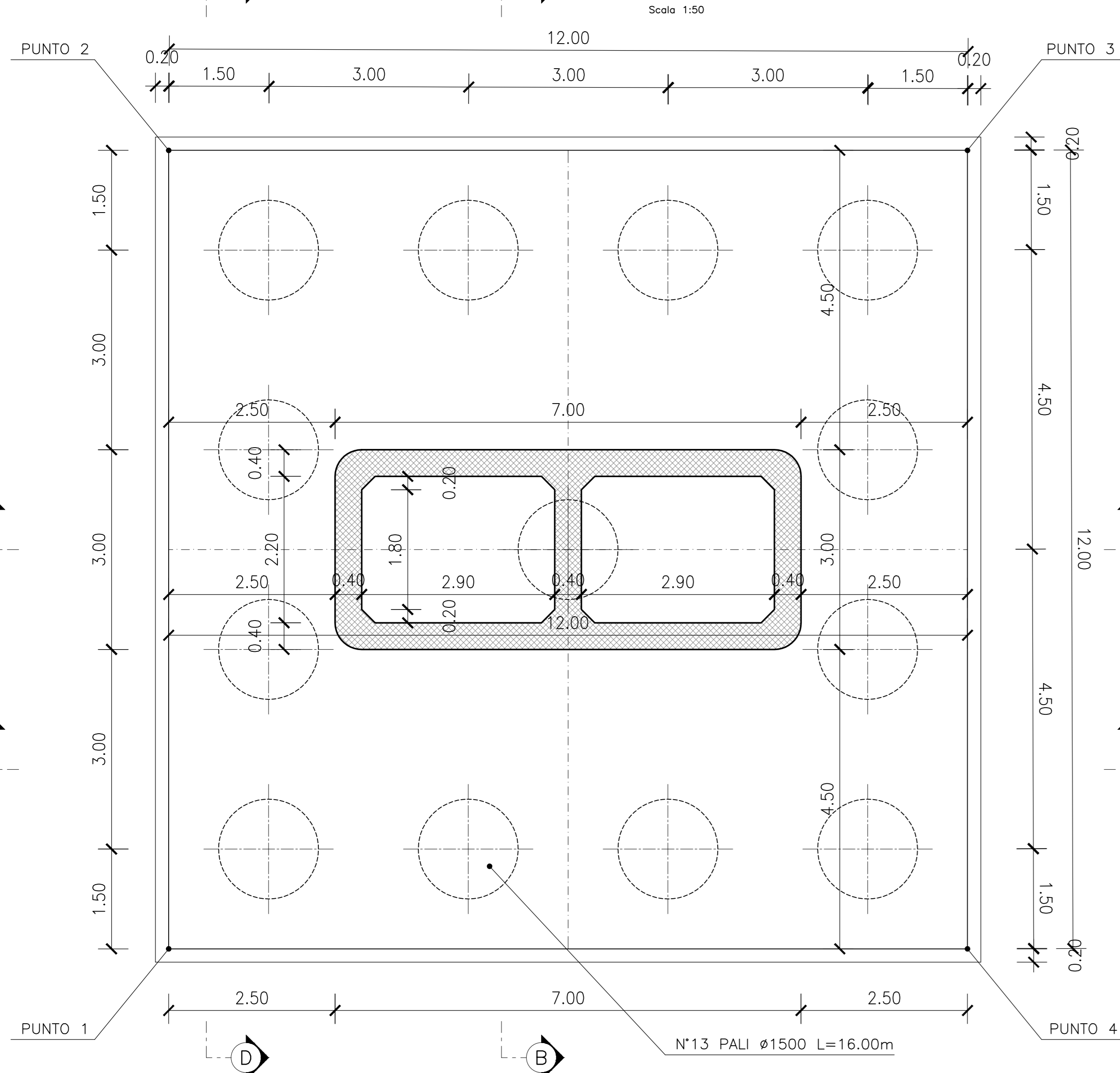
PIANTA FONDAZIONE Scala 1:50
