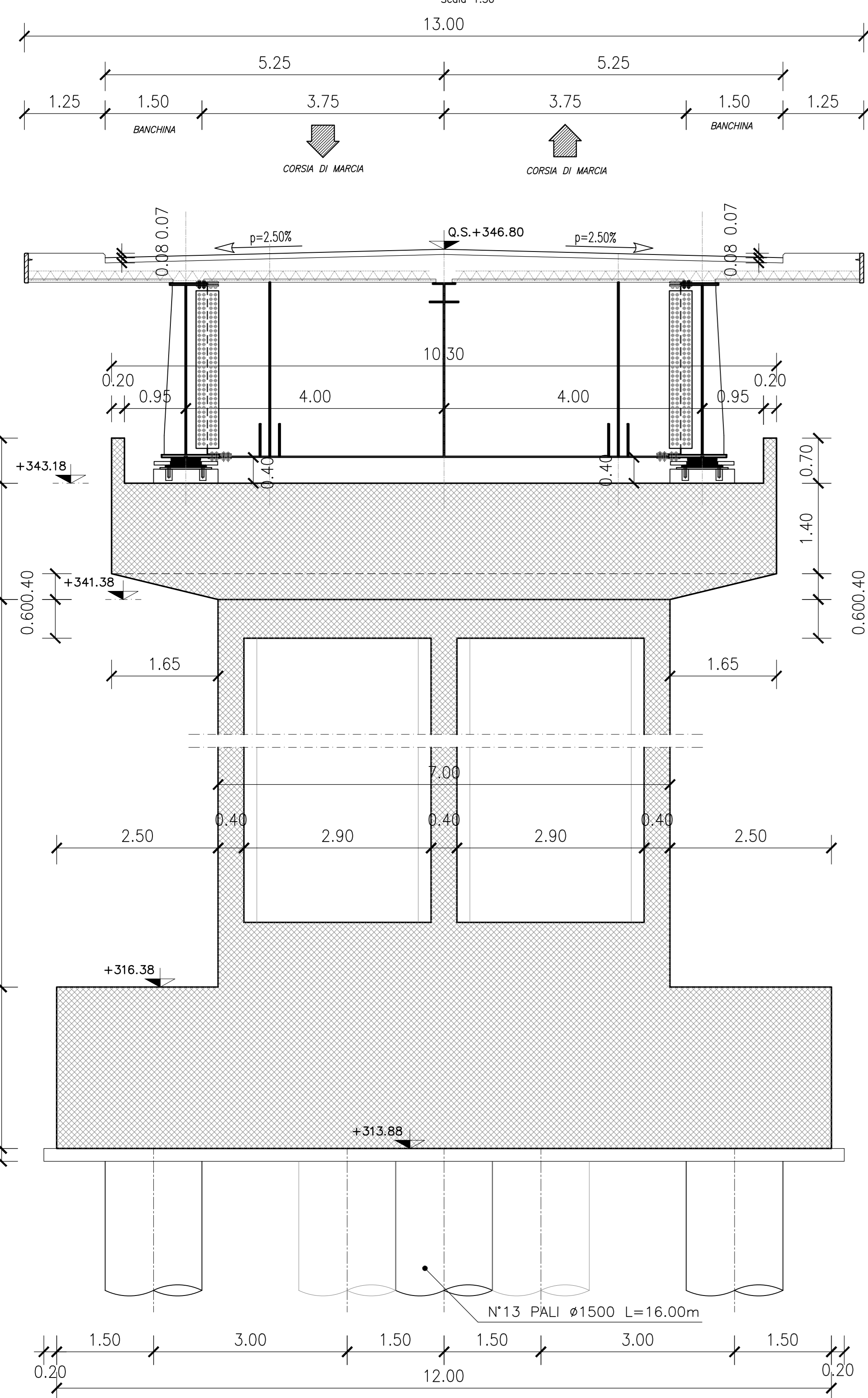
SEZIONE A-A Scala 1:50
