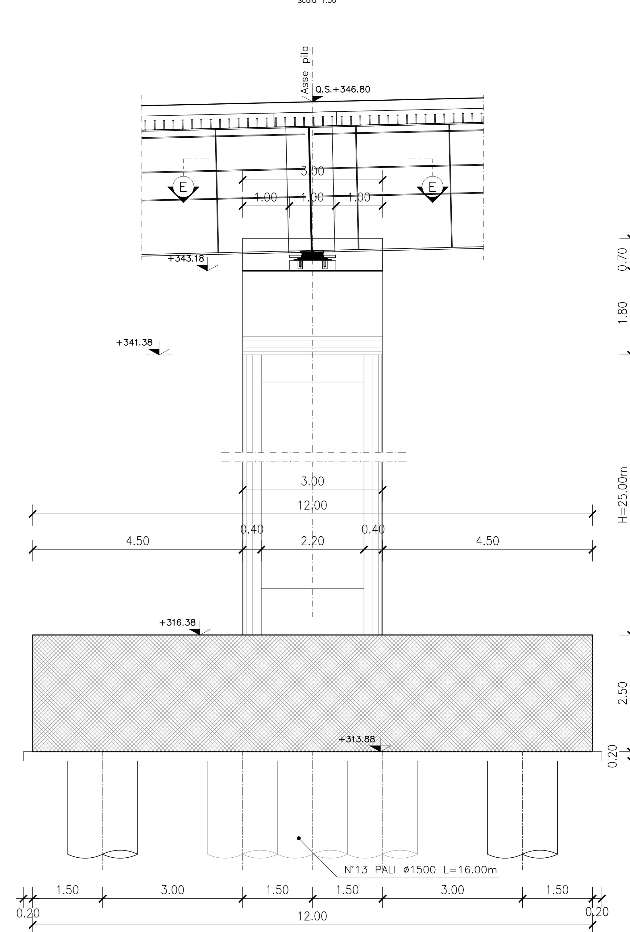
SEZIONE D-D Scala 1:50
