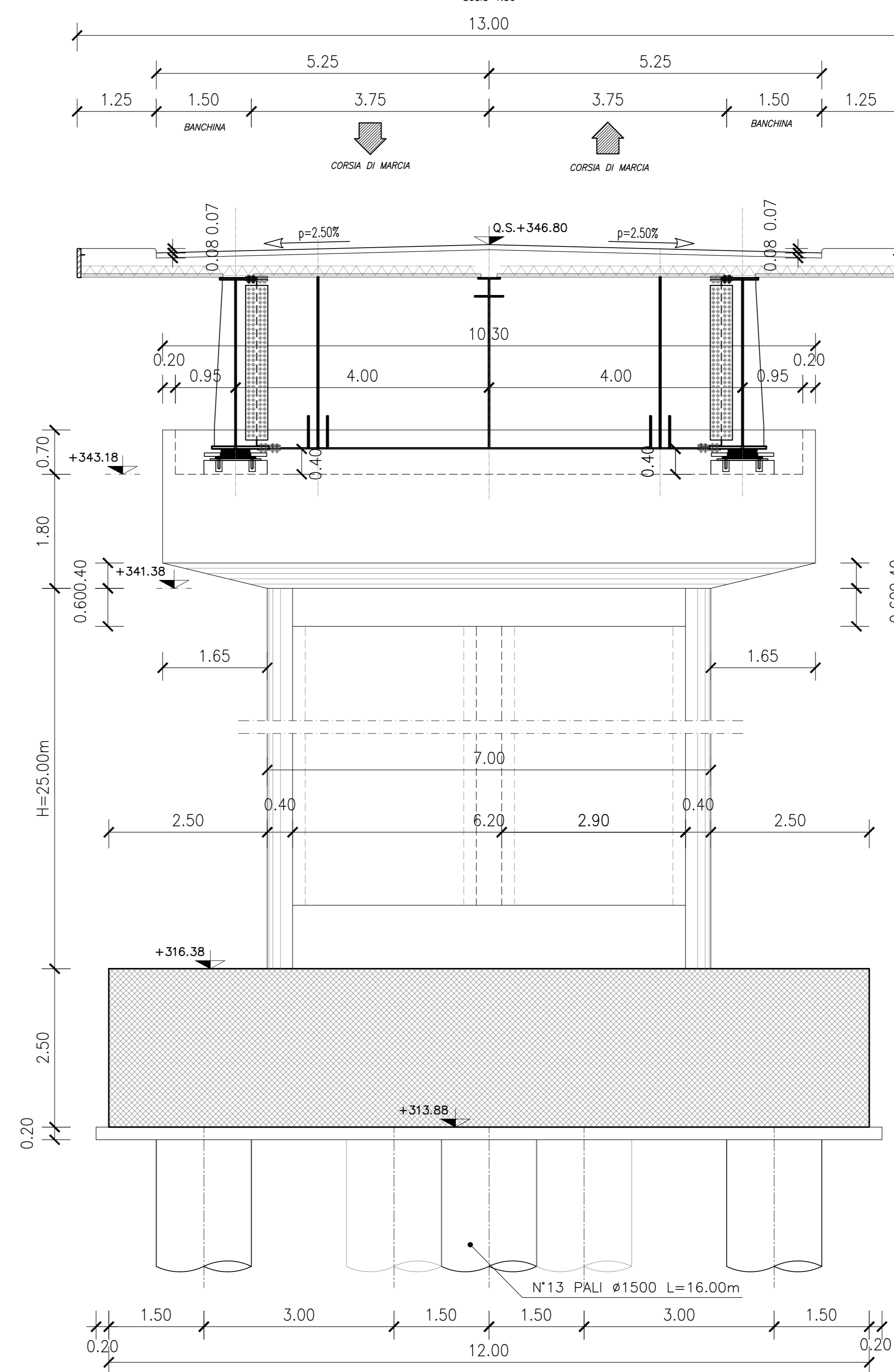
SEZIONE C-C Scala 1:50
