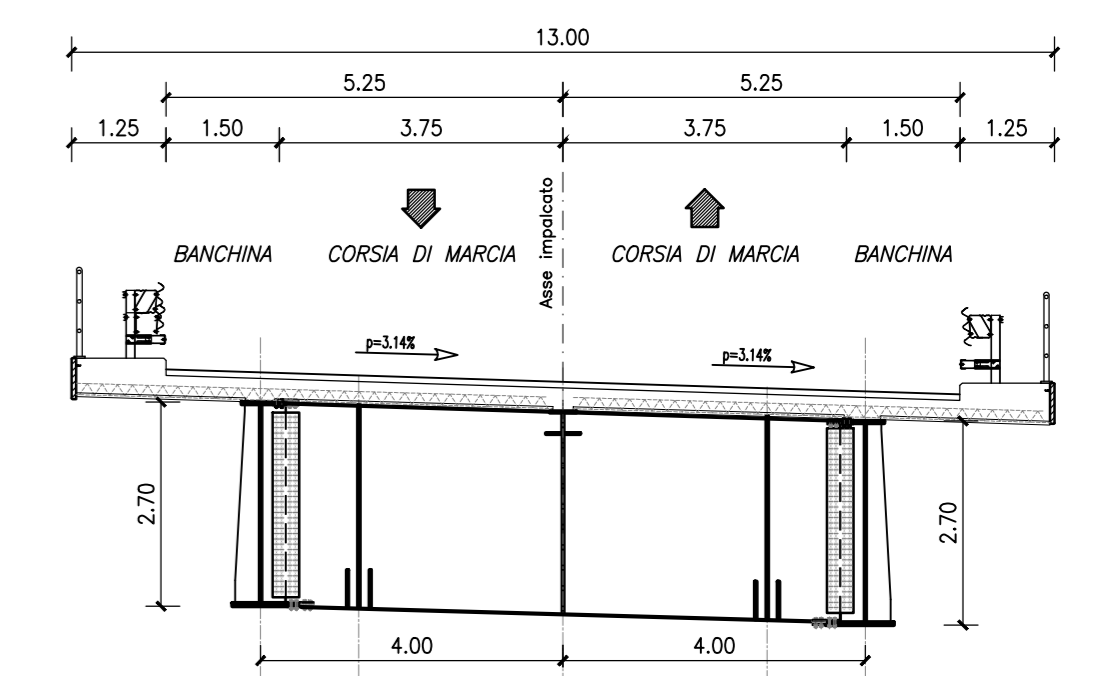
SEZIONE TRASVERSALE CORRENTE – Scala 1:100
