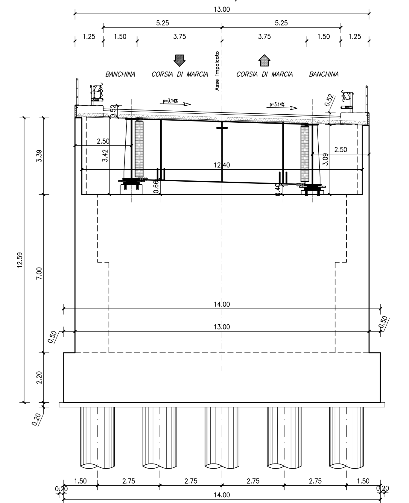
SEZIONE TRASVERSALE CORRENTE – Scala 1:100
